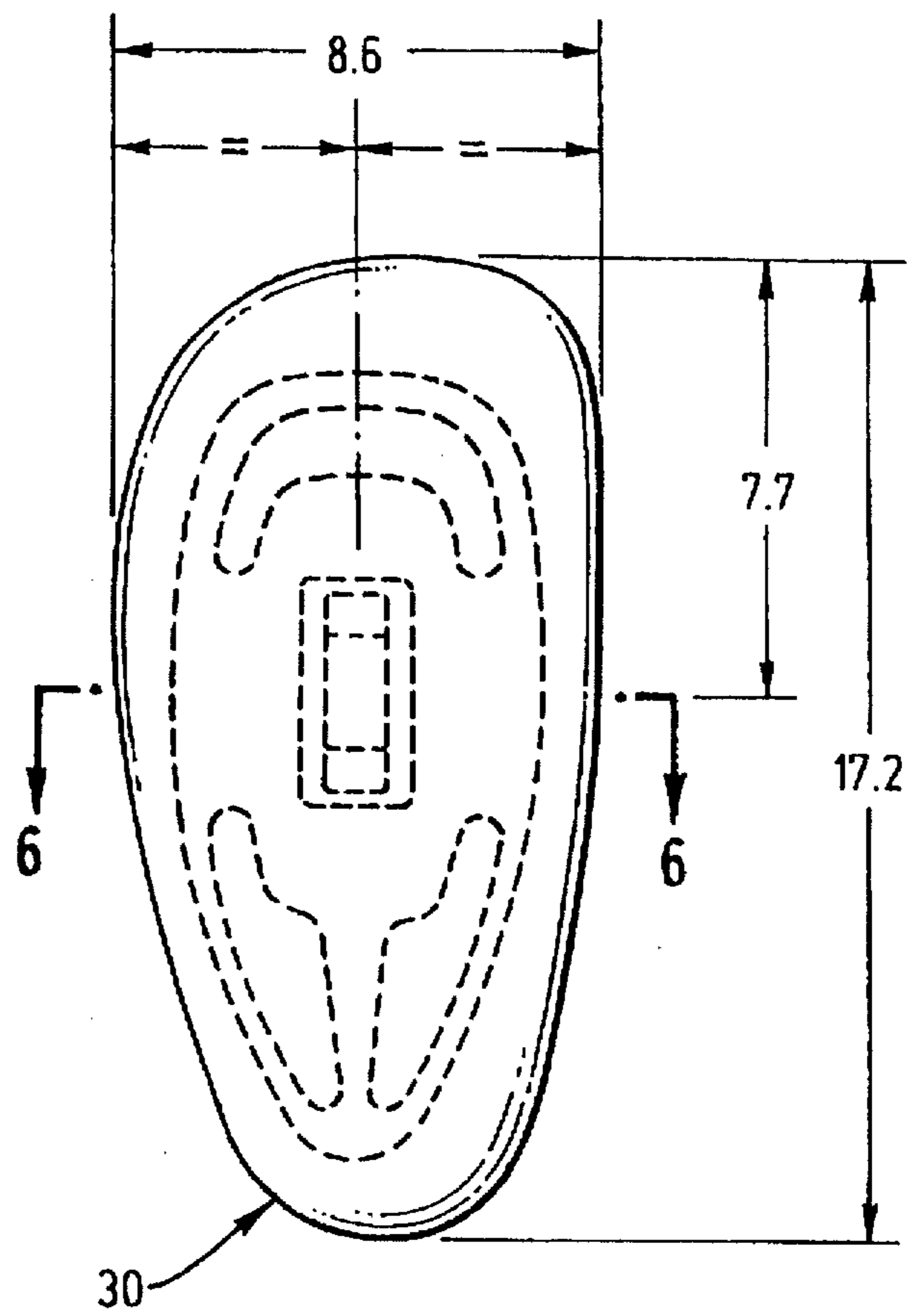
FIG. 5
