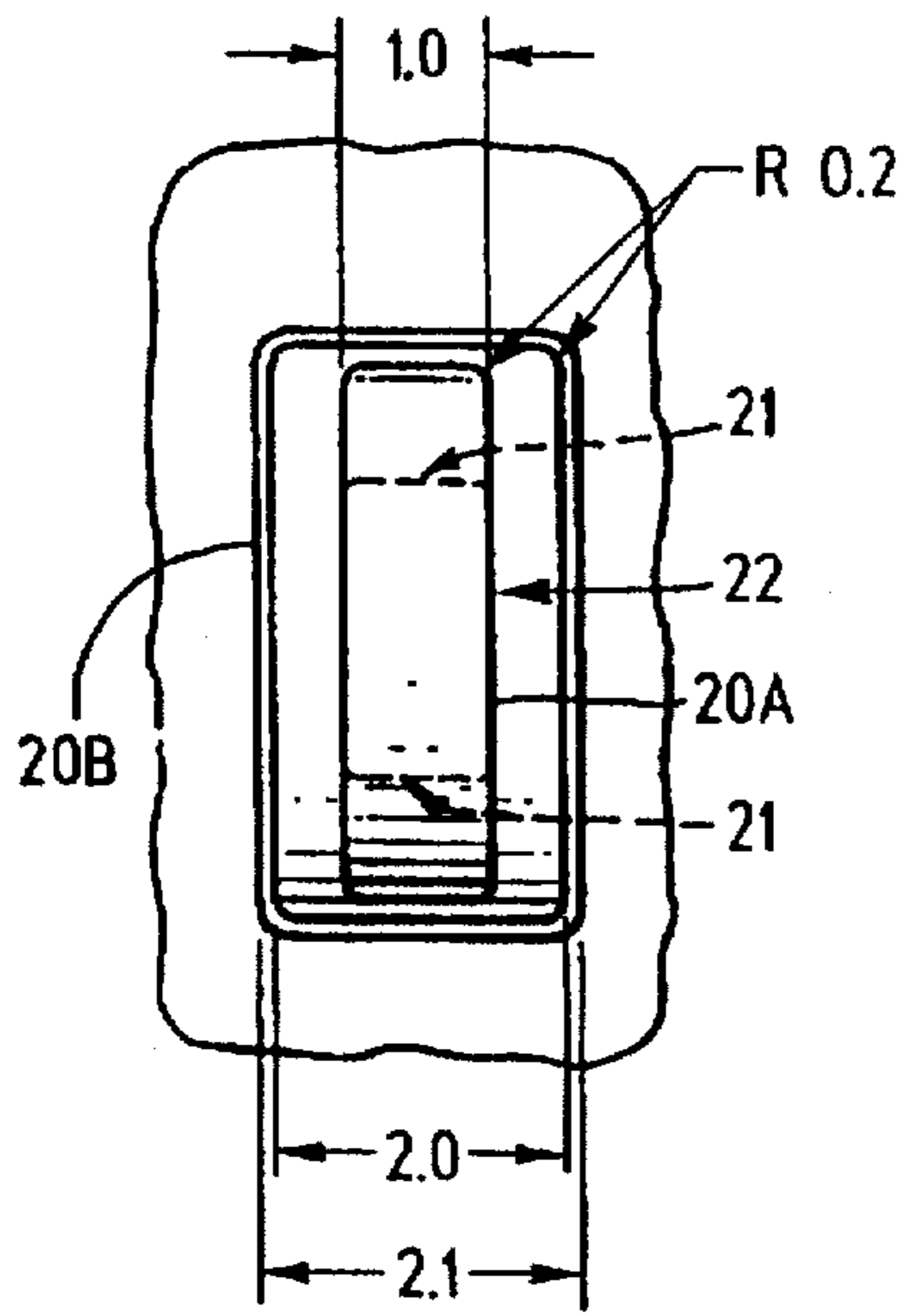
FIG. 7
