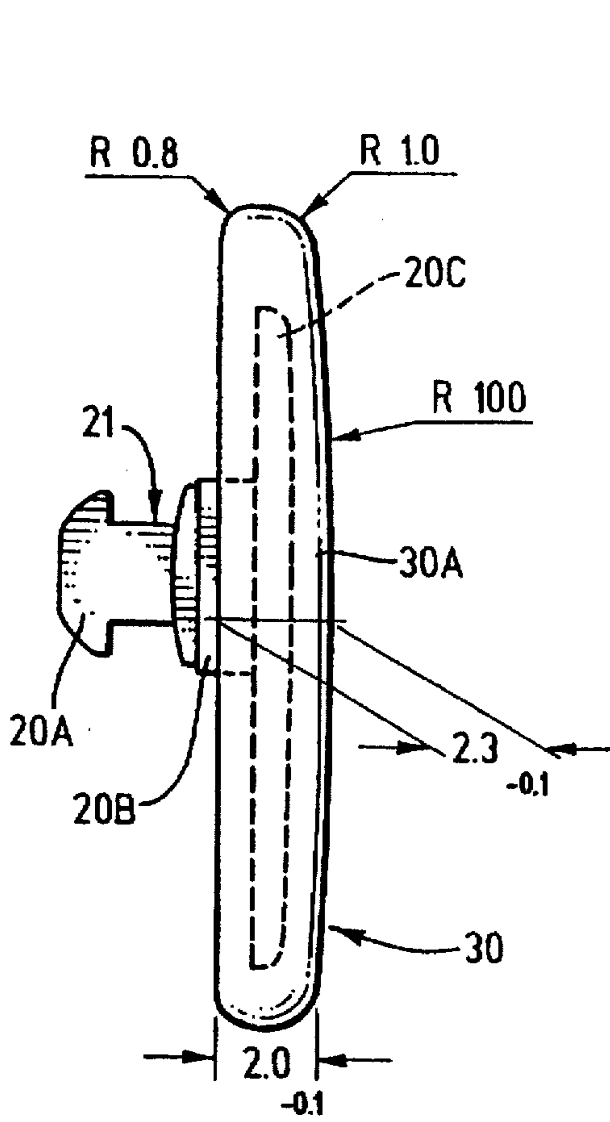
FIG. 4
