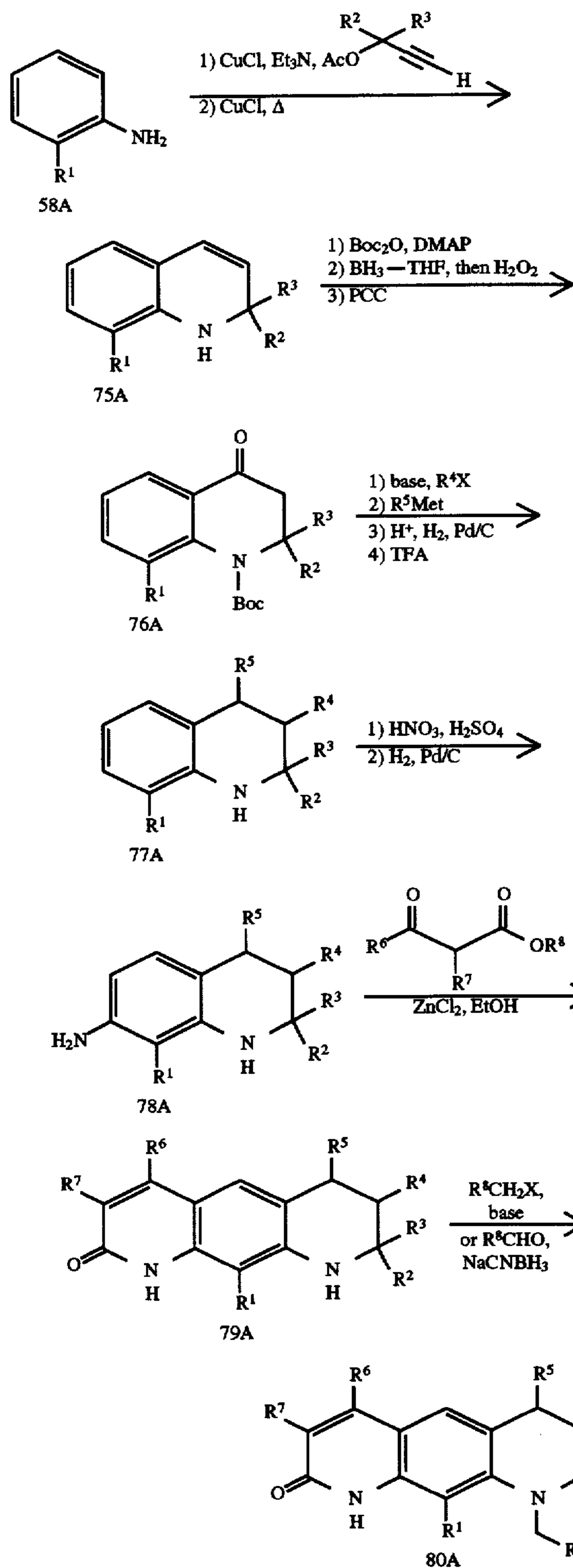
Scheme LIII
