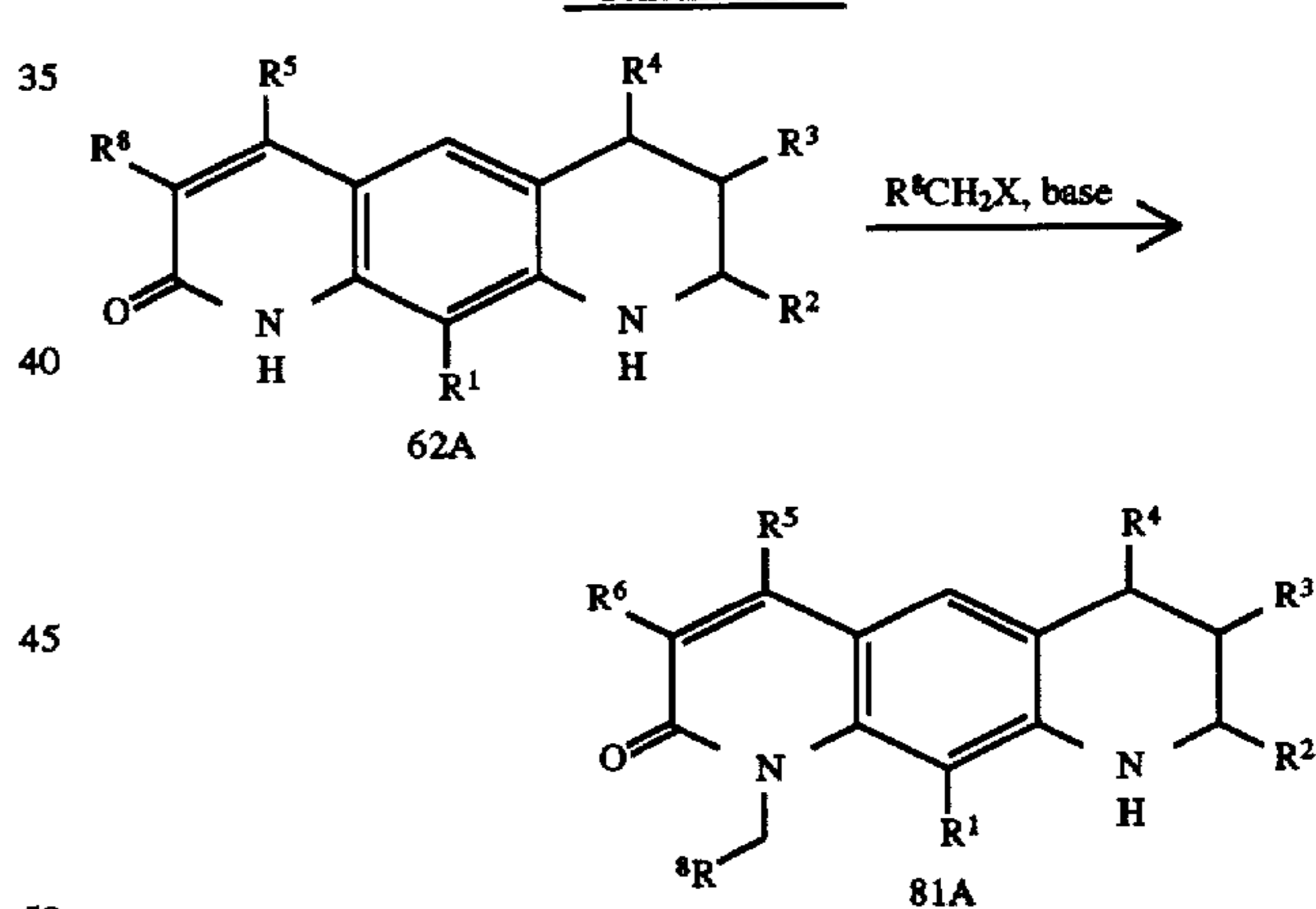
Scheme LIV
