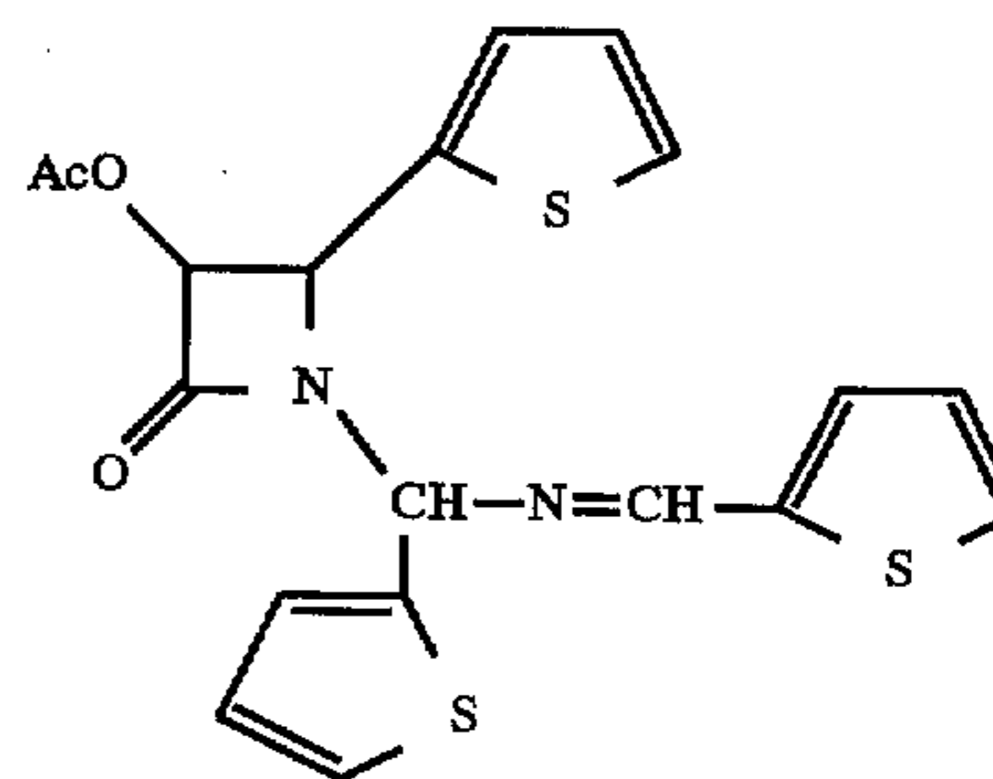
(±)-cis-3-Acetyloxy-1-[(2-thienyl) (2-thienylmethylenimino)methyl]-4-(2-thienyl)azetid-2-one (XIVc)
