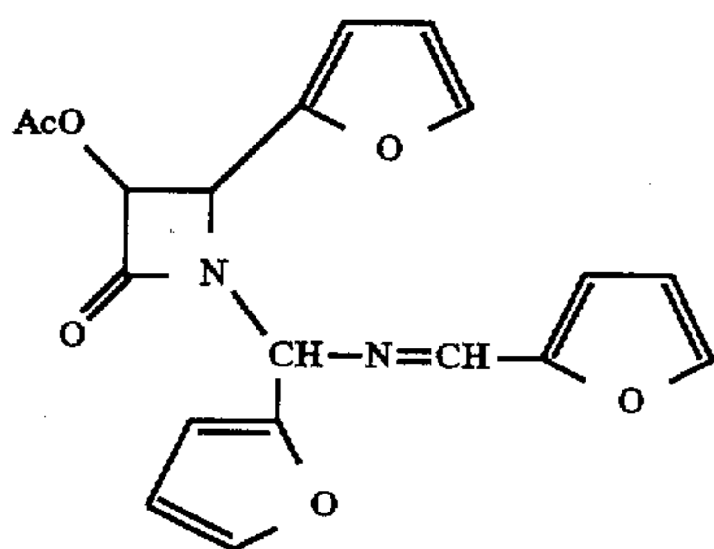
(±)-cis-3-Acetyloxy-1-[(2-furyl) (2-furylmethylenimino)methyl]-4-(2-furyl)azetid-2-one (XIVb)
