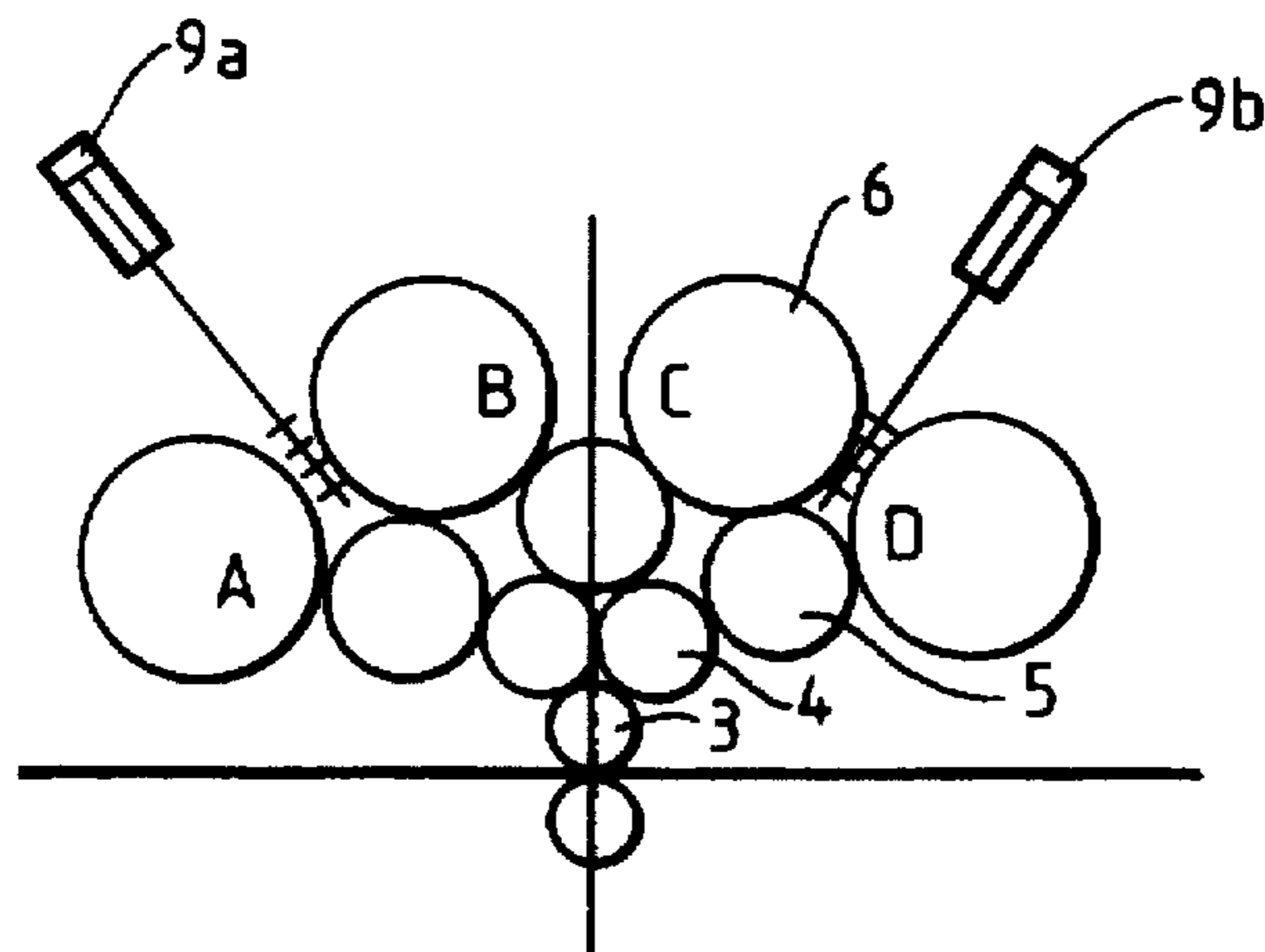
FIG. 12
