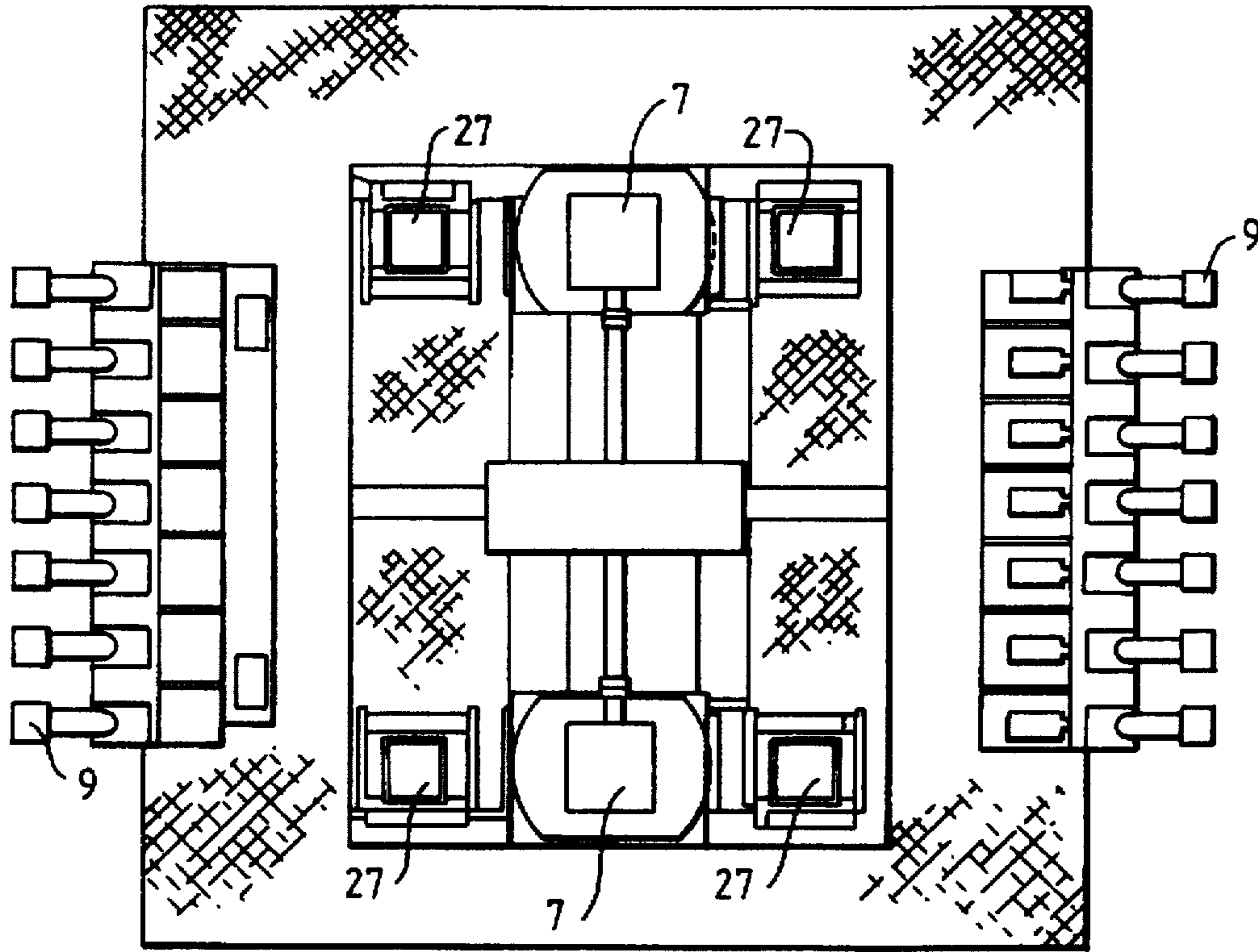
FIG. 16
