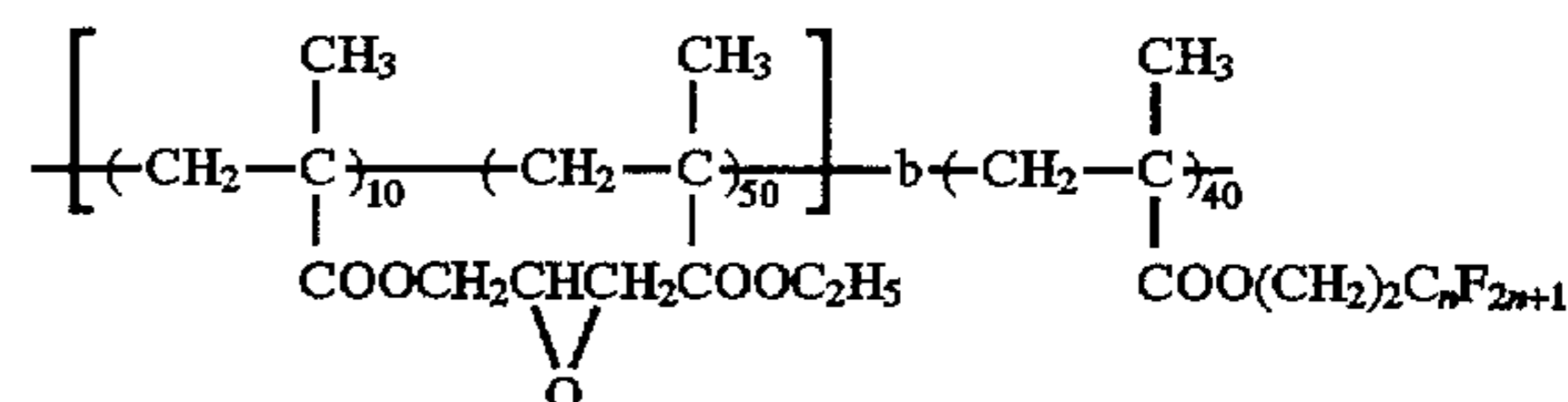
Resin (P-14)
