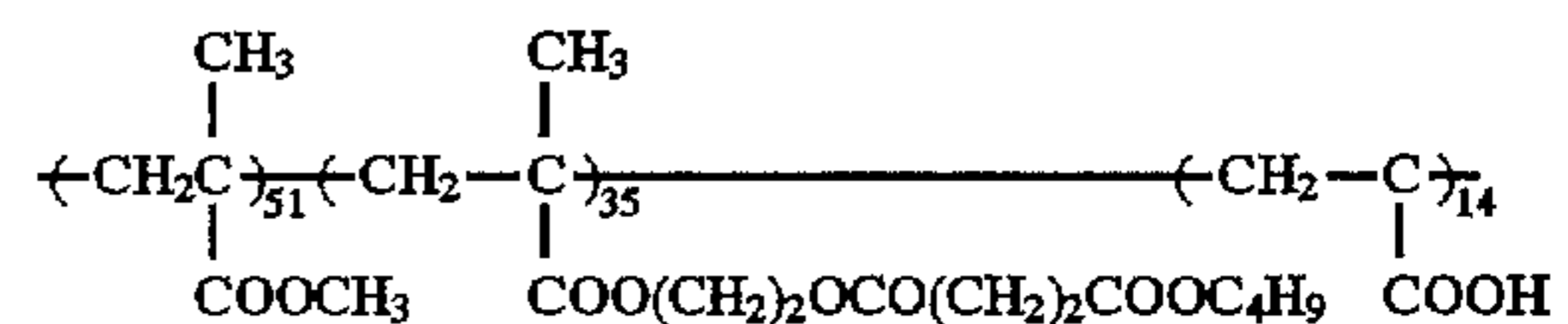
Resin (A-4)
