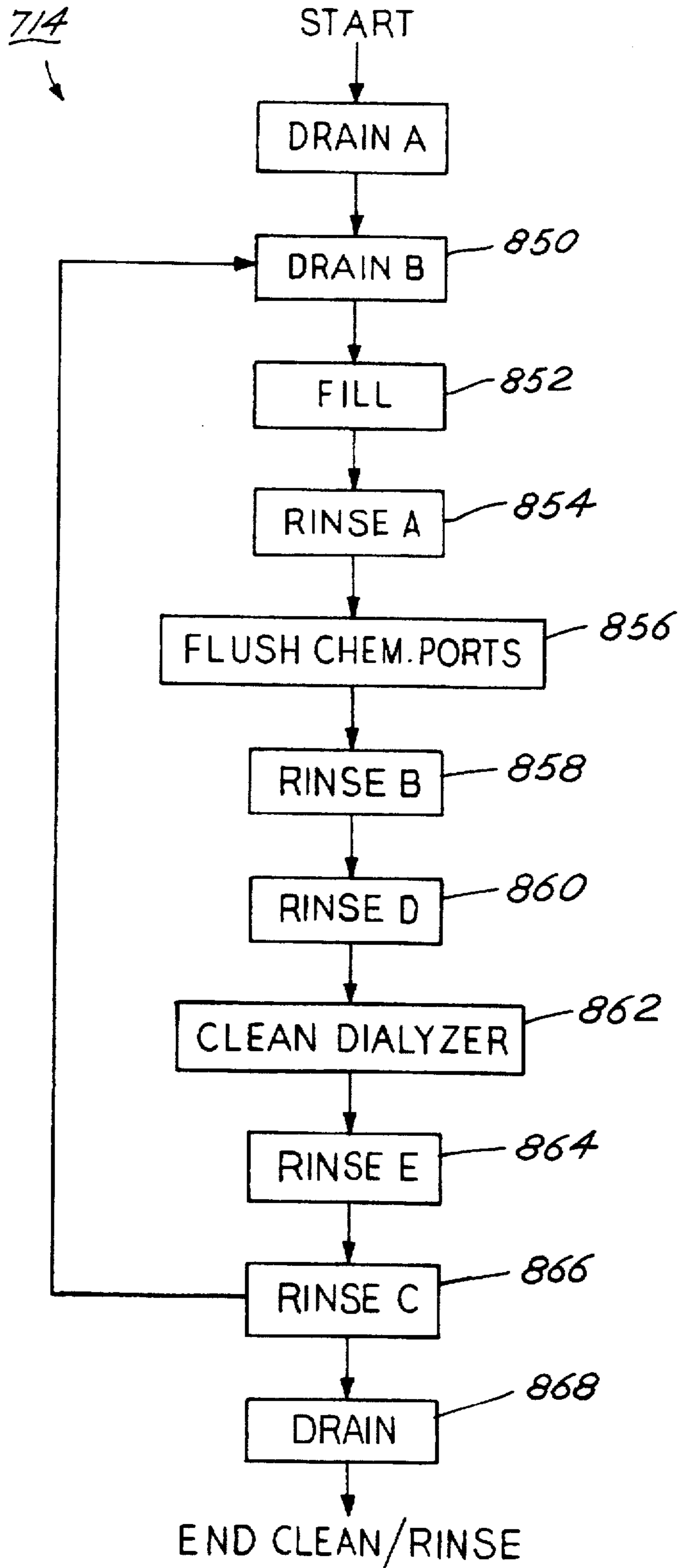
FIG. 23 CLEAN/RINSE
