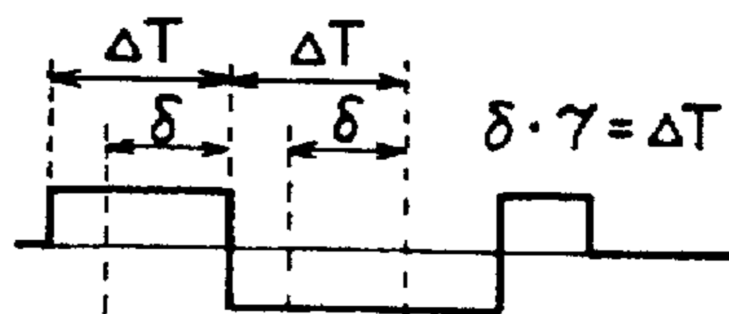
FIG. 26B-1 DATA SIGNAL I (-0%)
