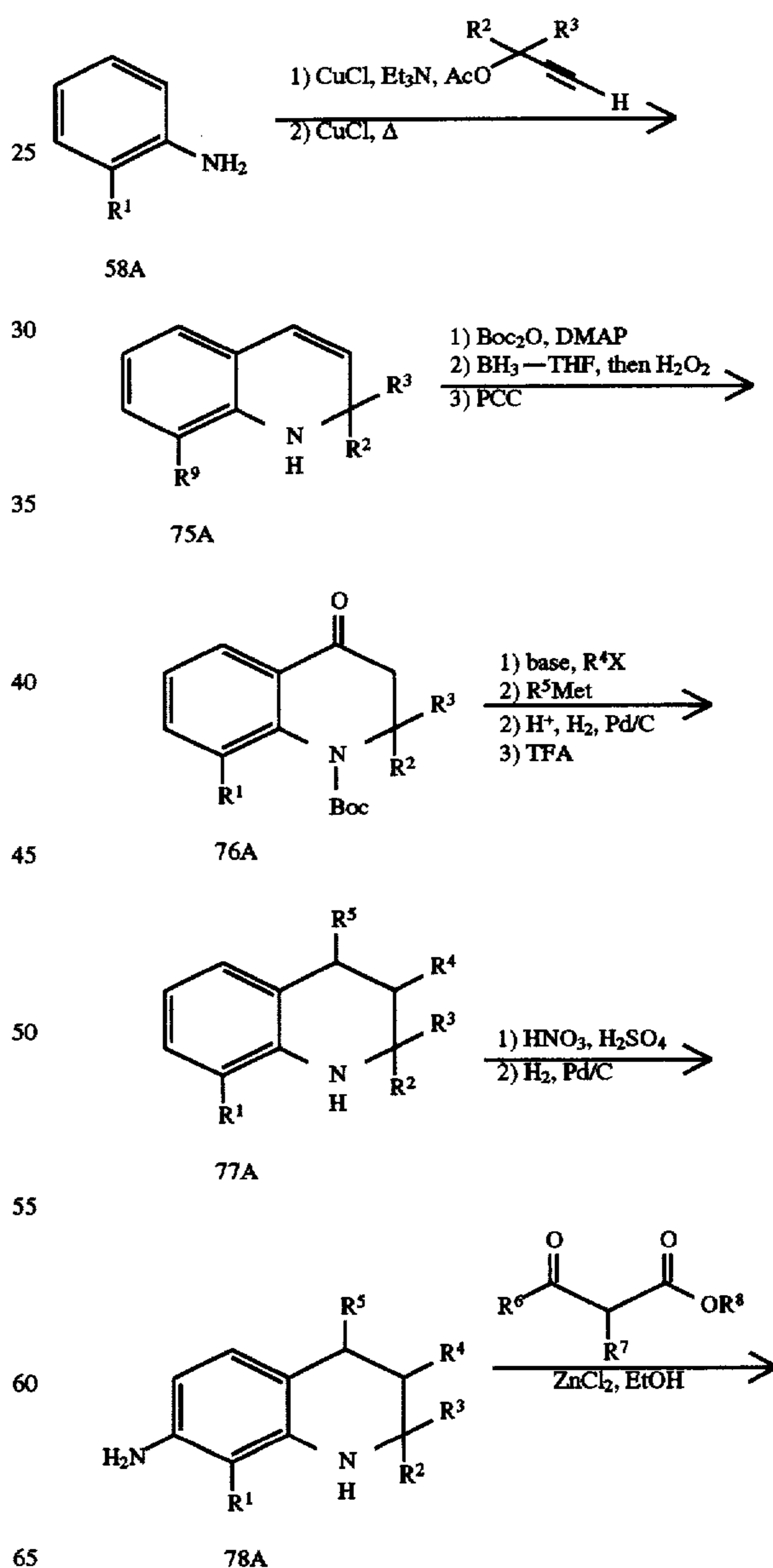
Scheme LIII
