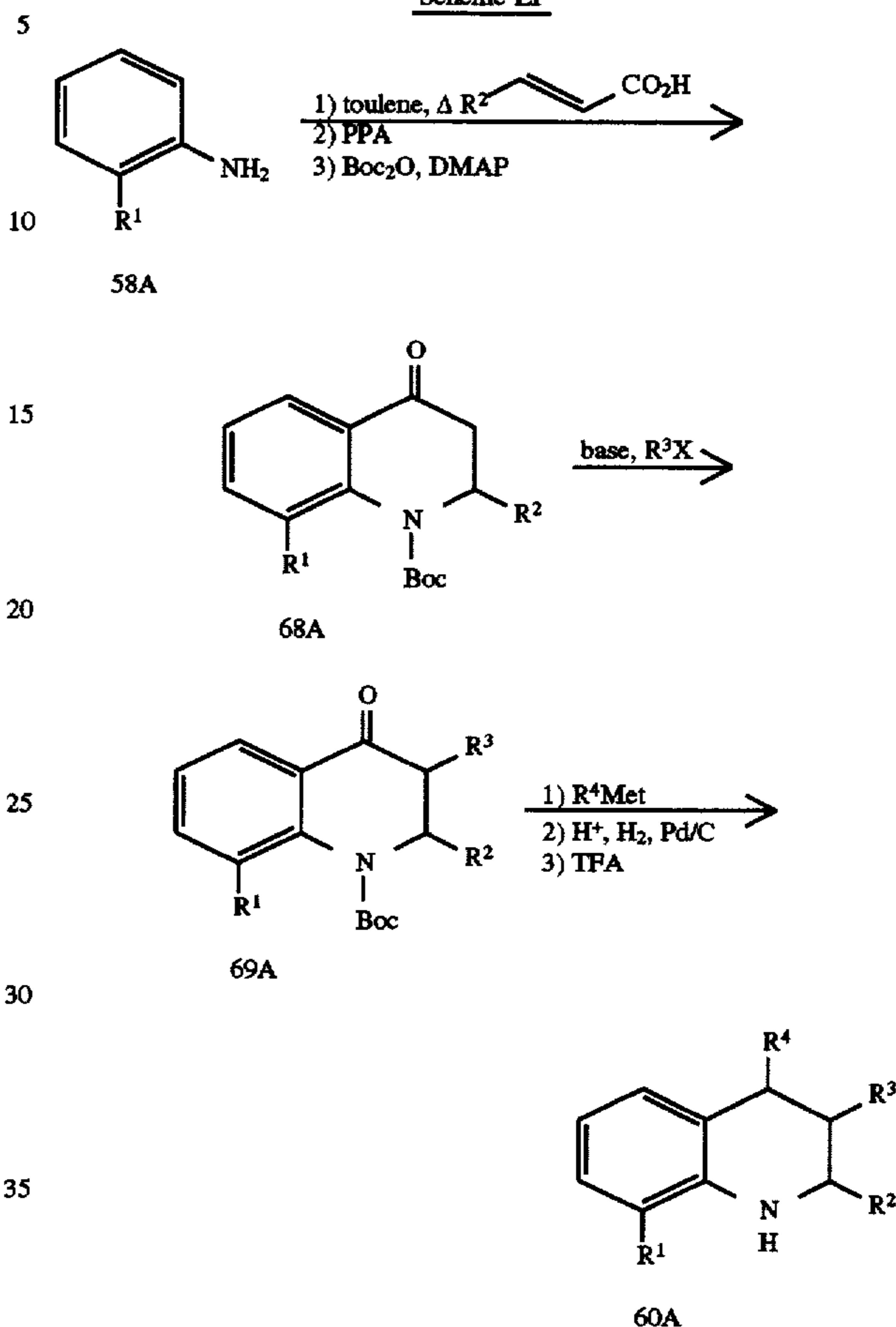
Scheme LI
