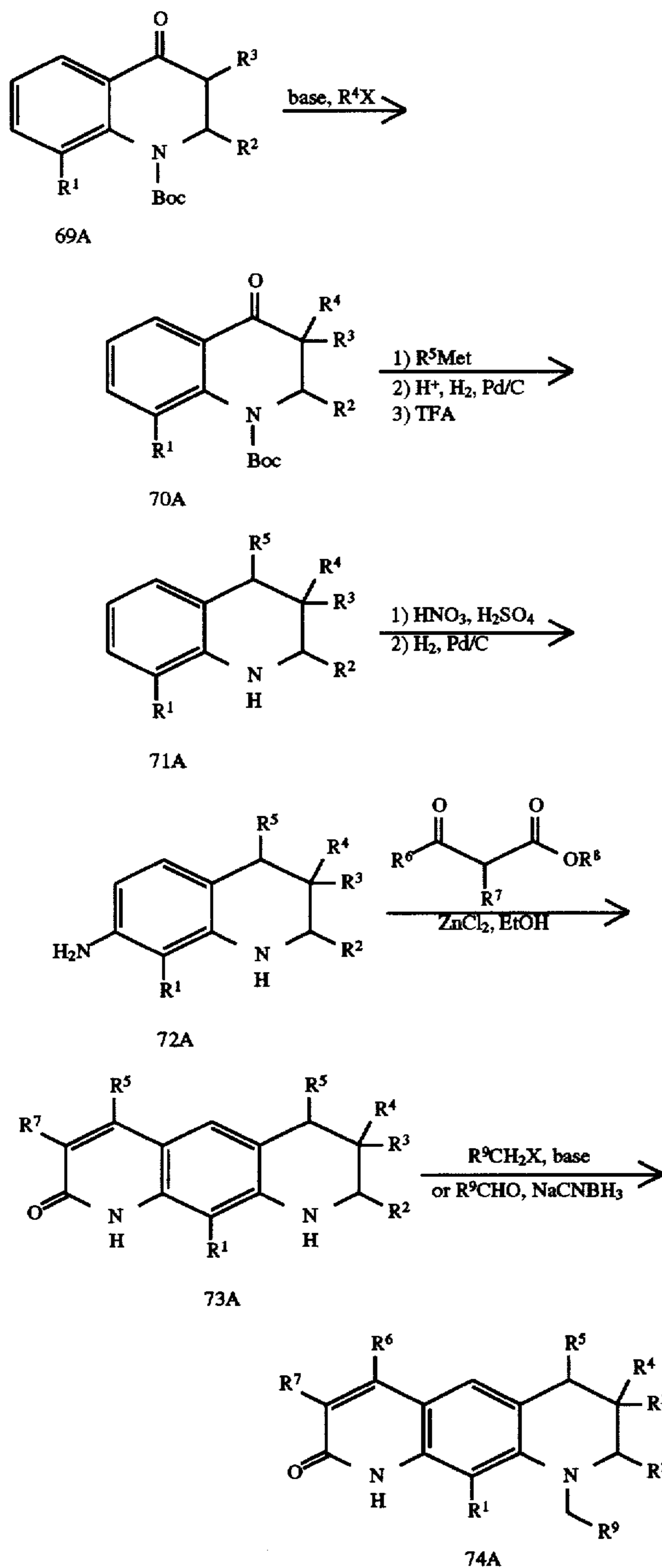
Scheme LII
