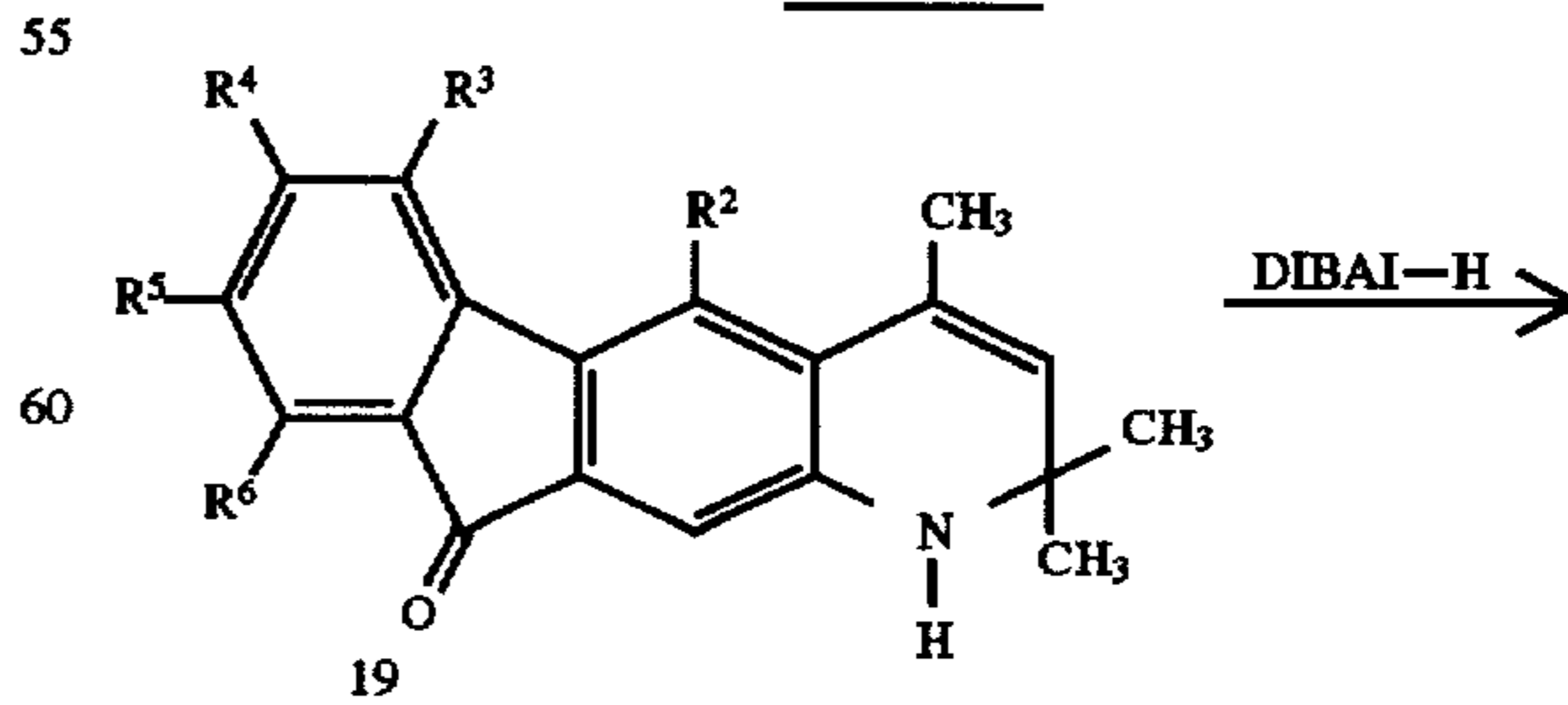
Scheme VI
