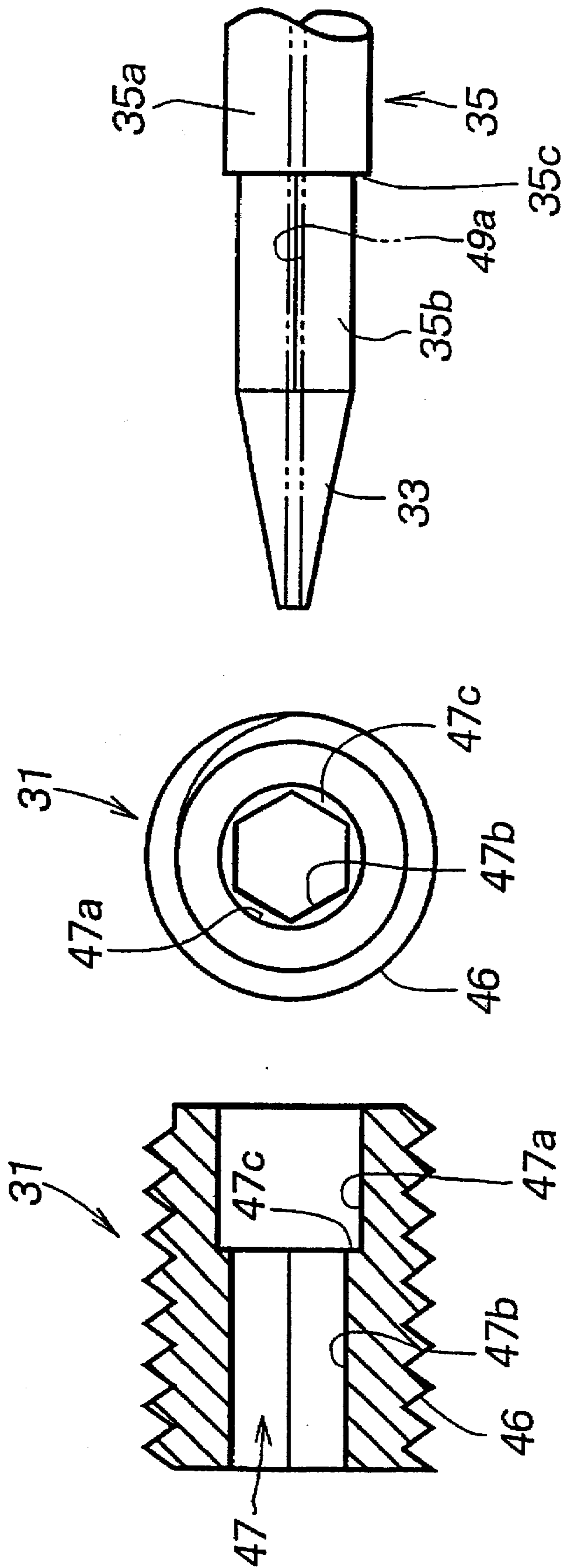
FIG. 11C
