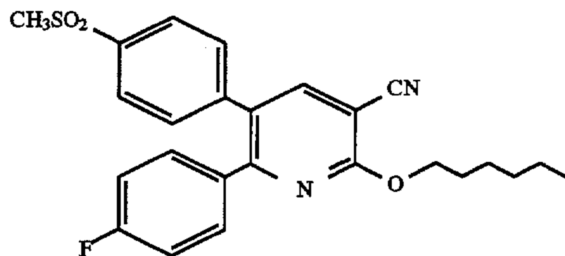
6-(4-Fluorophenyl)-2-hexyloxy-5-[4-(methylsulfonyl)phenyl]pyridine-3-carbonitrile
