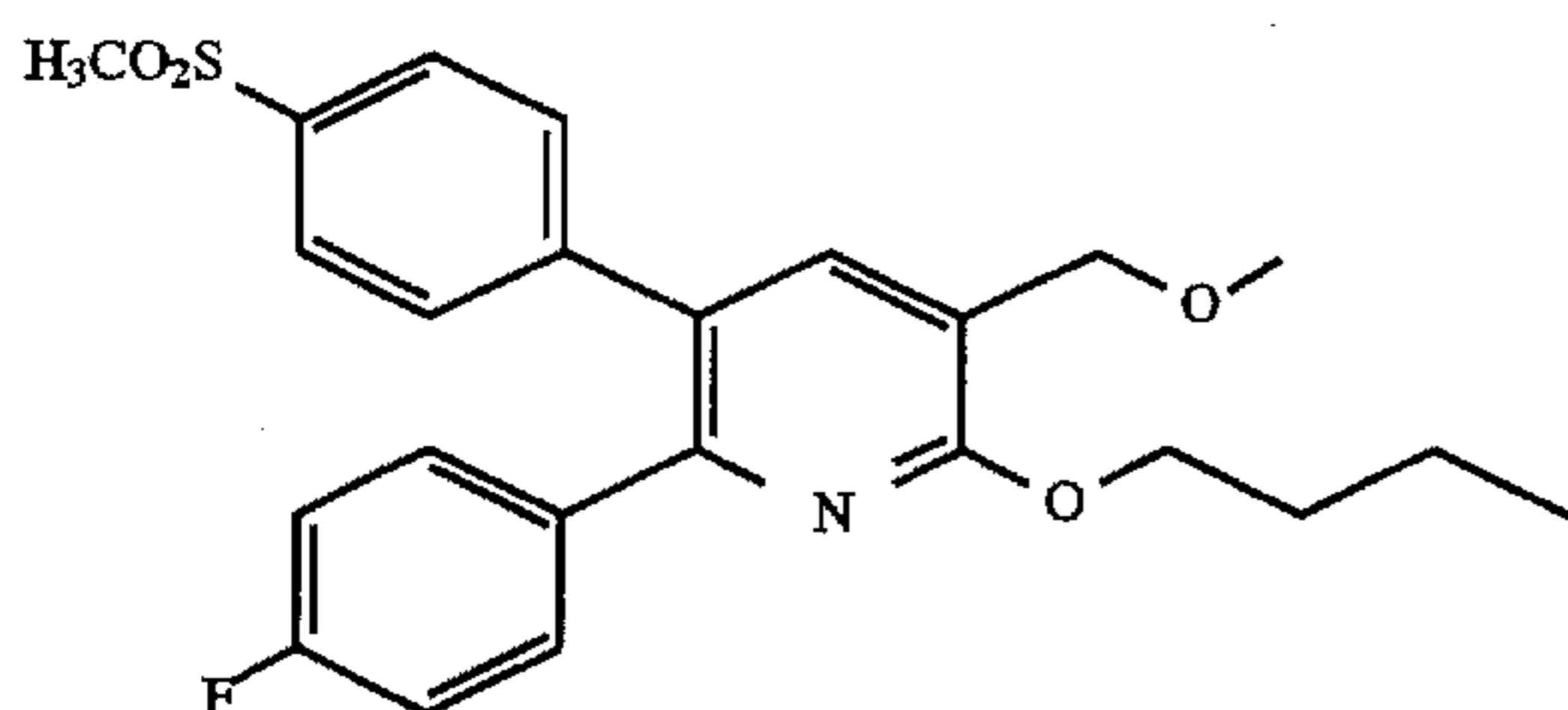
2-Butoxy-6-(4-fluorophenyl)-3-(methoxymethyl)-5-[4-(methylsulfonyl)phenyl]pyridine
