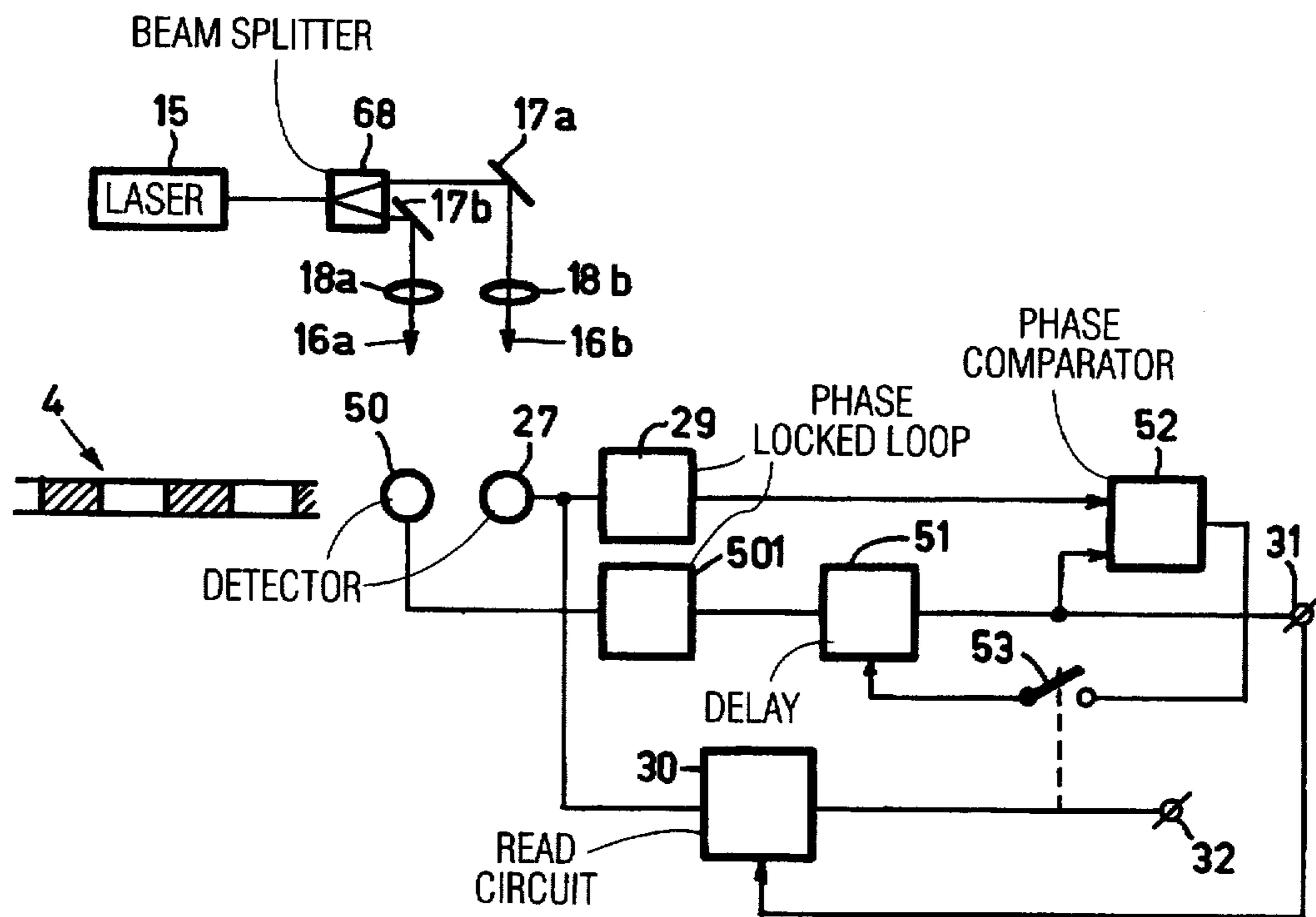
FIG. 12
