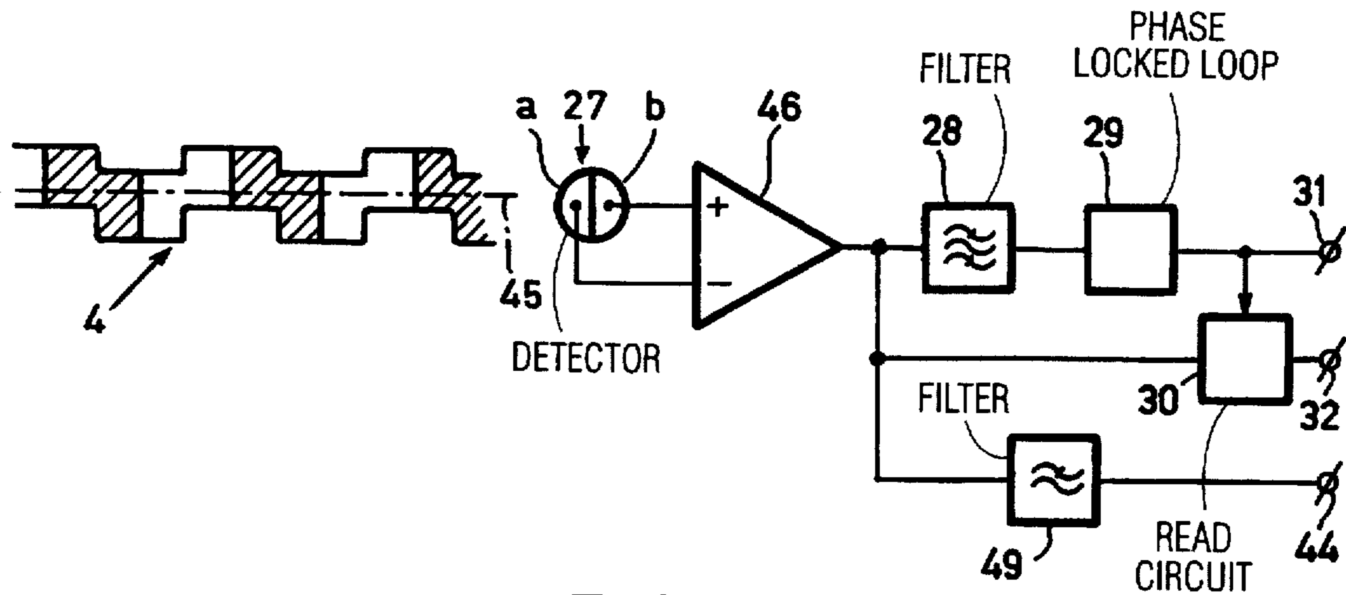
FIG. 12
