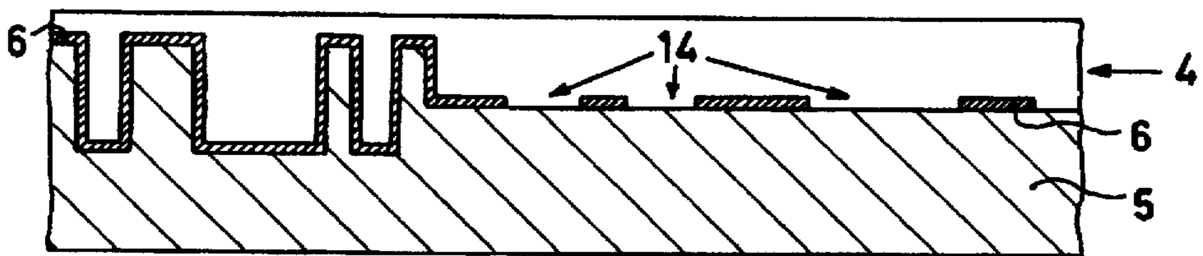
FIG. 3b
