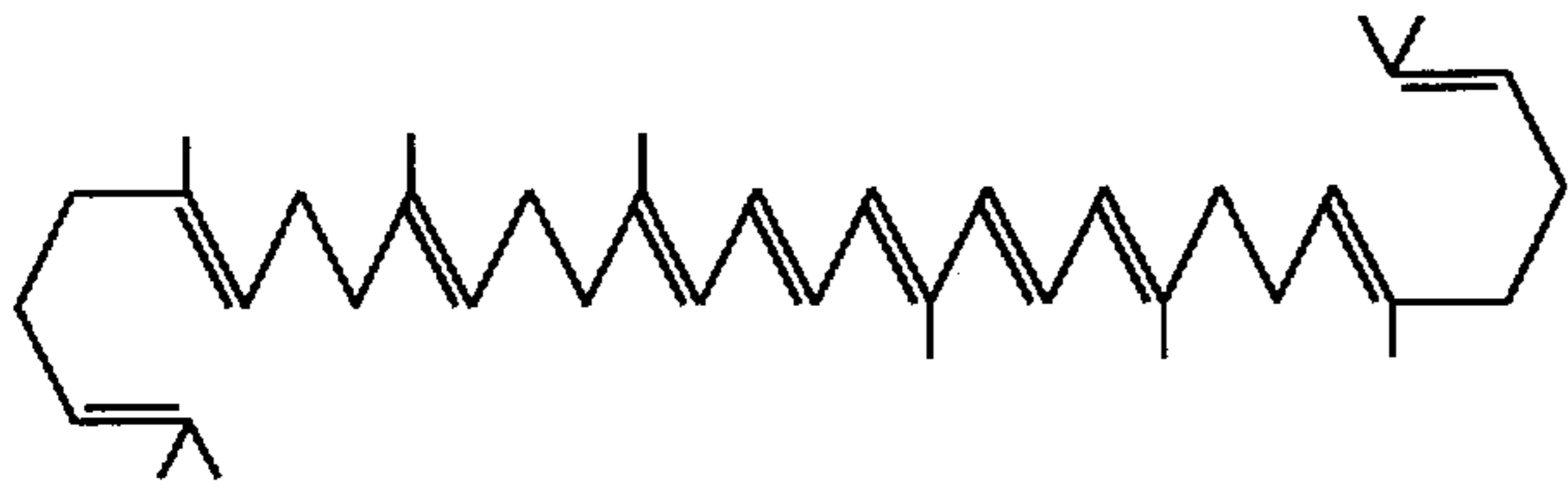
PHYTOFLUENE
