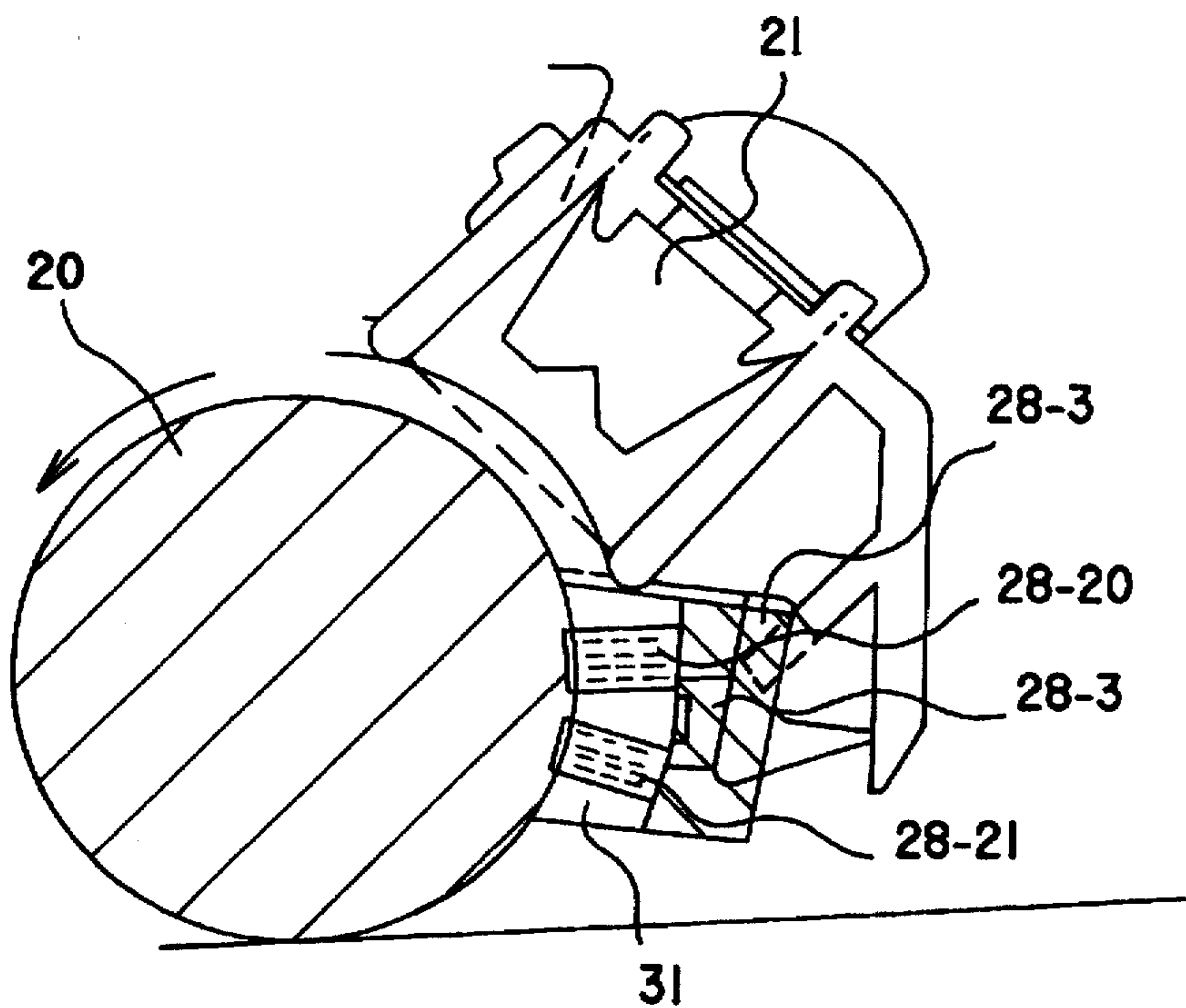
FIG.18A
