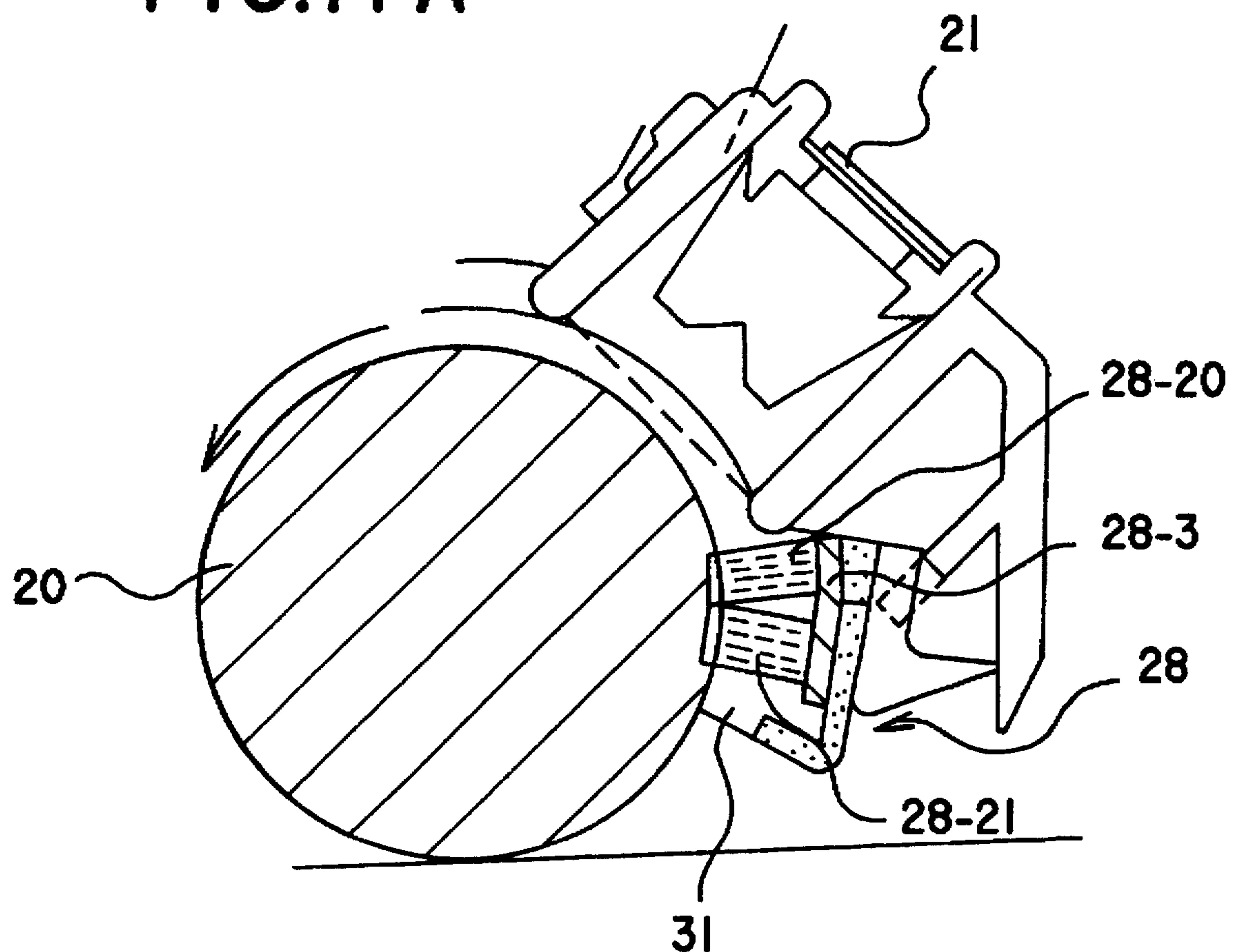
FIG.17A
