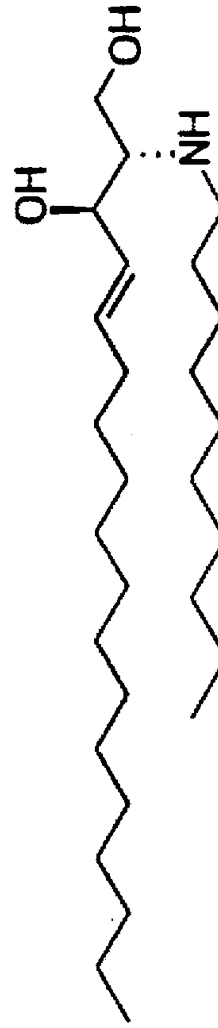
N-C10 Sphingosine
