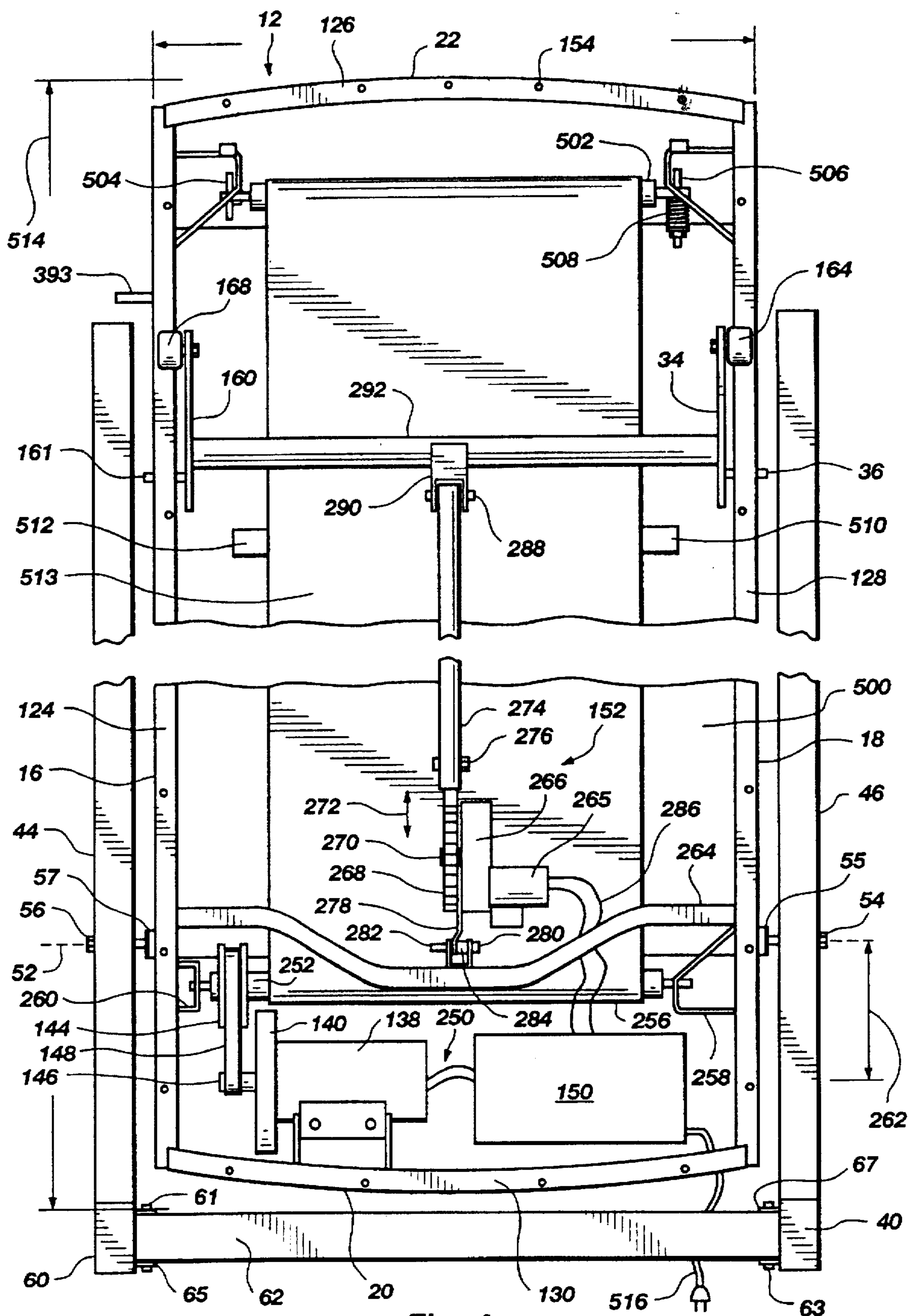
Fig. 4
