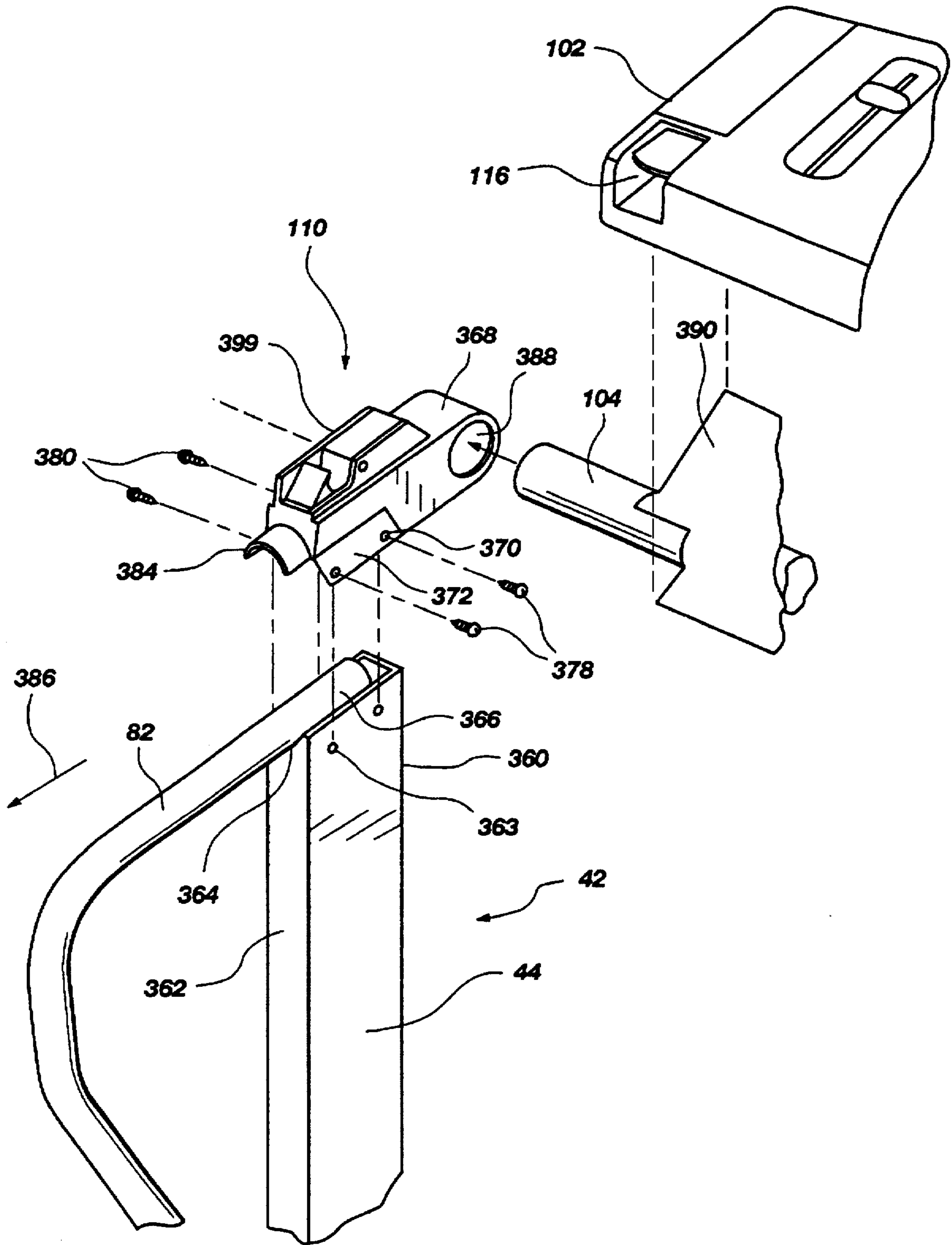
Fig. 8
