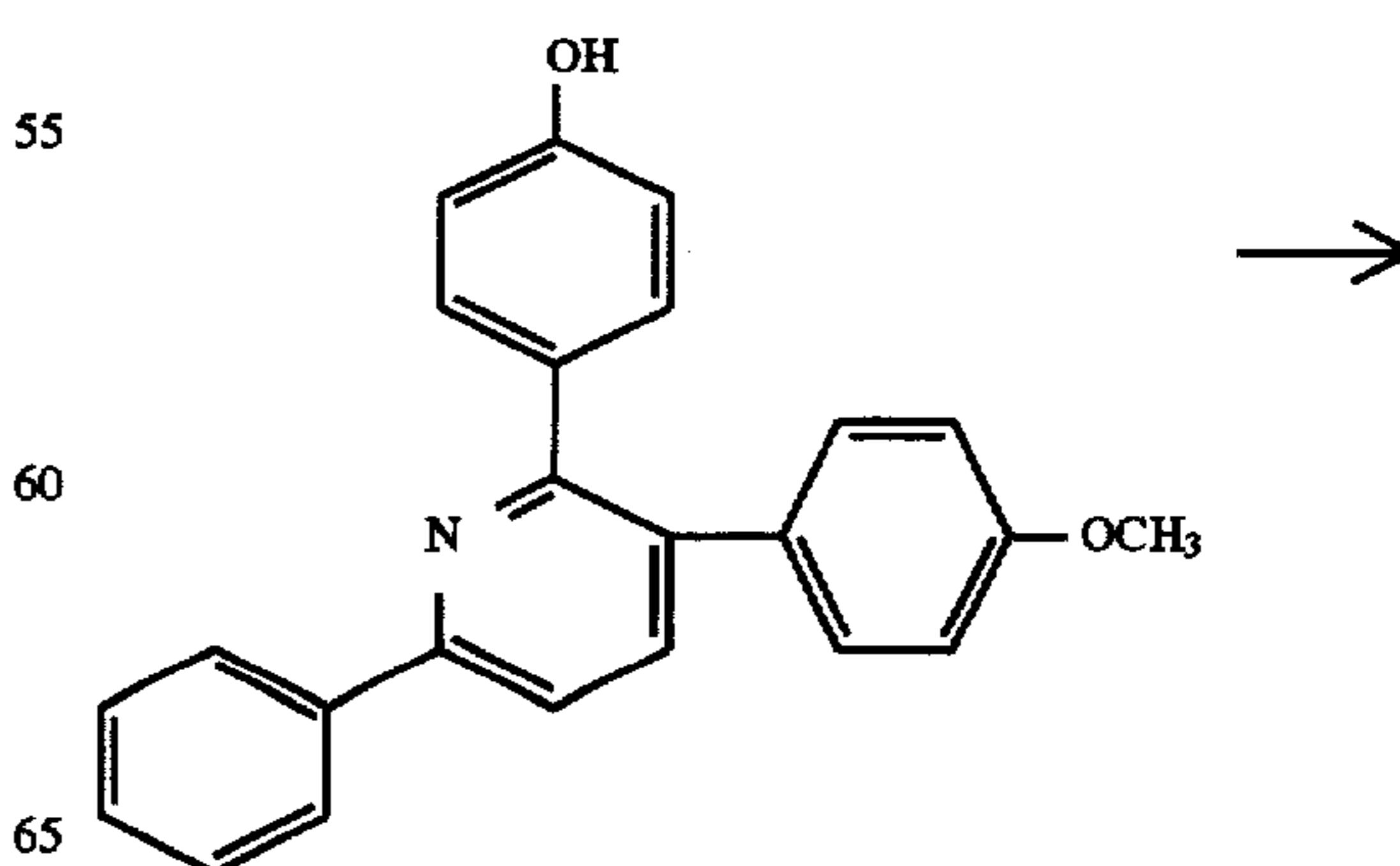
2-[4-[2-(1-Pyrrolidinyl)ethoxy]phenyl]-3-(4-methoxyphenyl)-6-phenylpyridine
