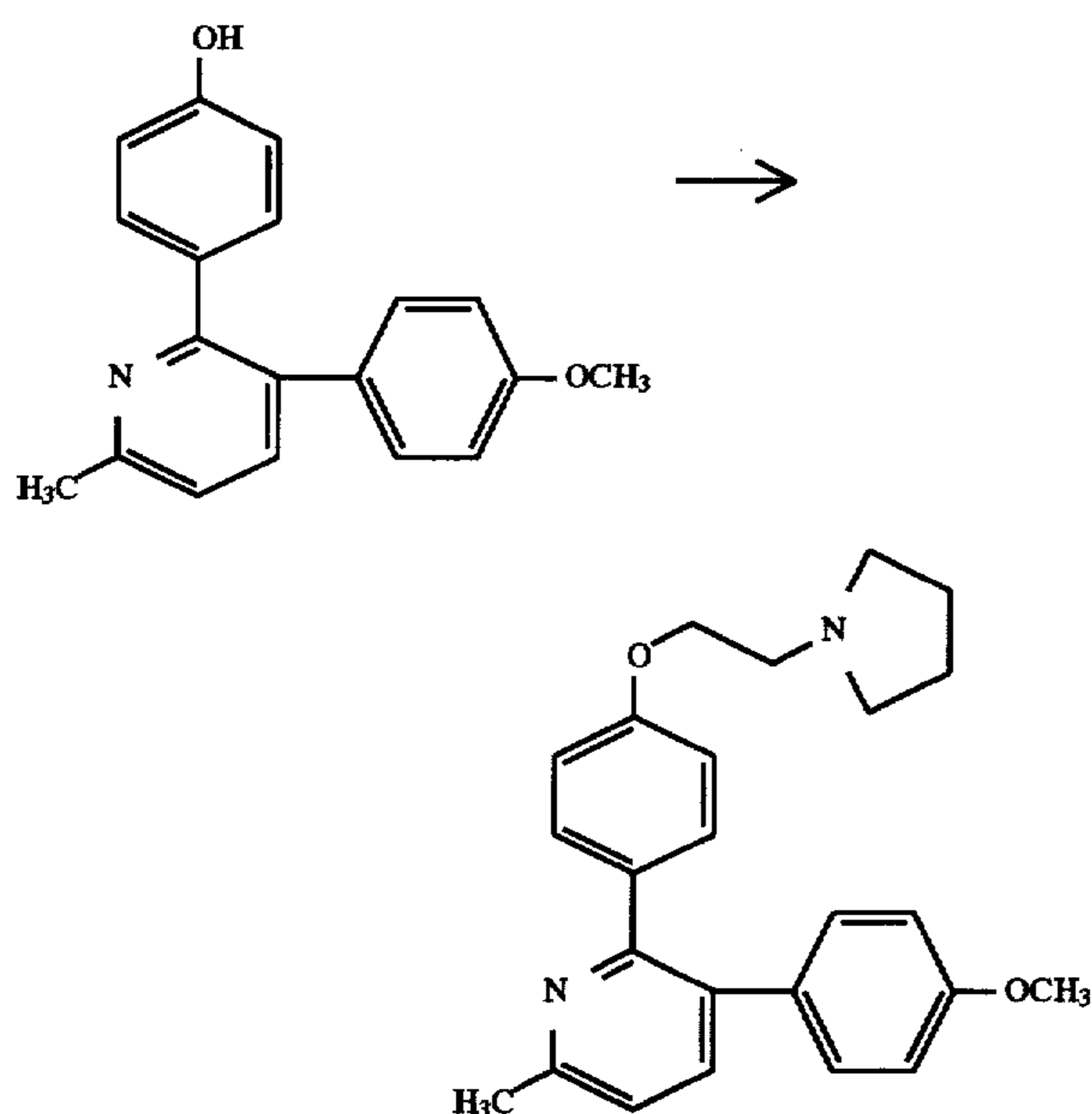
2-[4-[2-(1-Pyrrolidinyl)ethoxy]phenyl]-3-(4-methoxyphenyl)-6-methylpyridine
