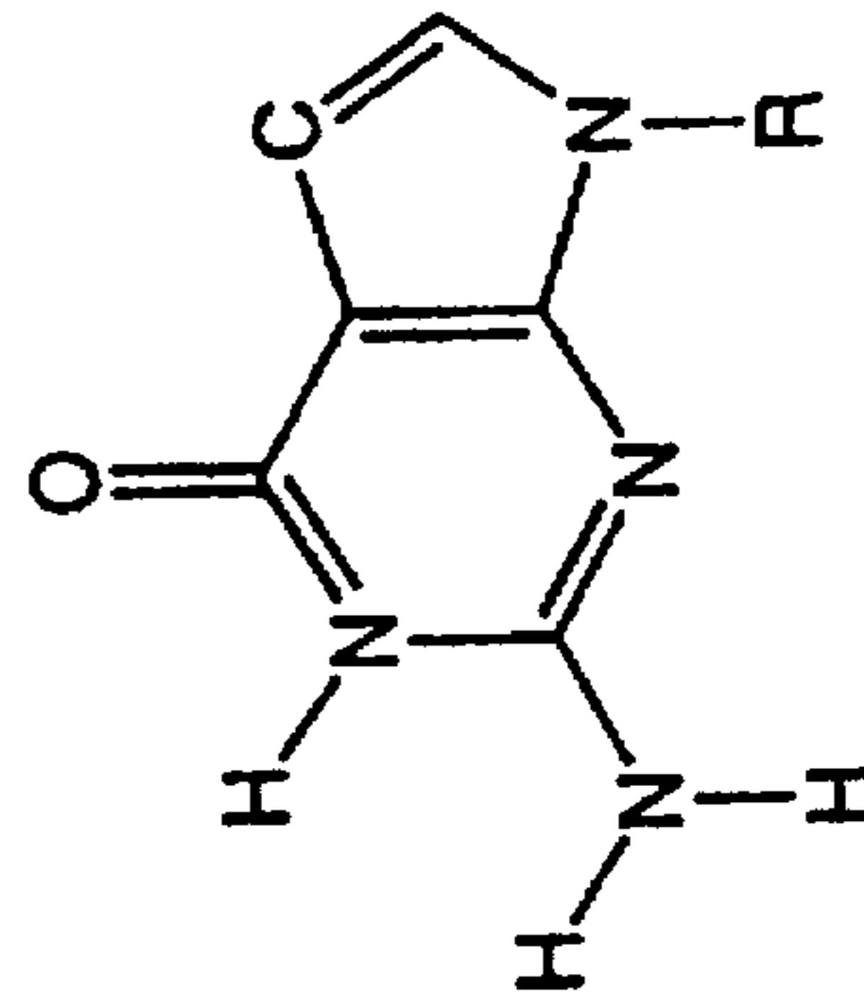
7-Deaza-Guanine
