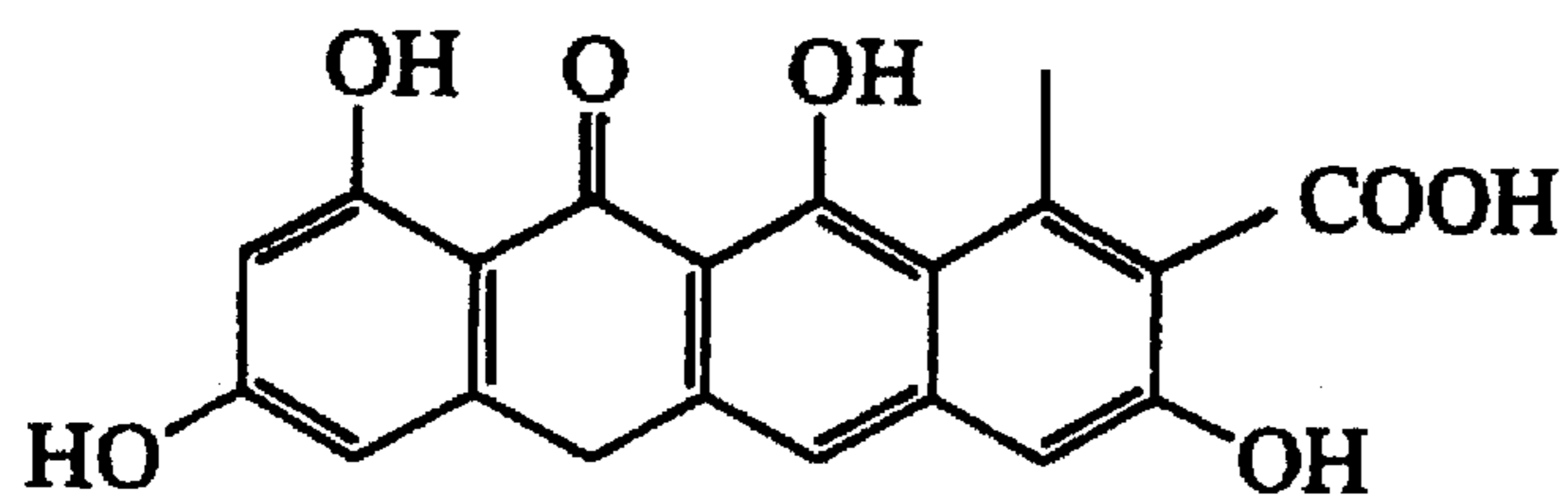
TETRACENOMYCIN F1 (5)
