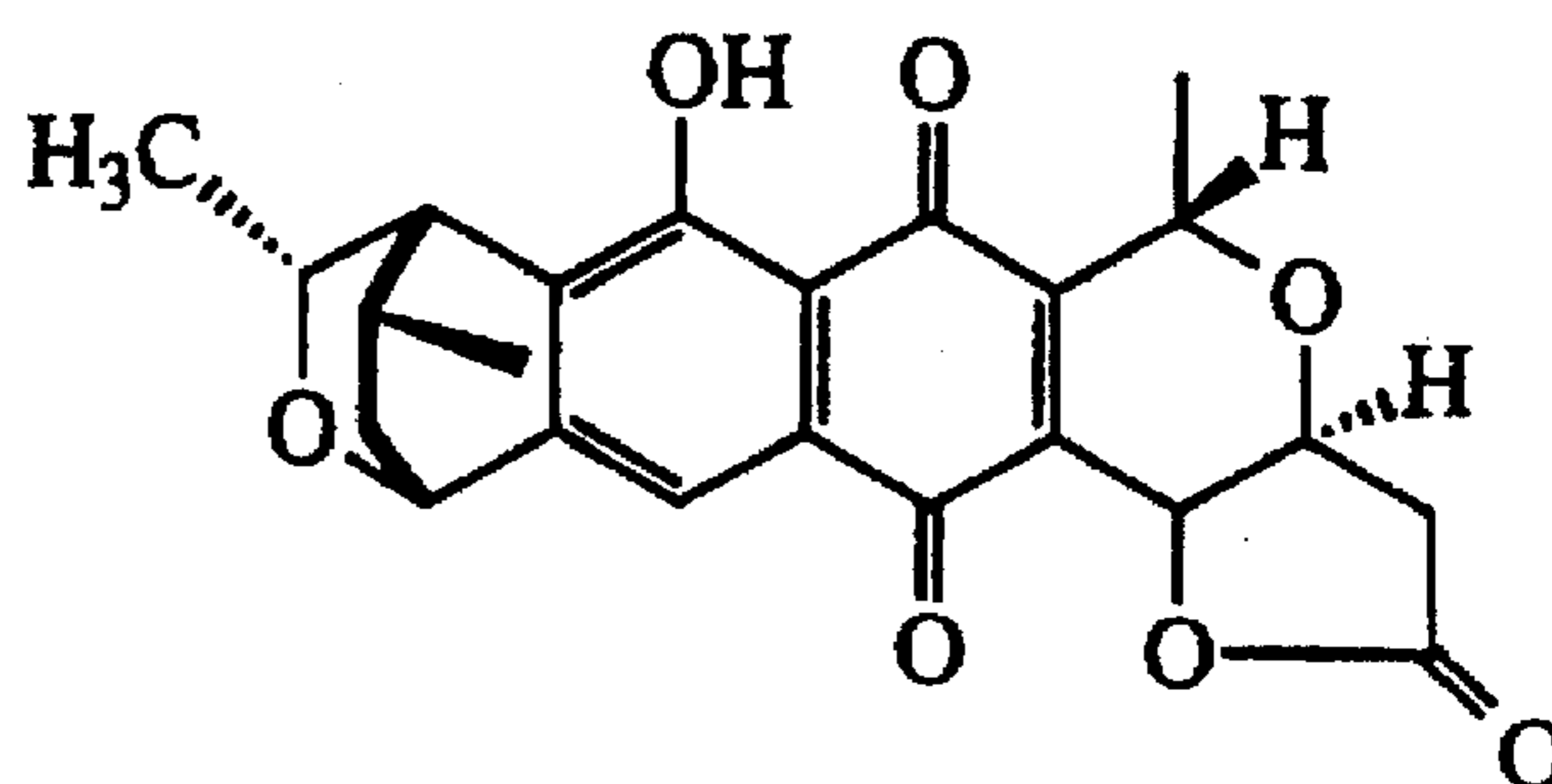
GRANATICIN (4)
