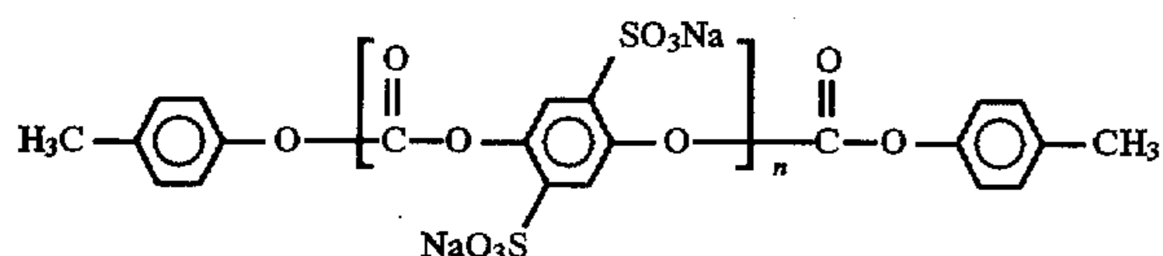
Oligomer A (n=6)
