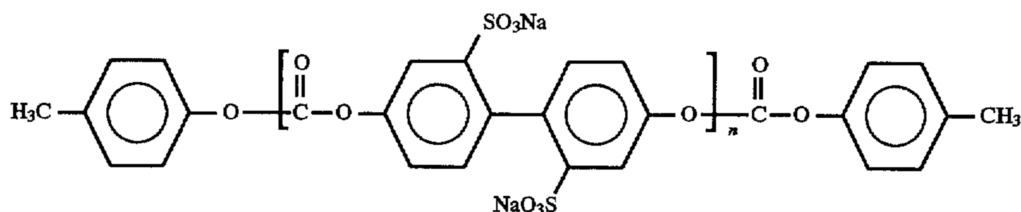
Oligomer A (n=6)
