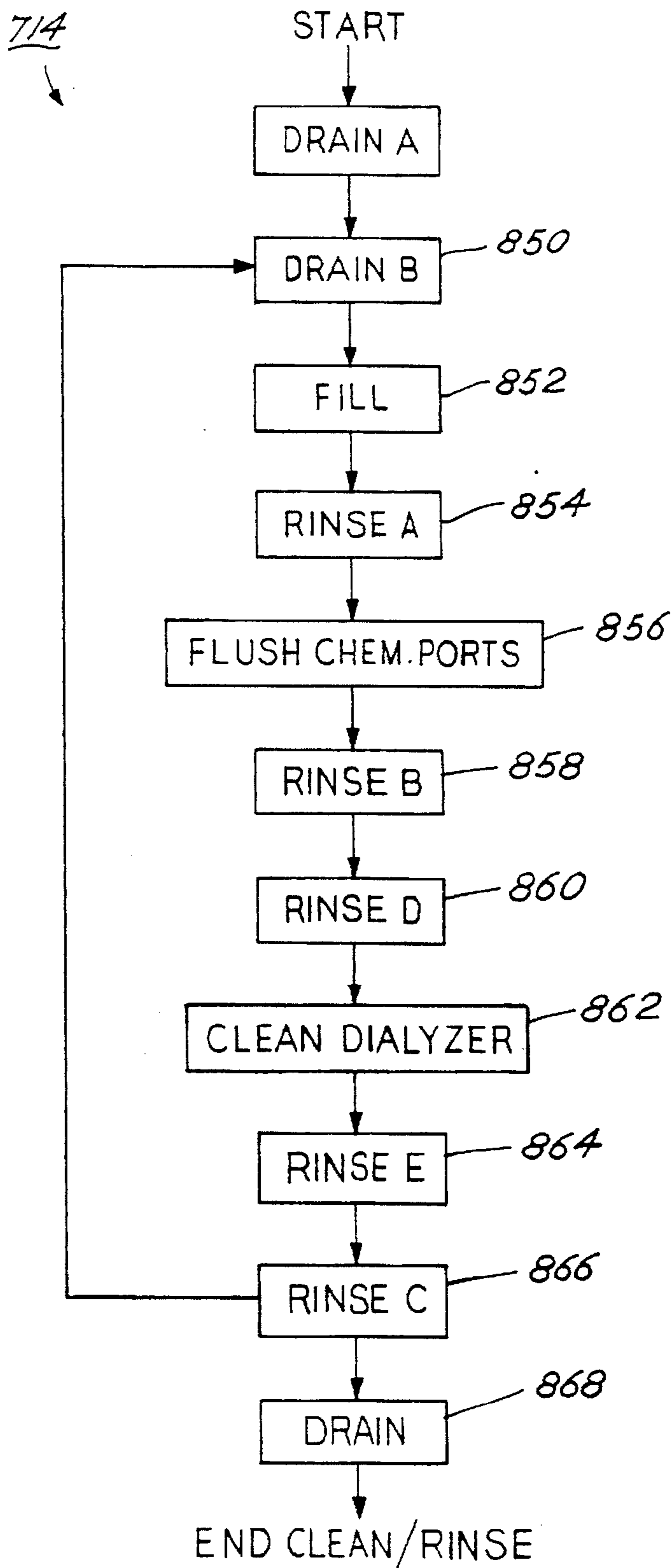
FIG. 23 CLEAN/RINSE
