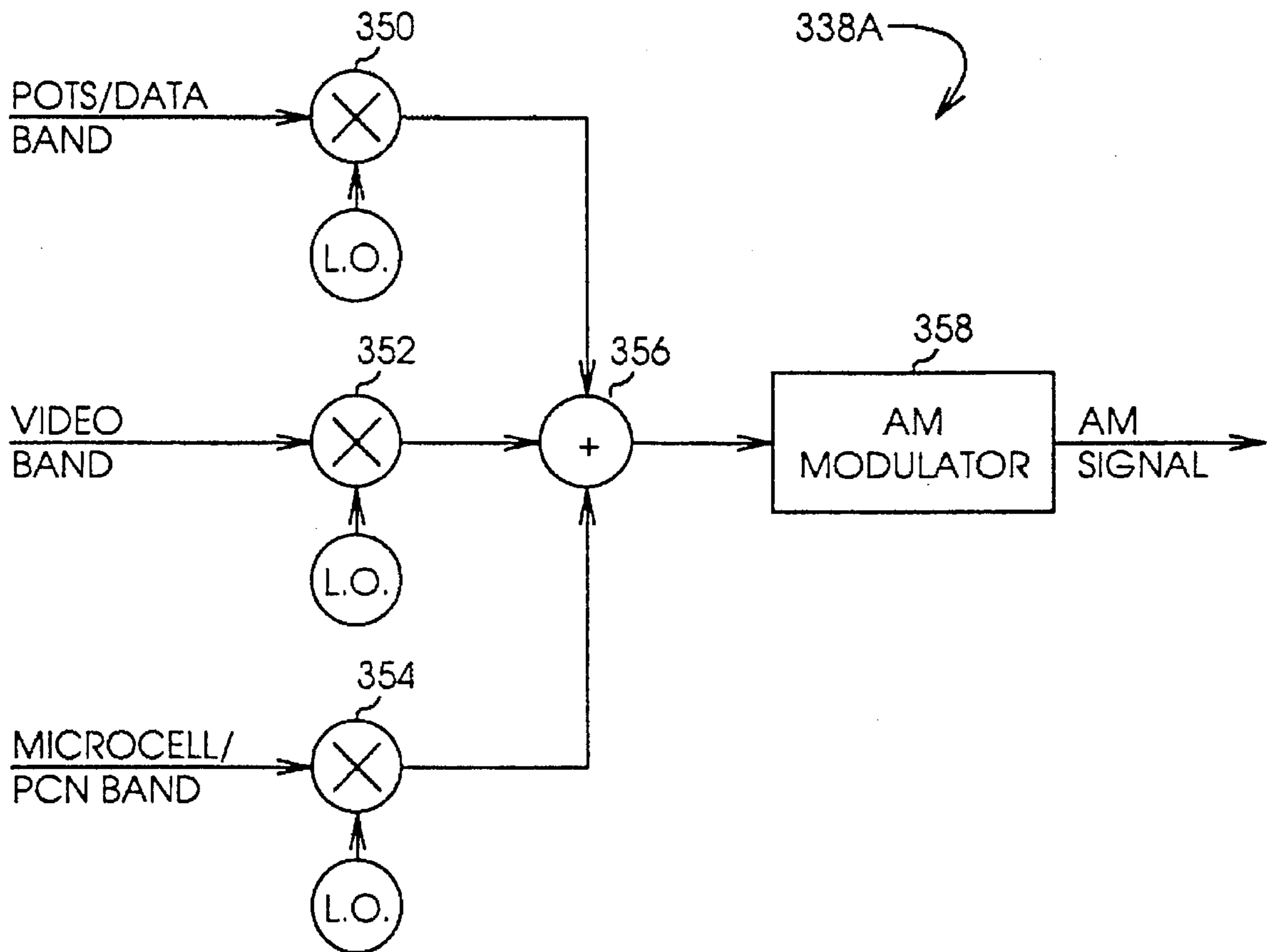
AM Modulator Fig. 25
