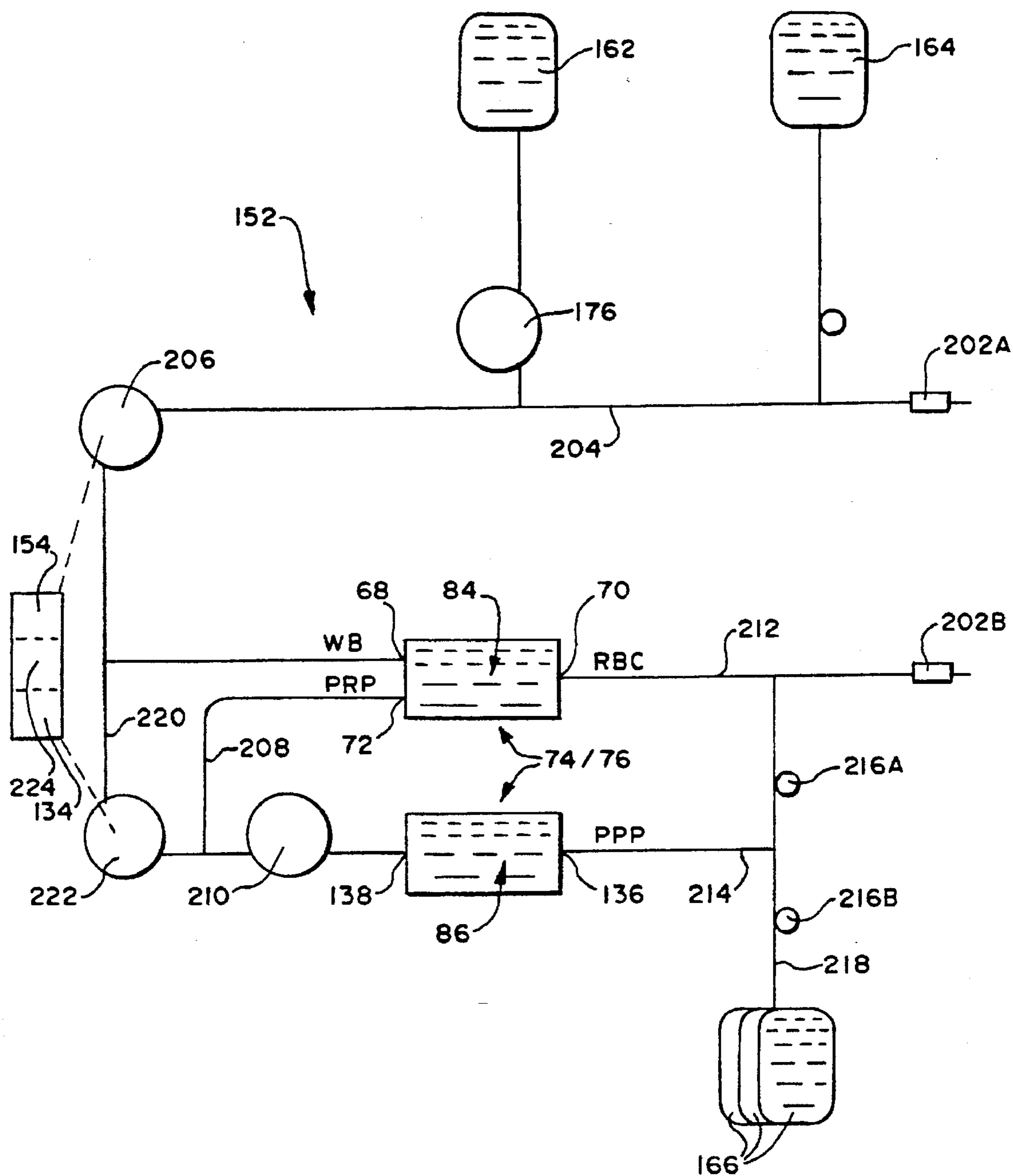
FIG. 28
