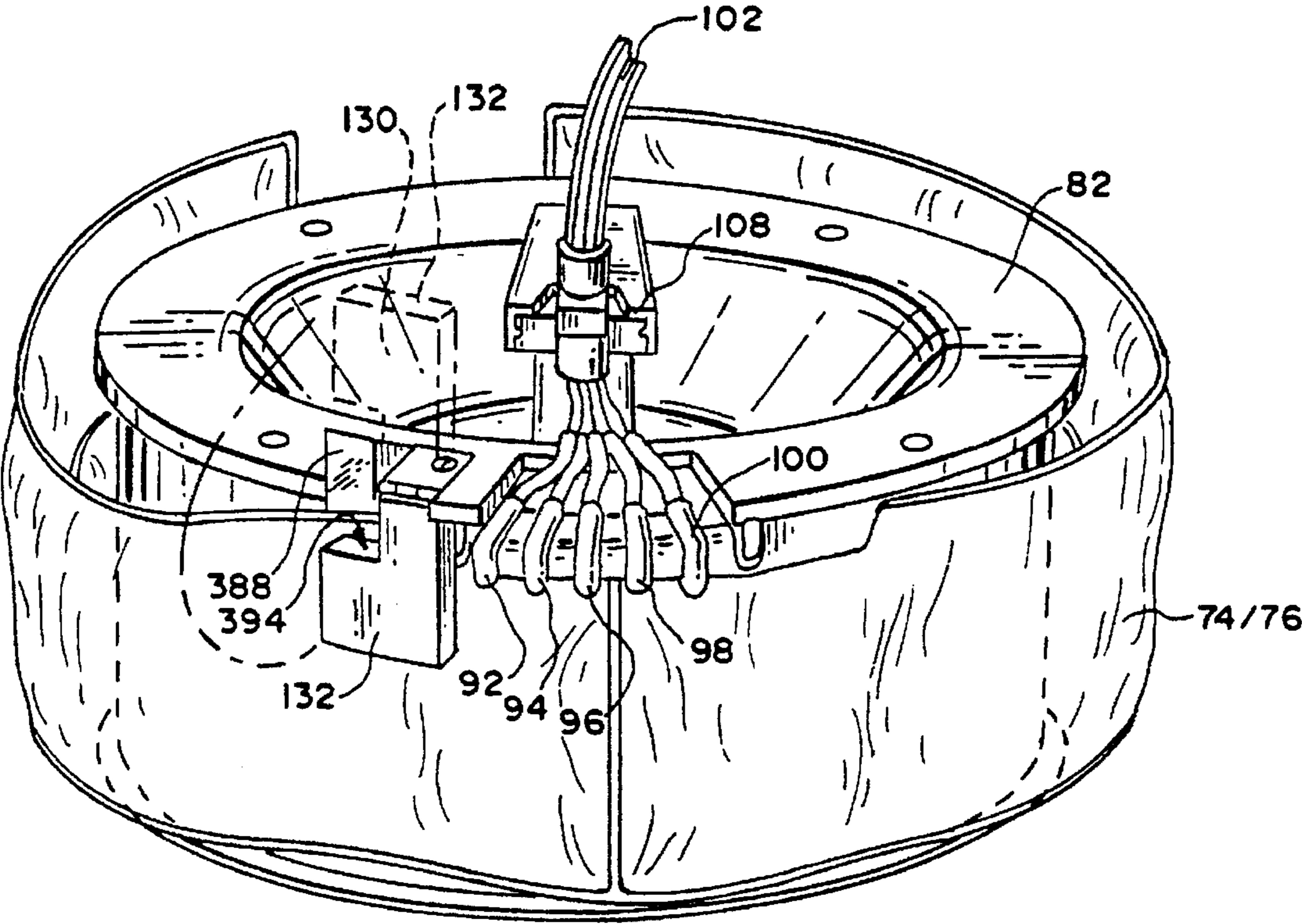
FIG. 22
