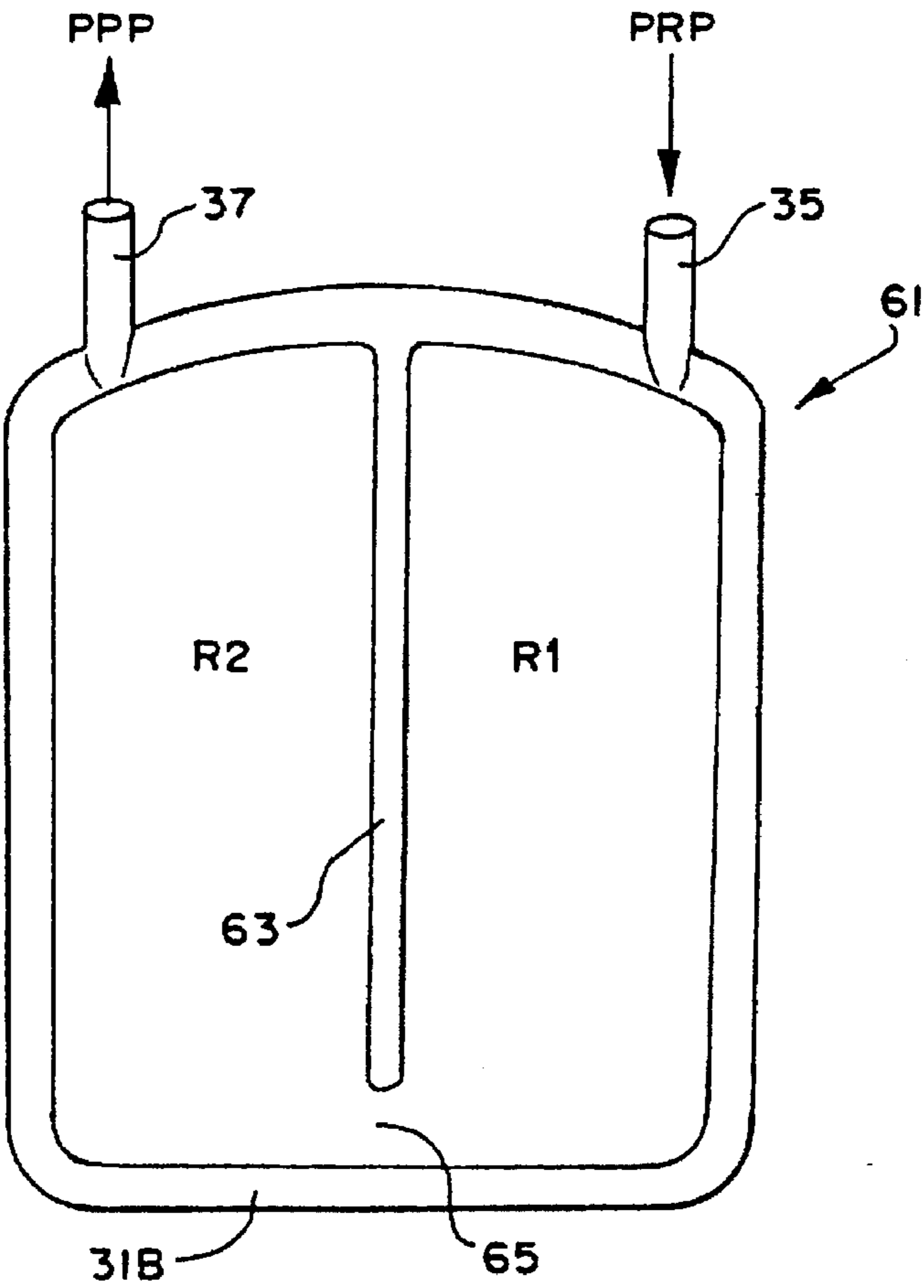
FIG. 10B
