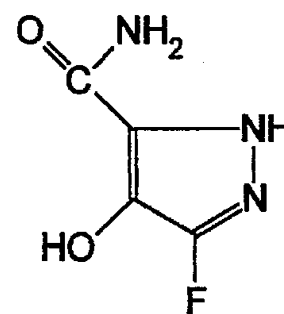
PYRAZOMYCIN
