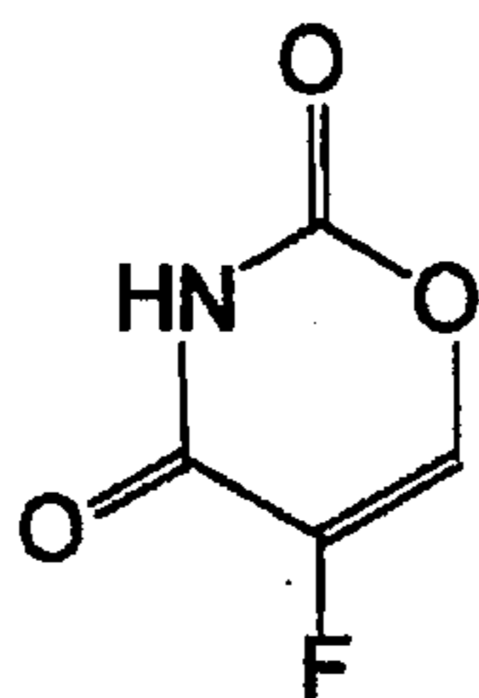
MINIMYCIN
