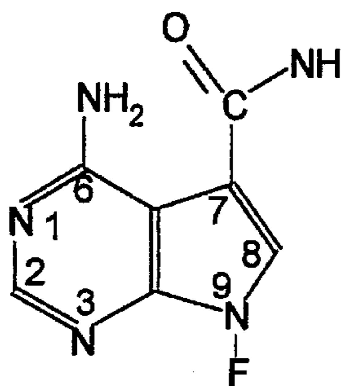
SANGIVAMYCIN
