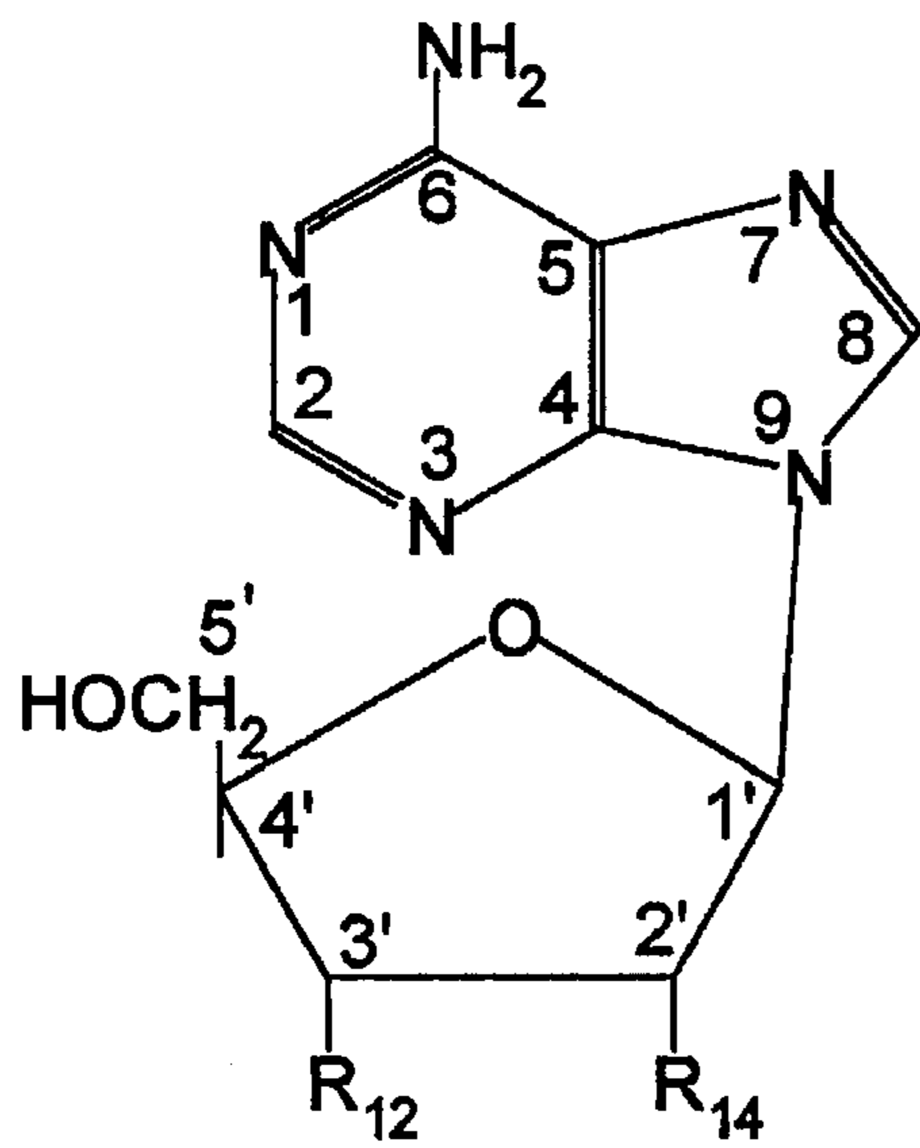
Adenosine
