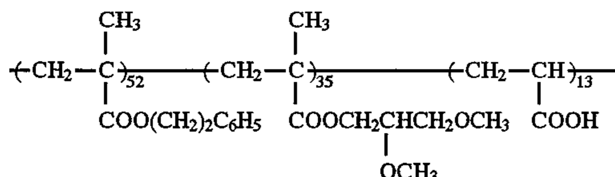
Resin (A-4)
