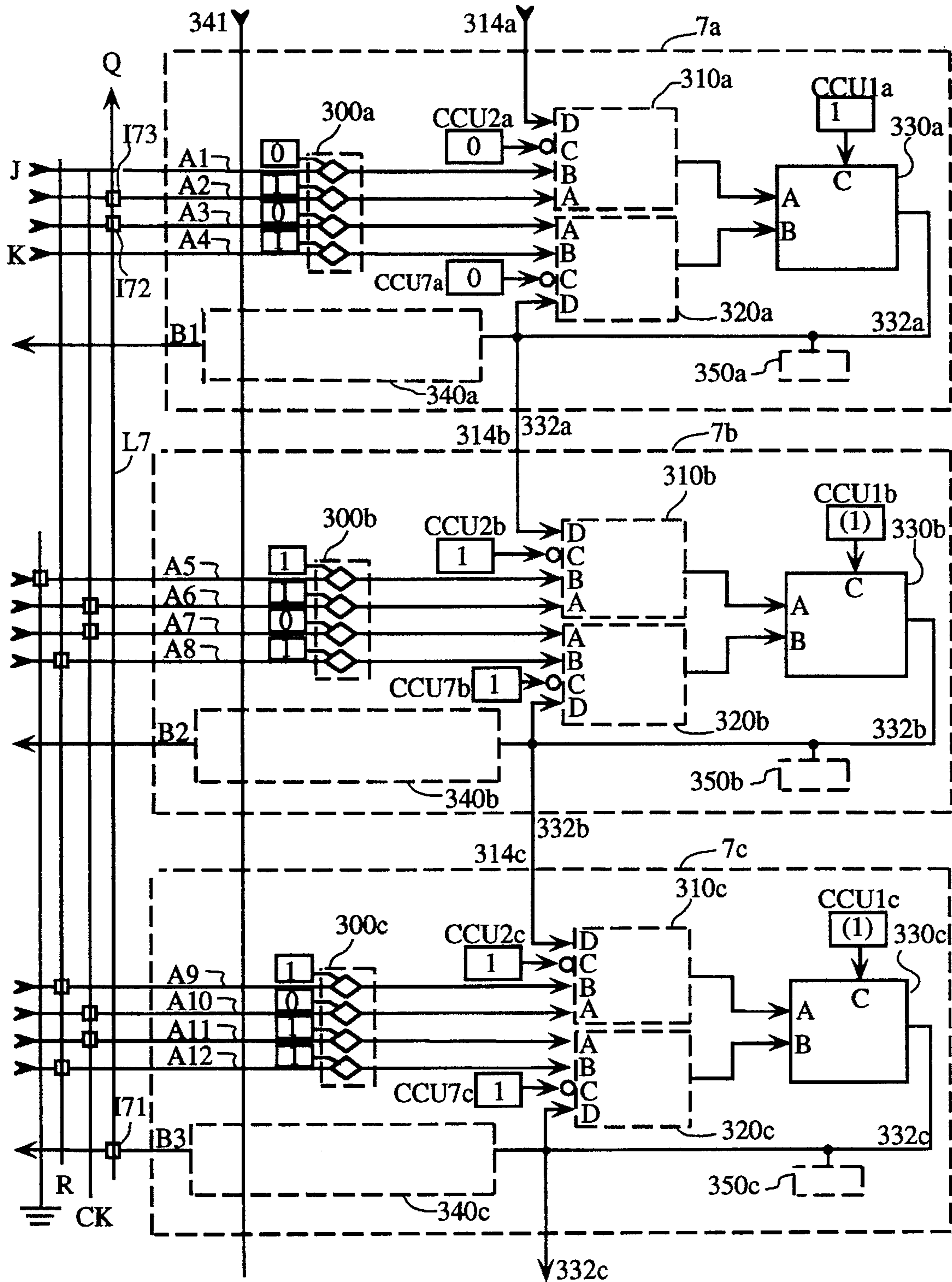
FIG. 14B JK FLIP FLOP
