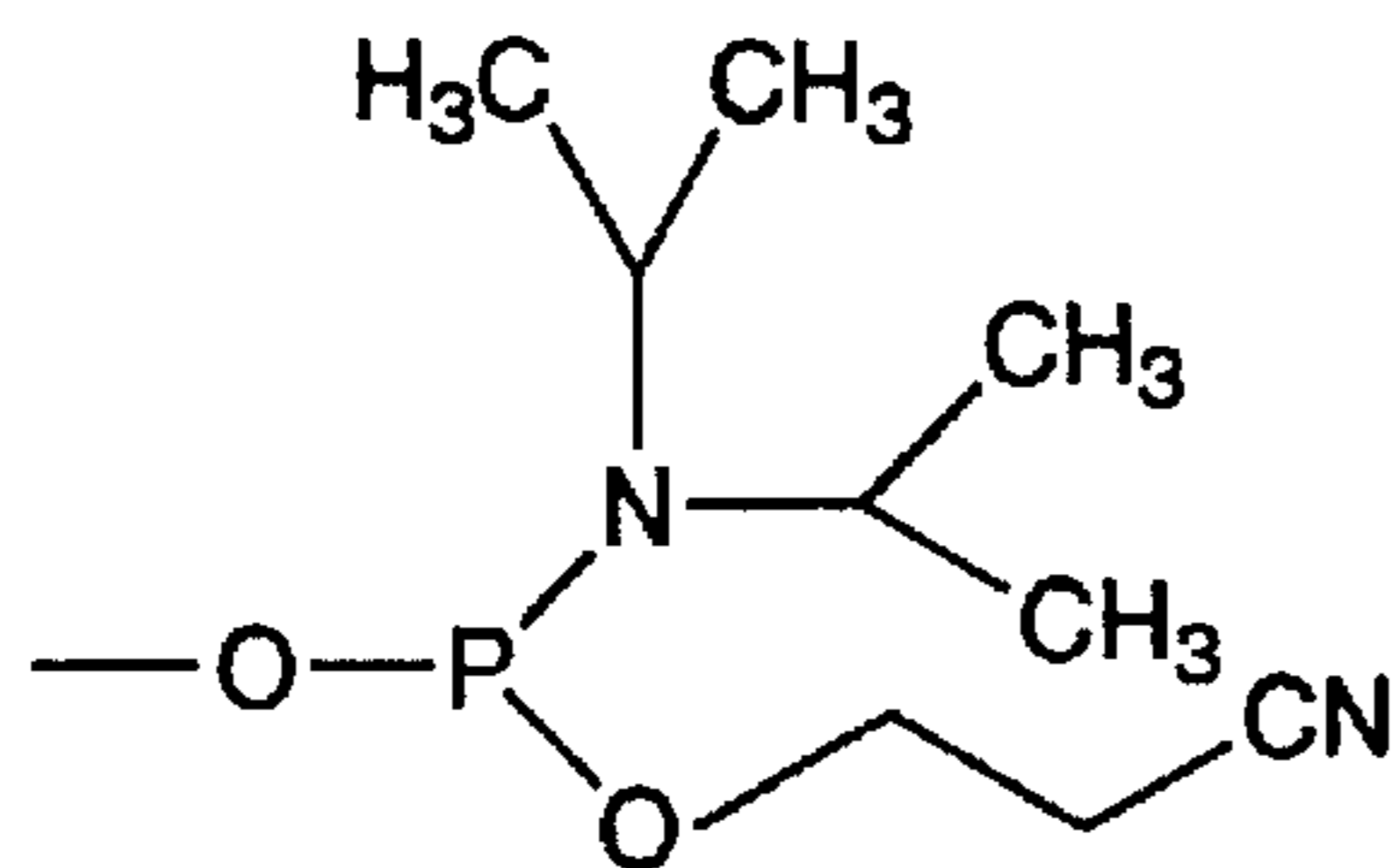
N,N-diisopropylamino-β-cyanoethoxyphosphine
