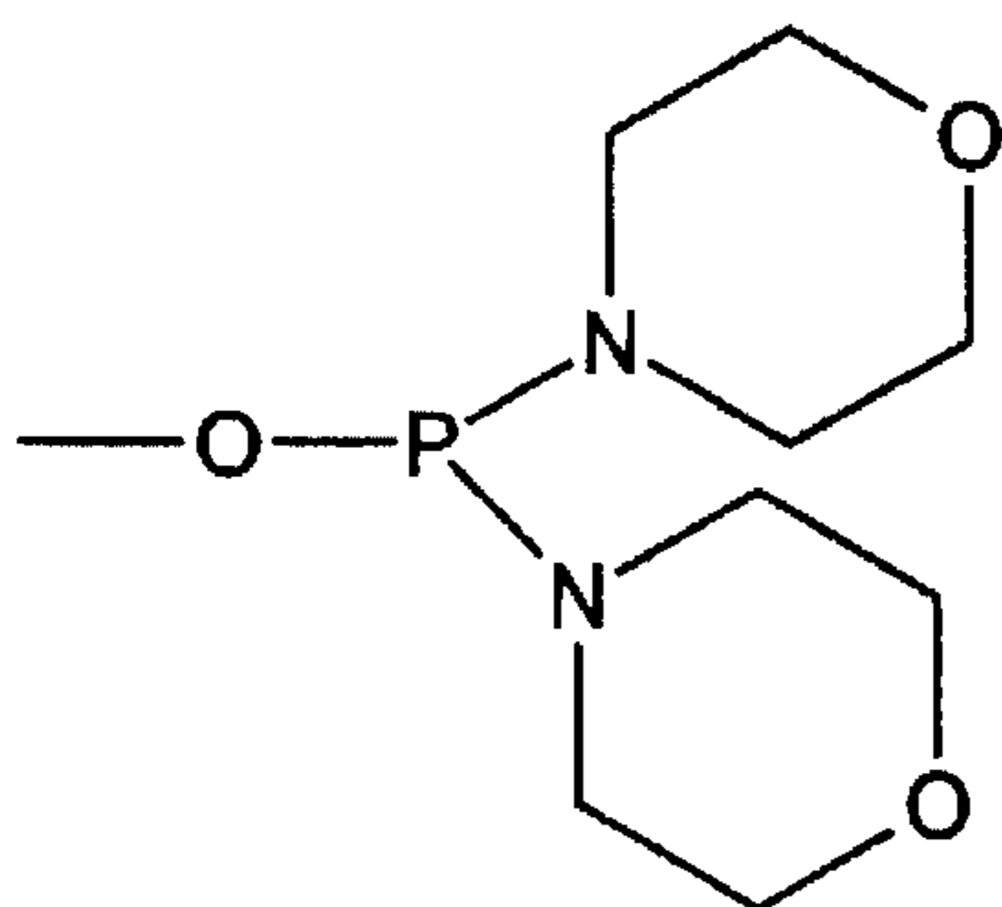
Bis morpholino-phosphine
