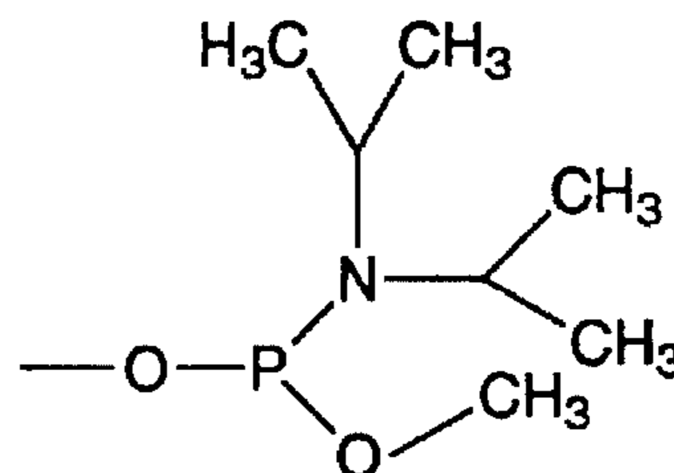
N,N-diisopropylamino-methoxyphosphine
