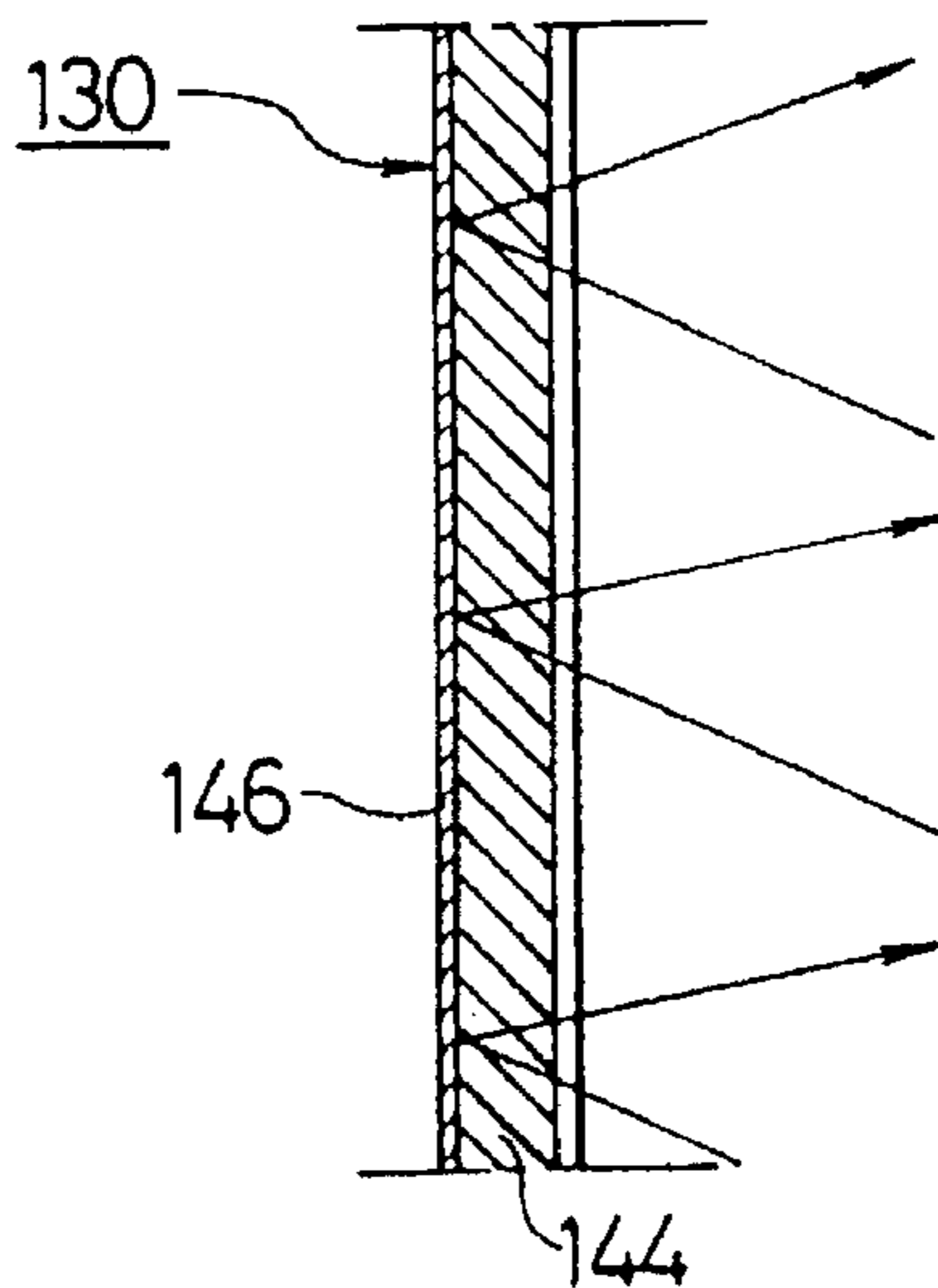
FIG. 29
