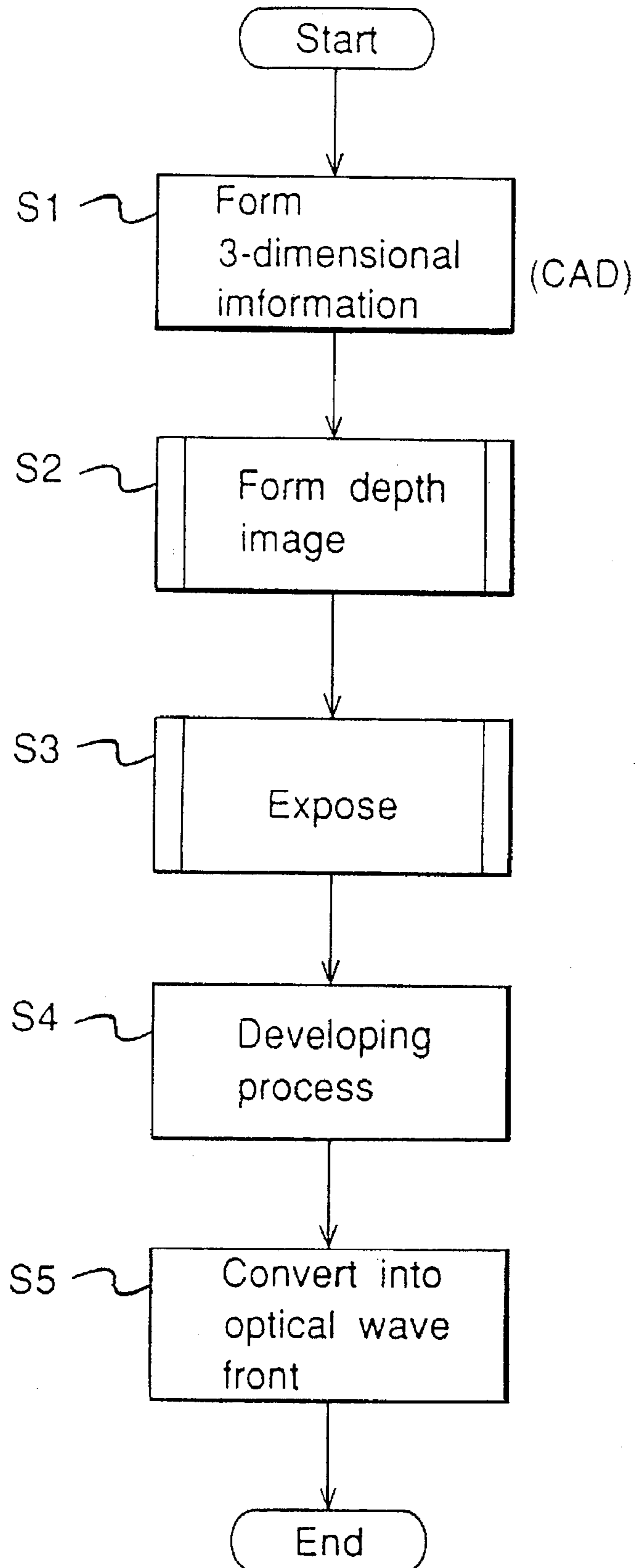
FIG. 39
