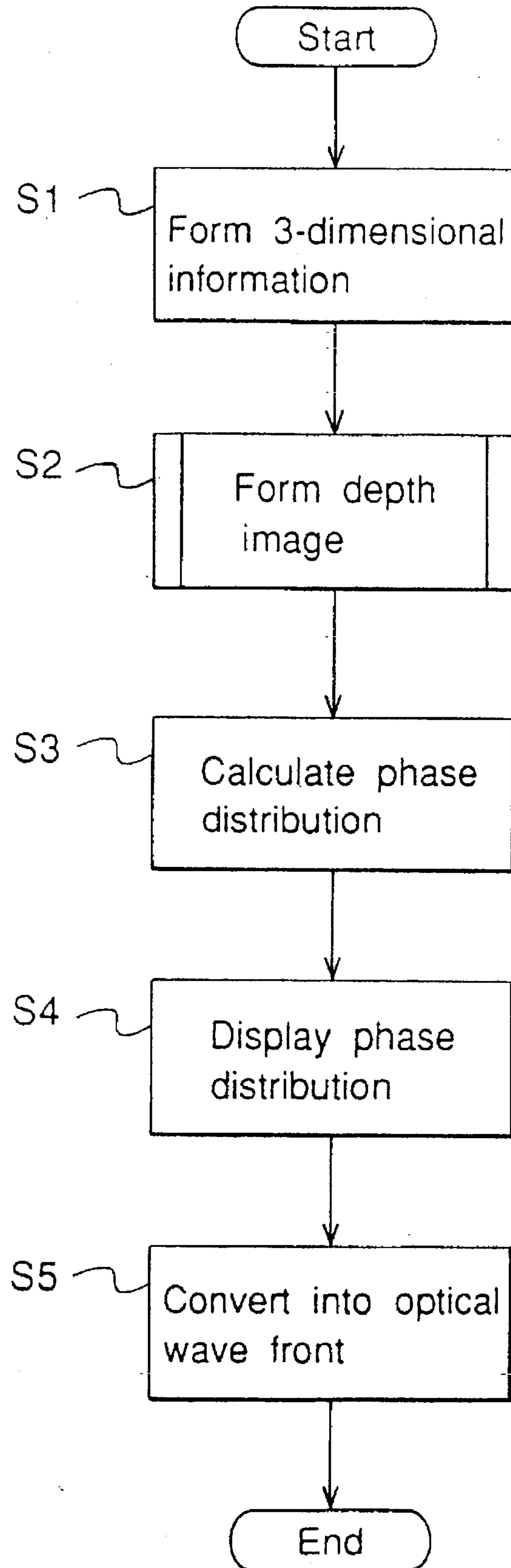
FIG. 1
