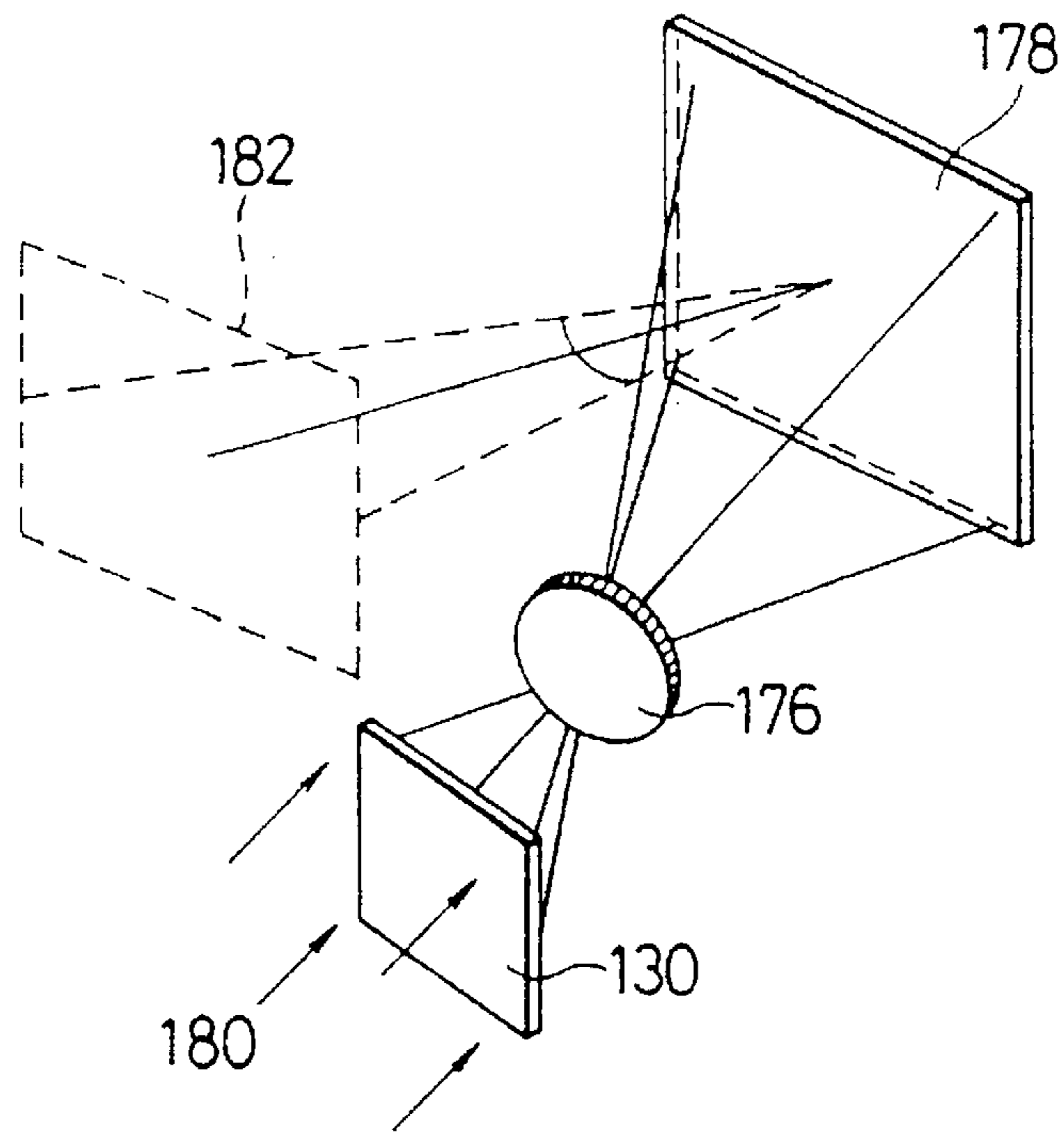
FIG. 32
