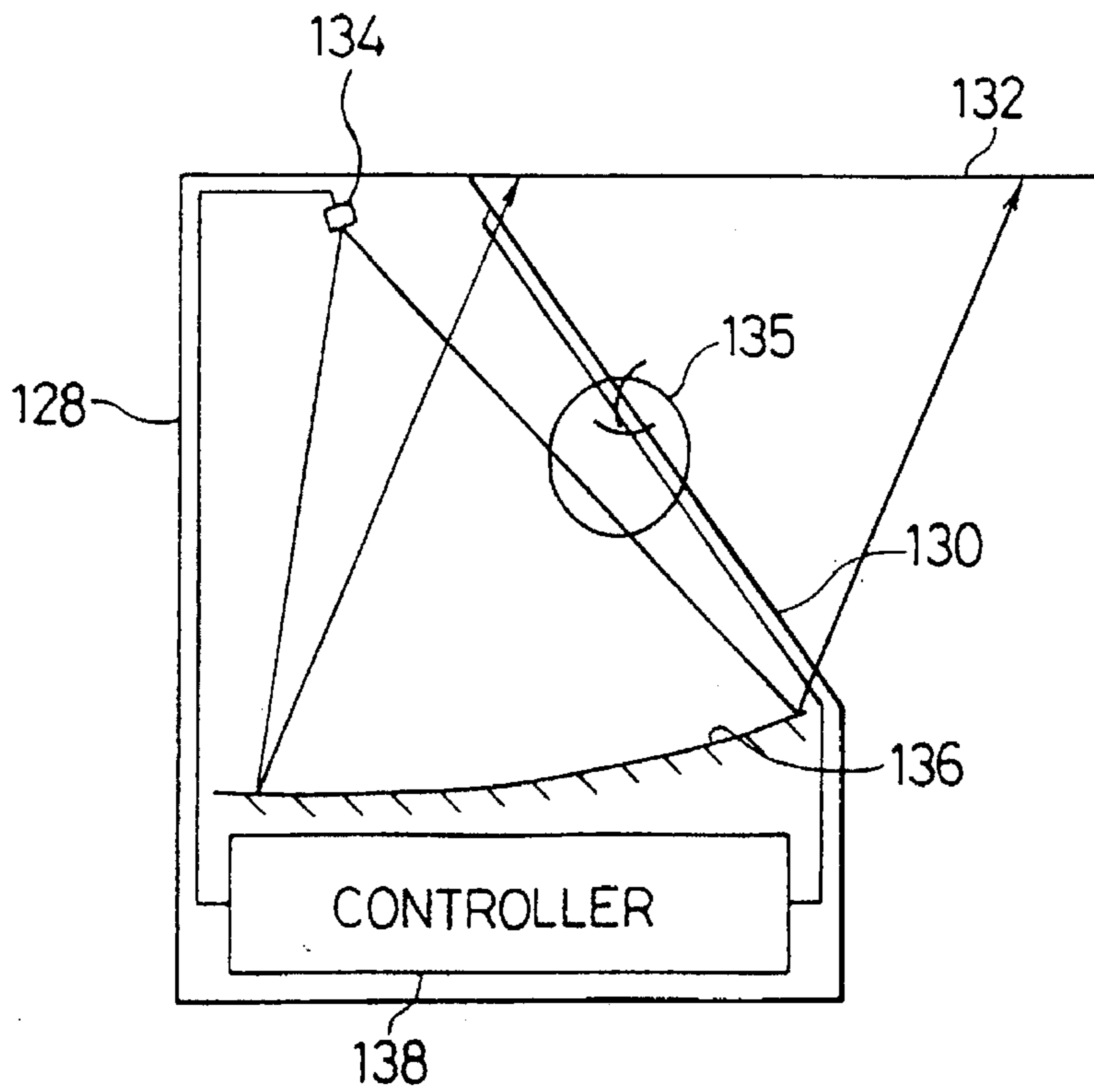
FIG. 25
