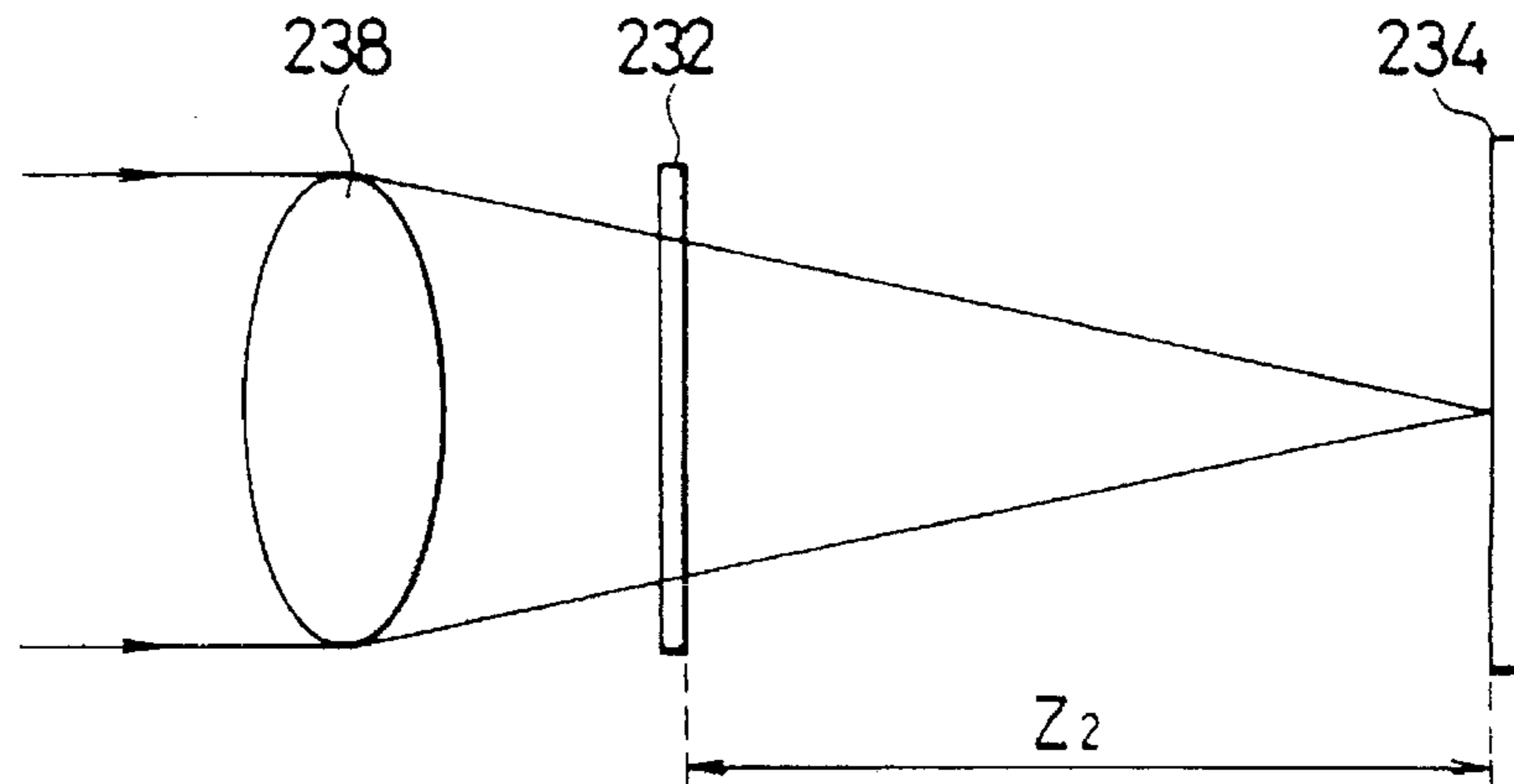
FIG. 42B
