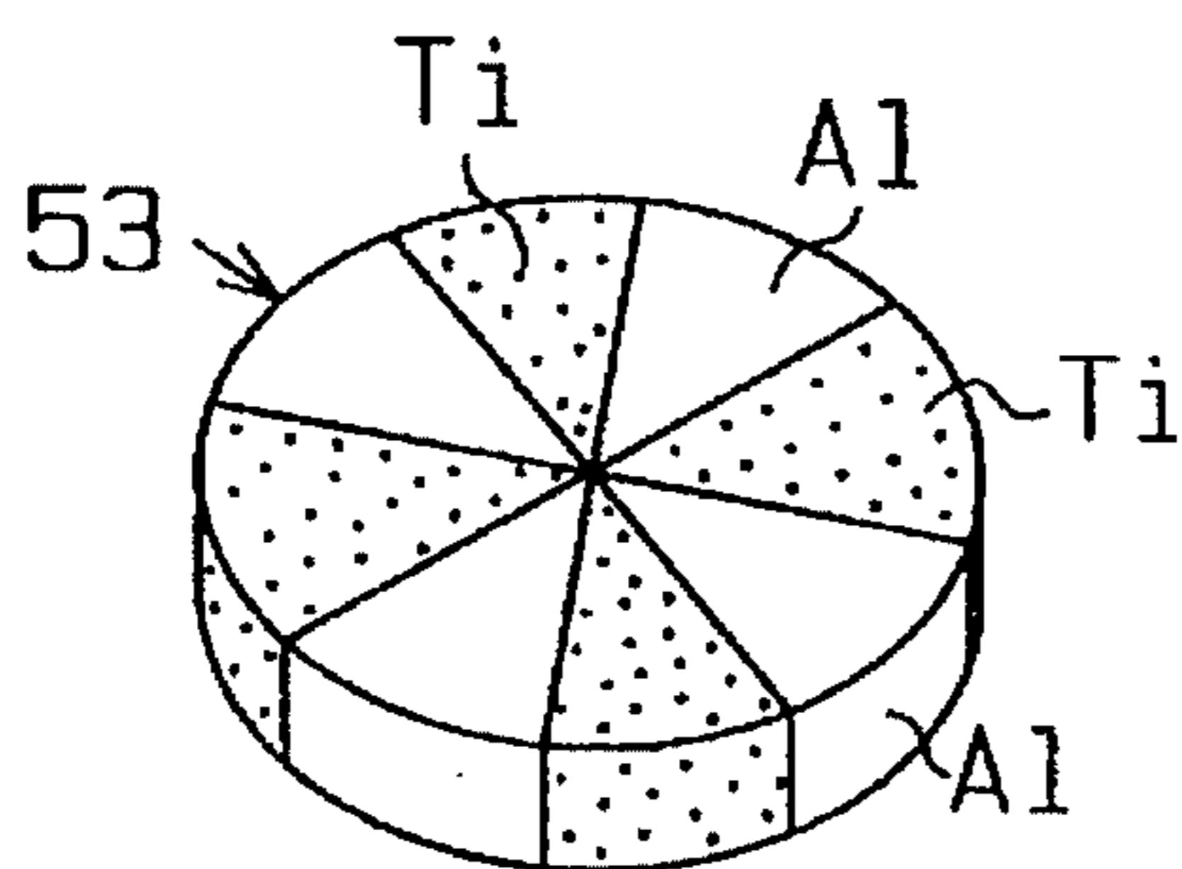
Fig. 15B
