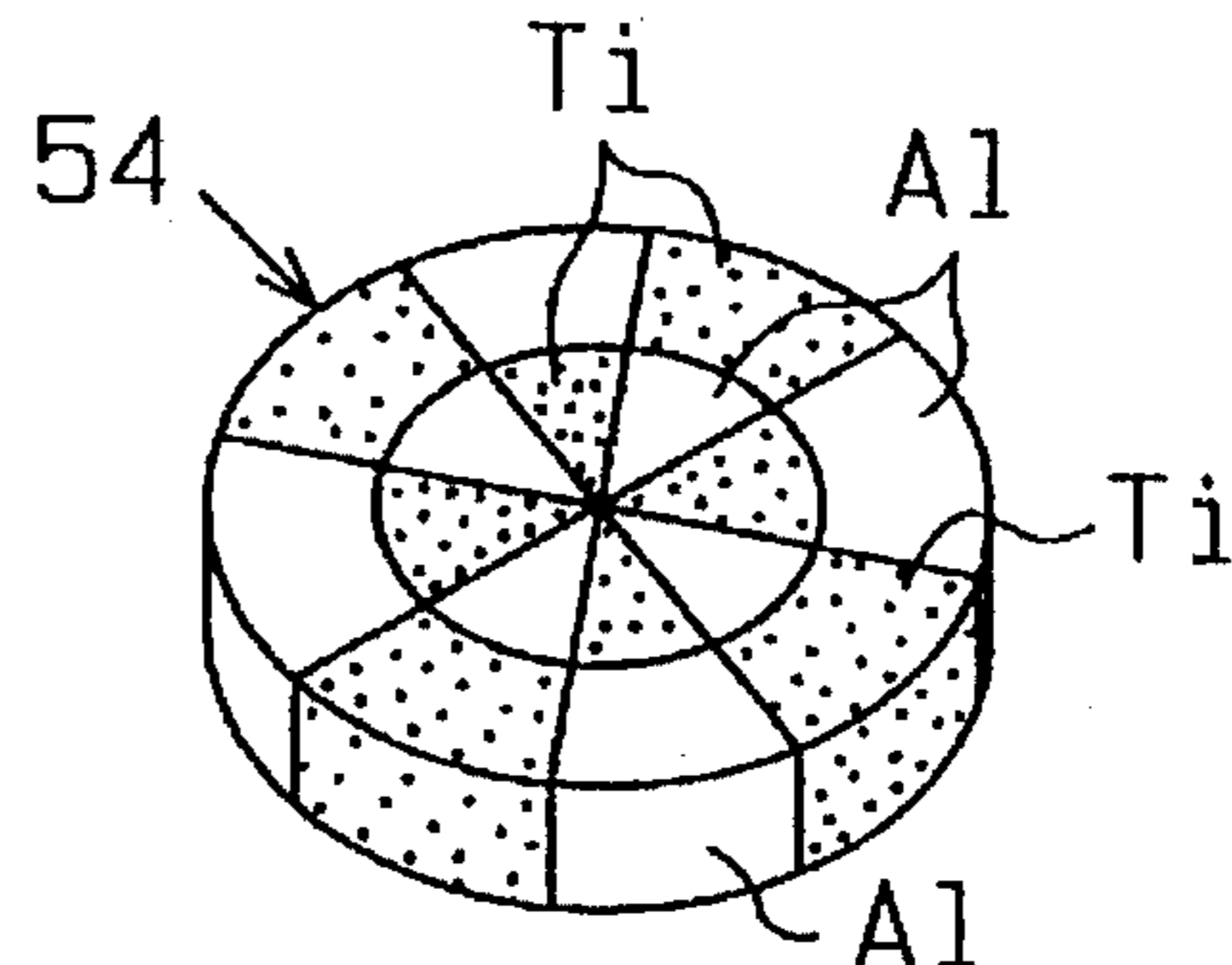
Fig. 15C
