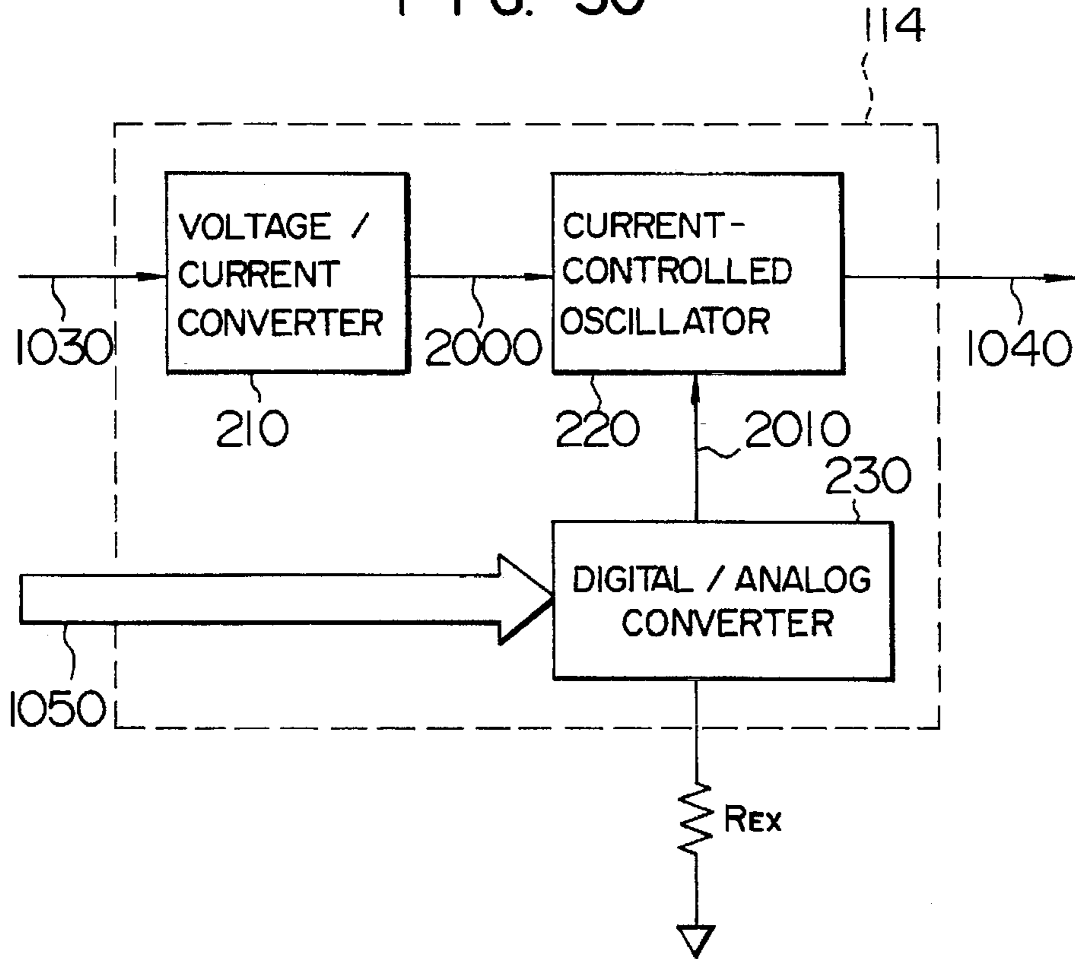
FIG. 30
