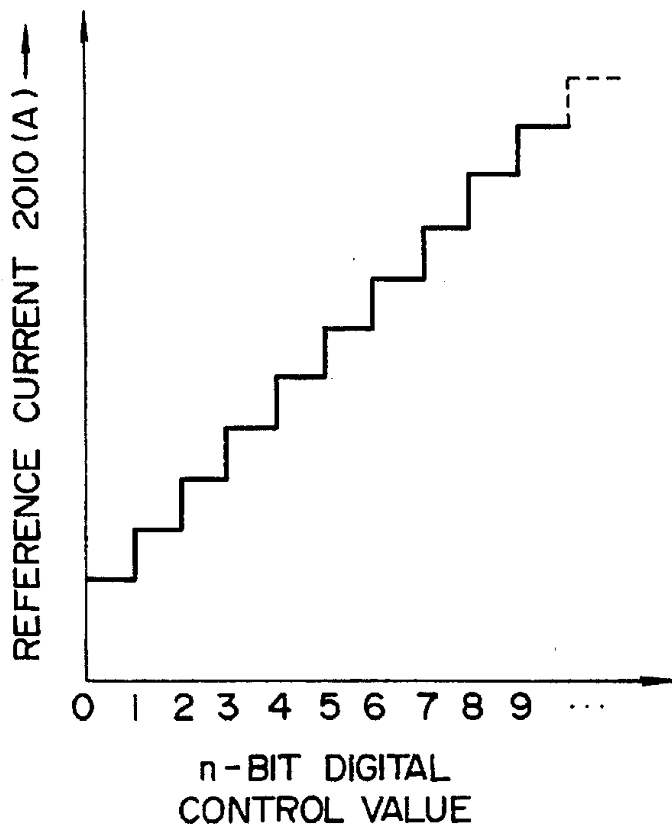
FIG. 31A
