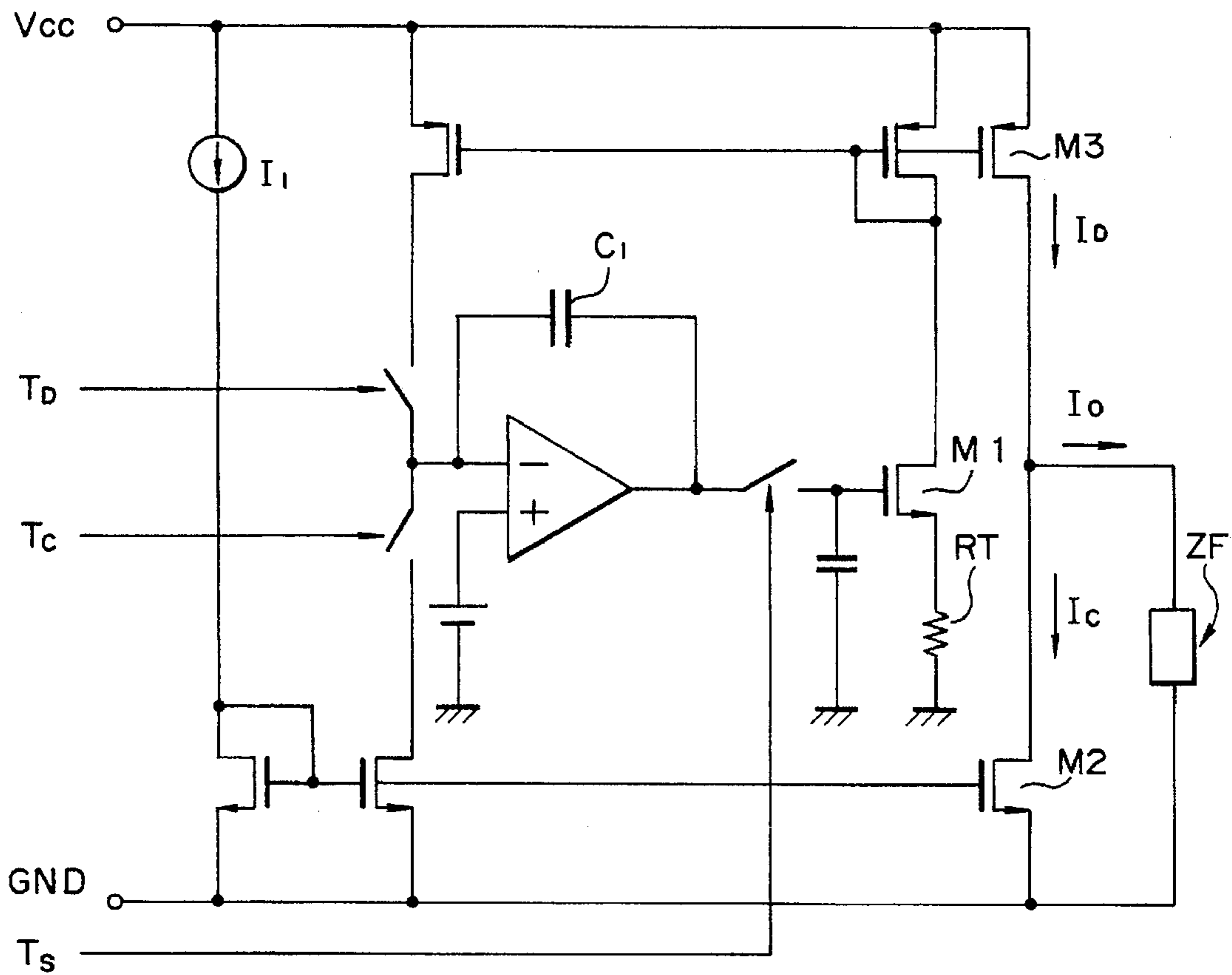
FIG. 27
