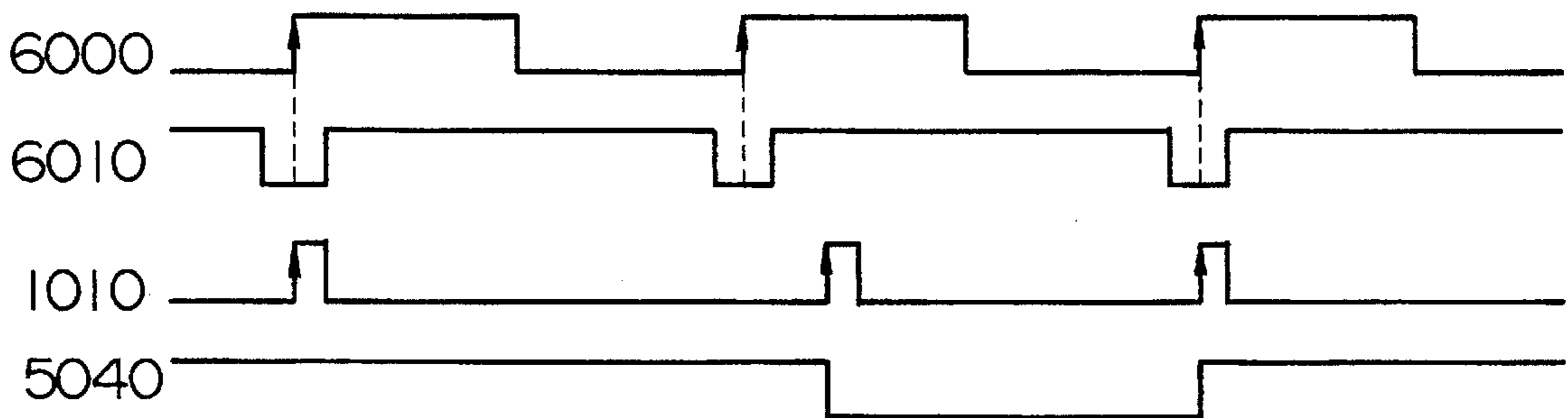
FIG. 40
