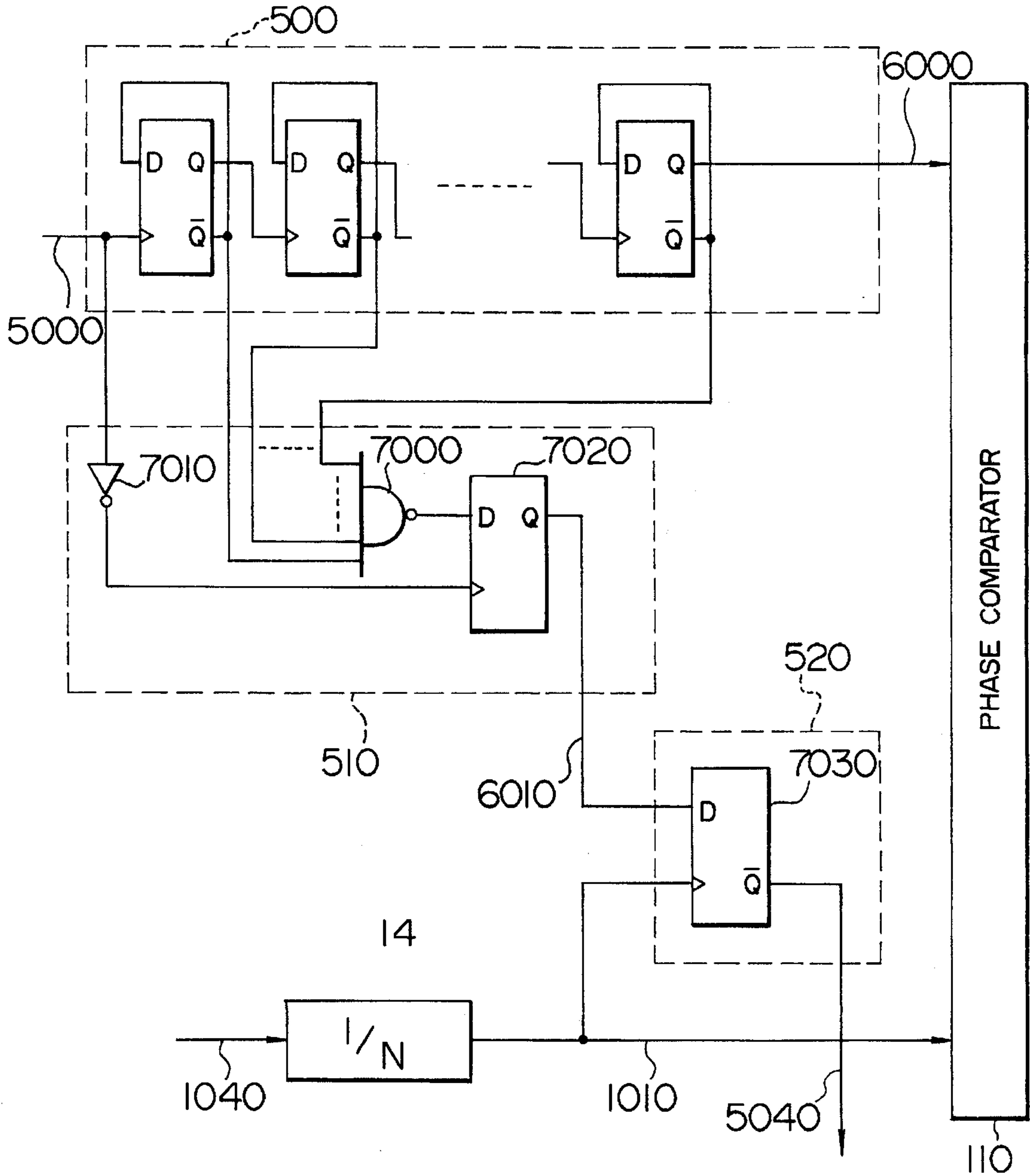
FIG. 40
