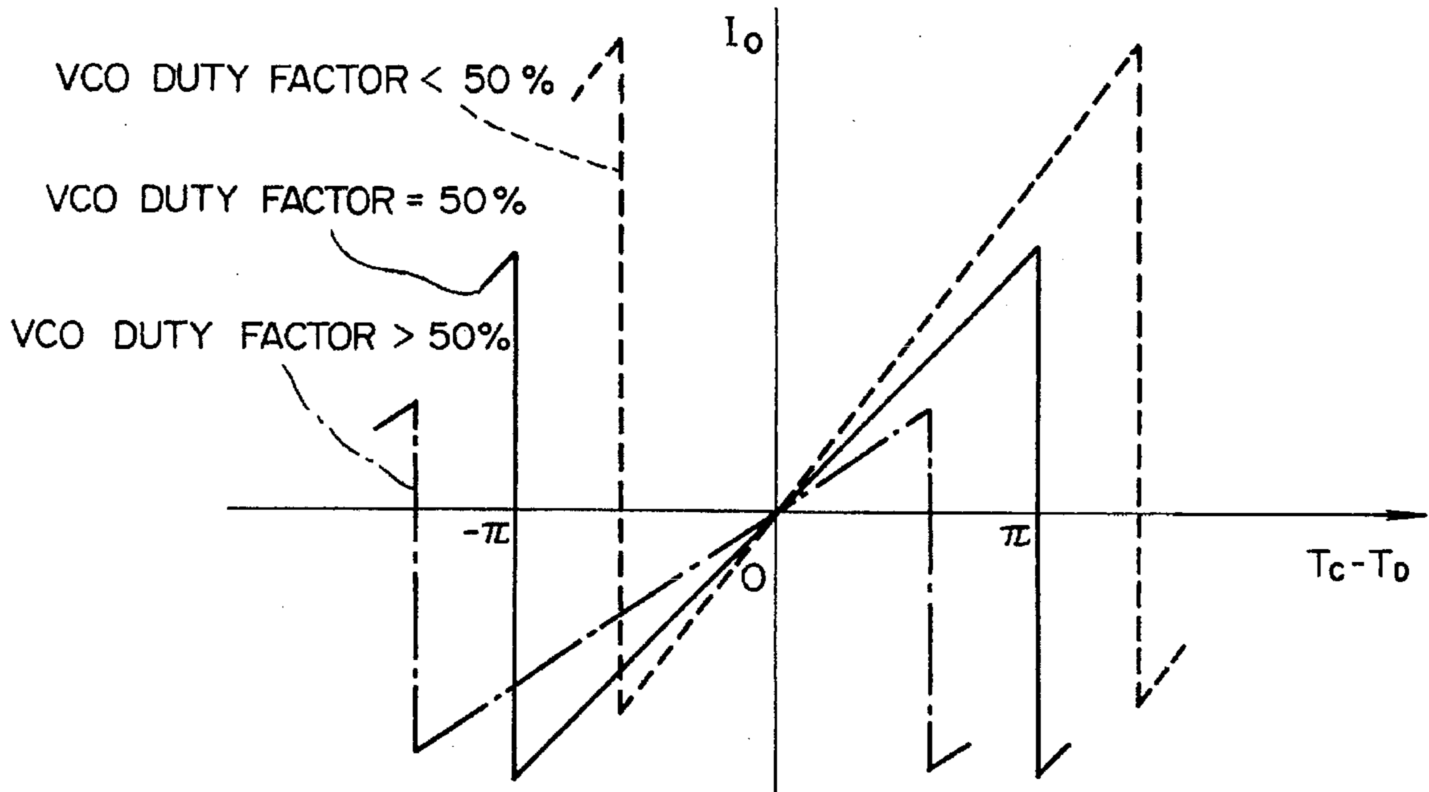
FIG. 27
