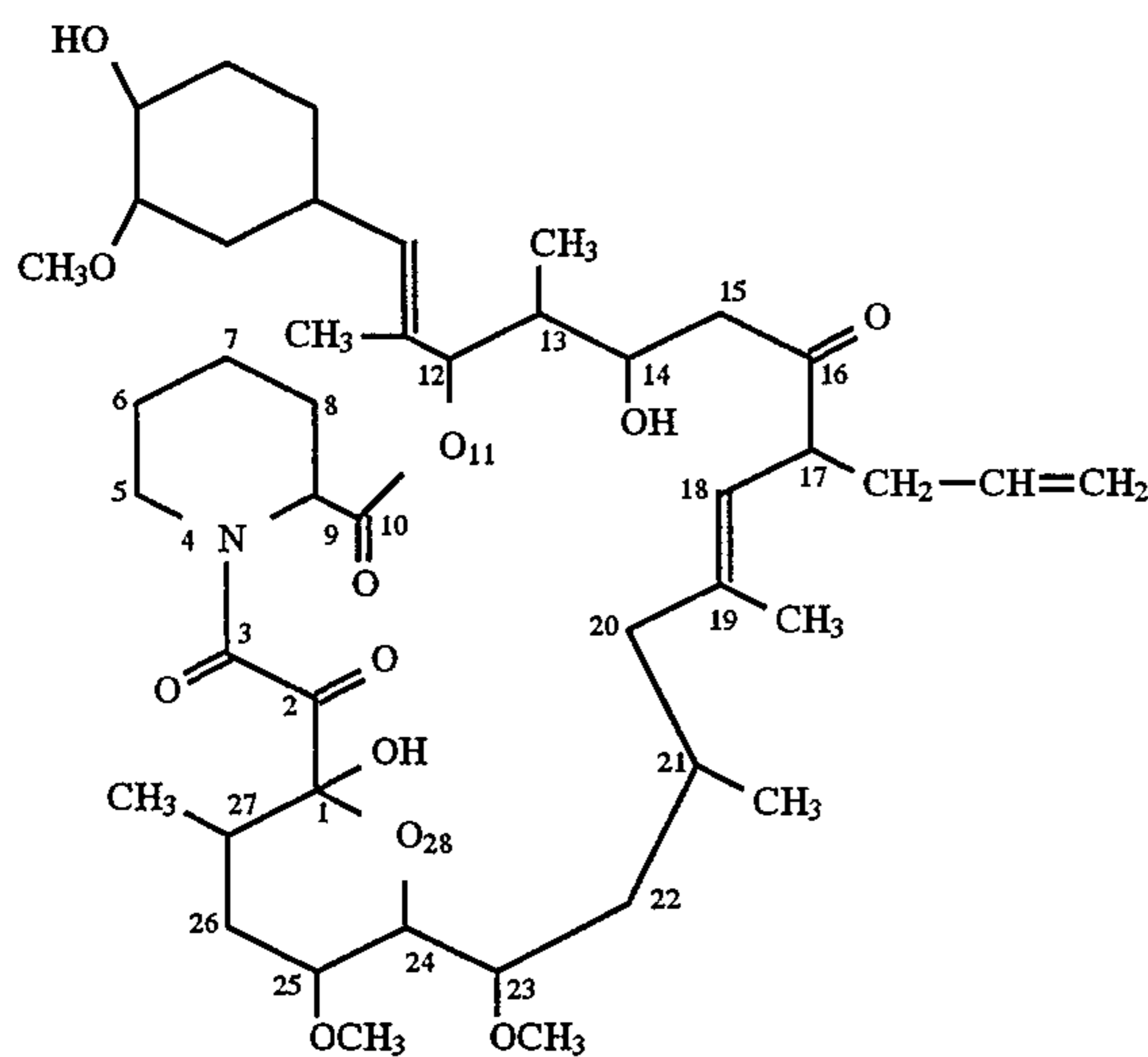
17-Allyl-1,14-dihydroxy-12-[2-(4-hydroxy-3-methoxycyclohexyl)-1-methylvinyl]-23,25-
