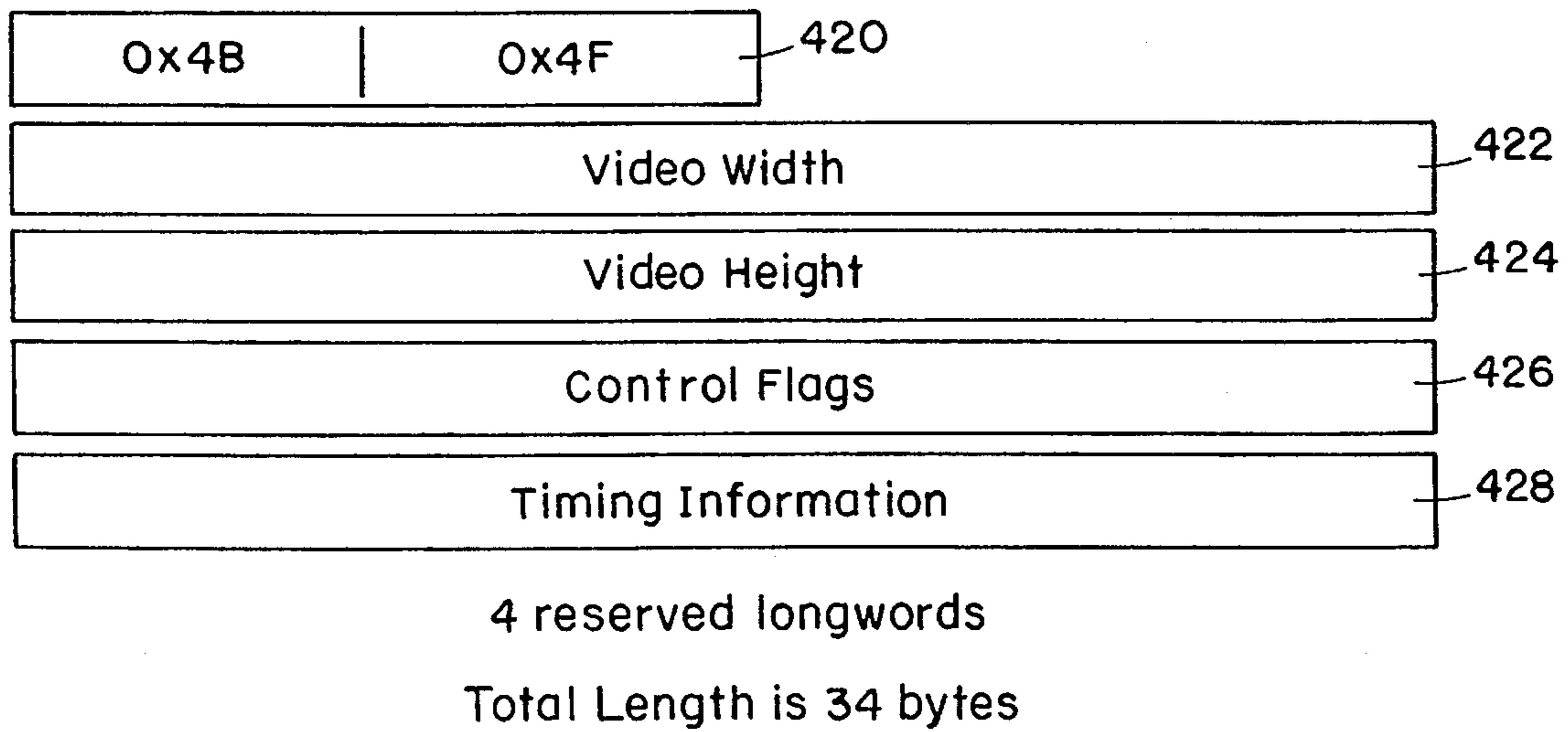
FIG. 16
