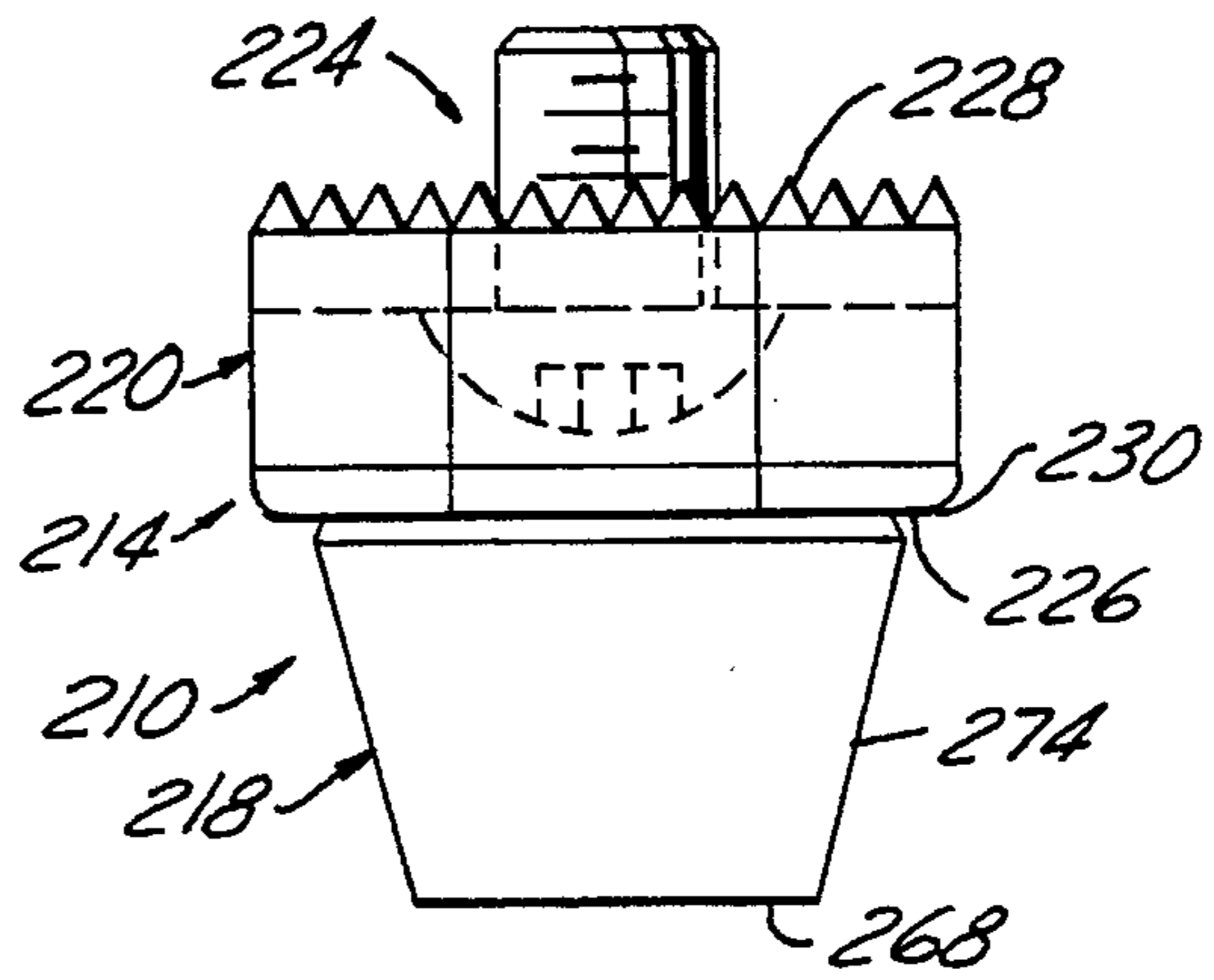
FIG. 18
