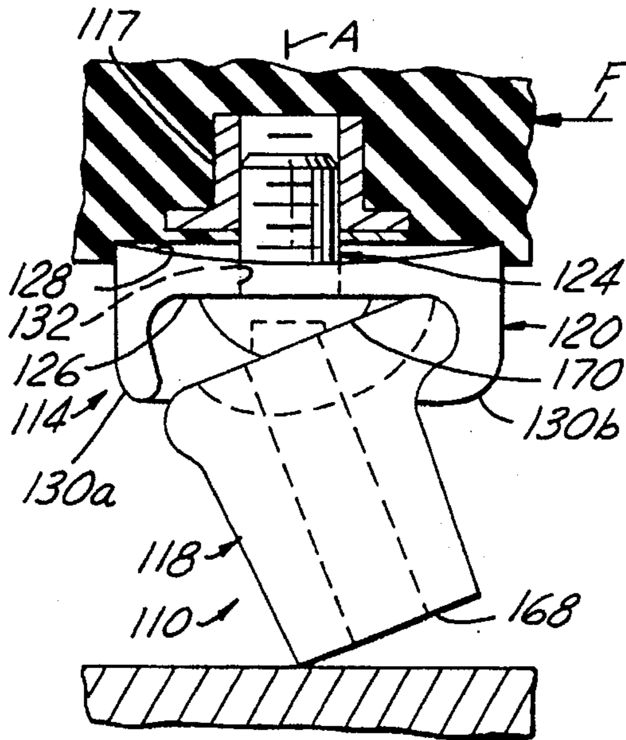
FIG. 13
