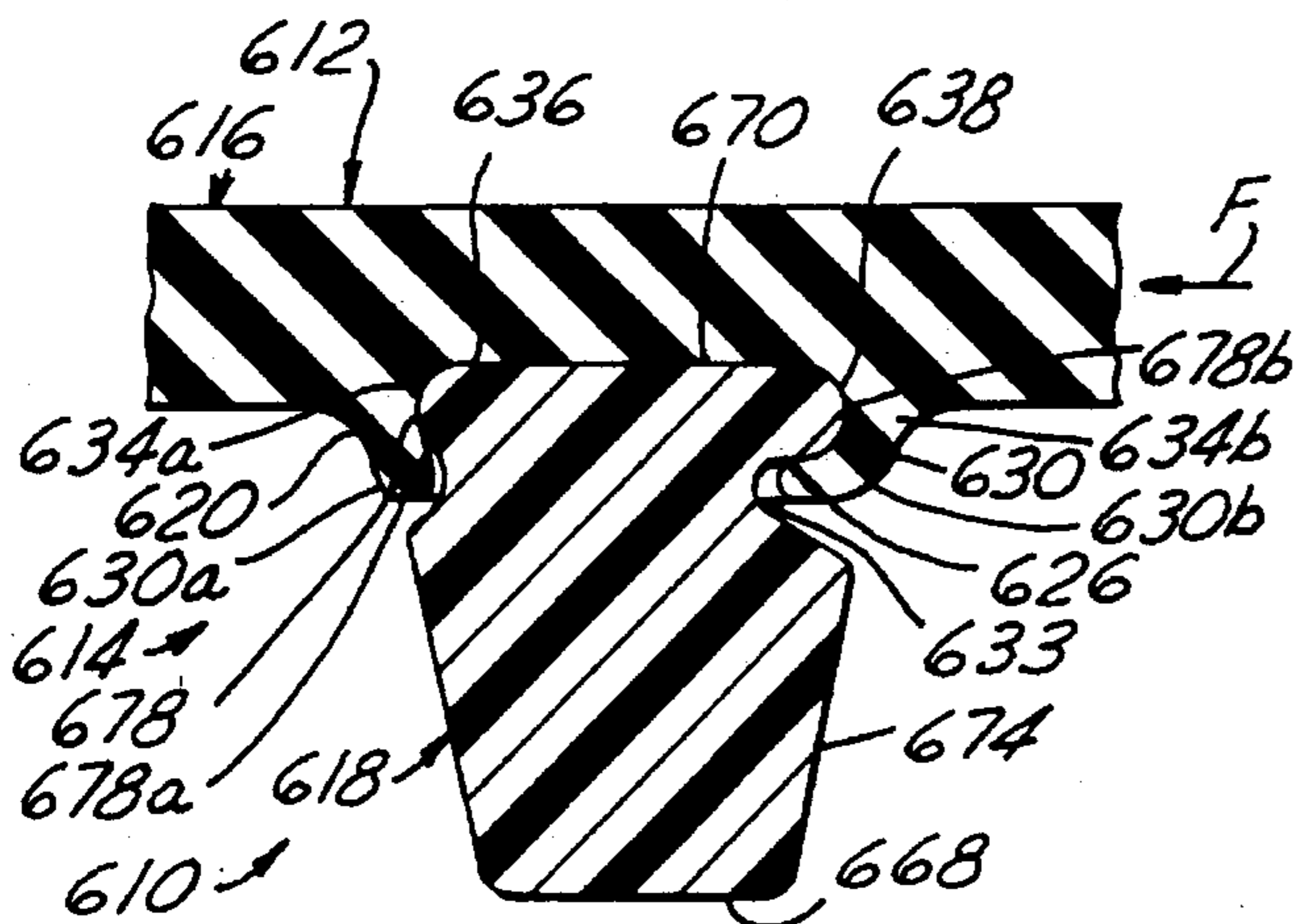
FIG. 32
