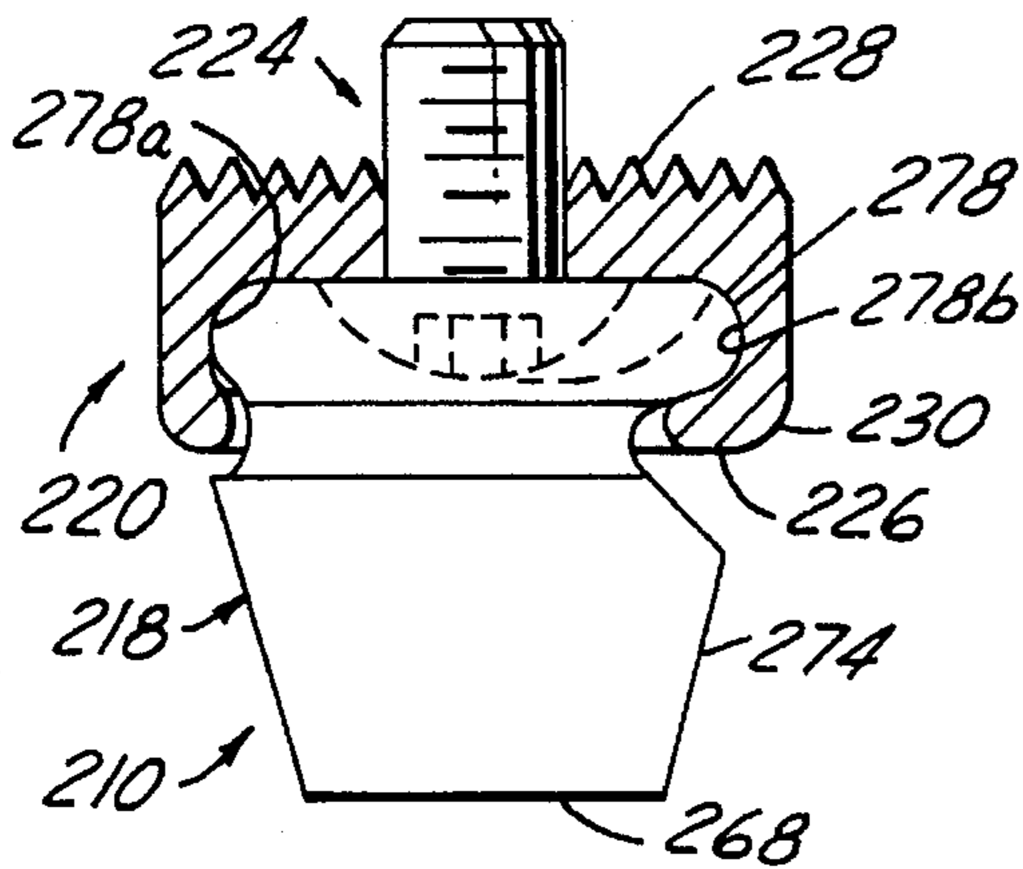
FIG. 19
