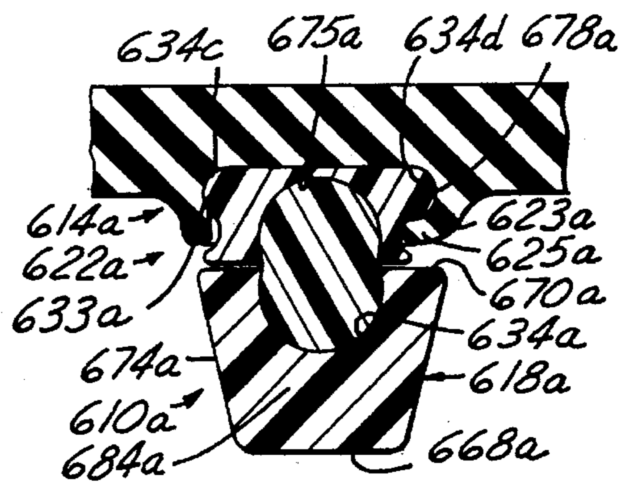
FIG. 32a
