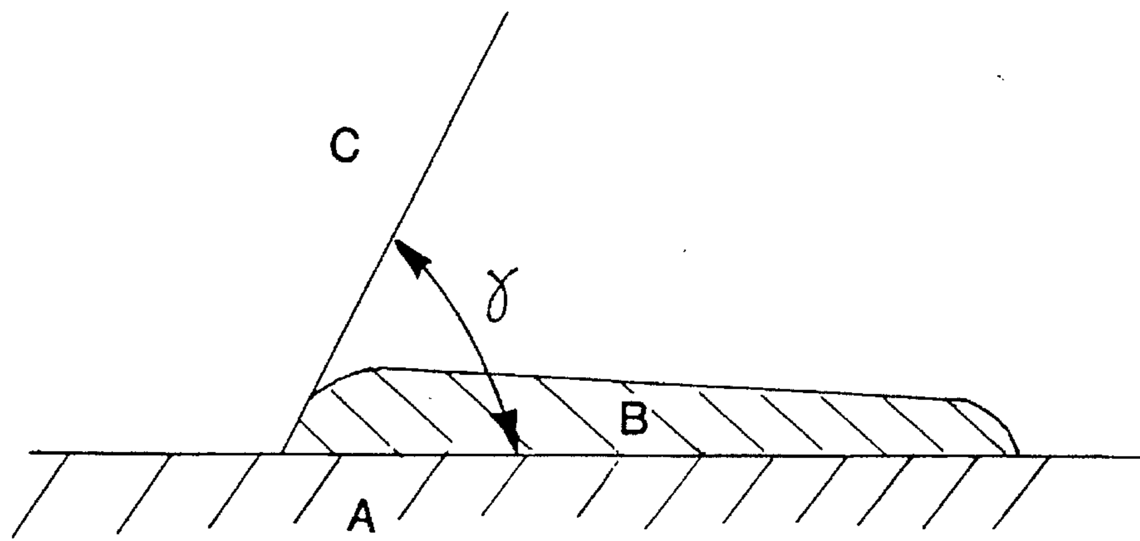
FIG. 1 SESSILE DROP
