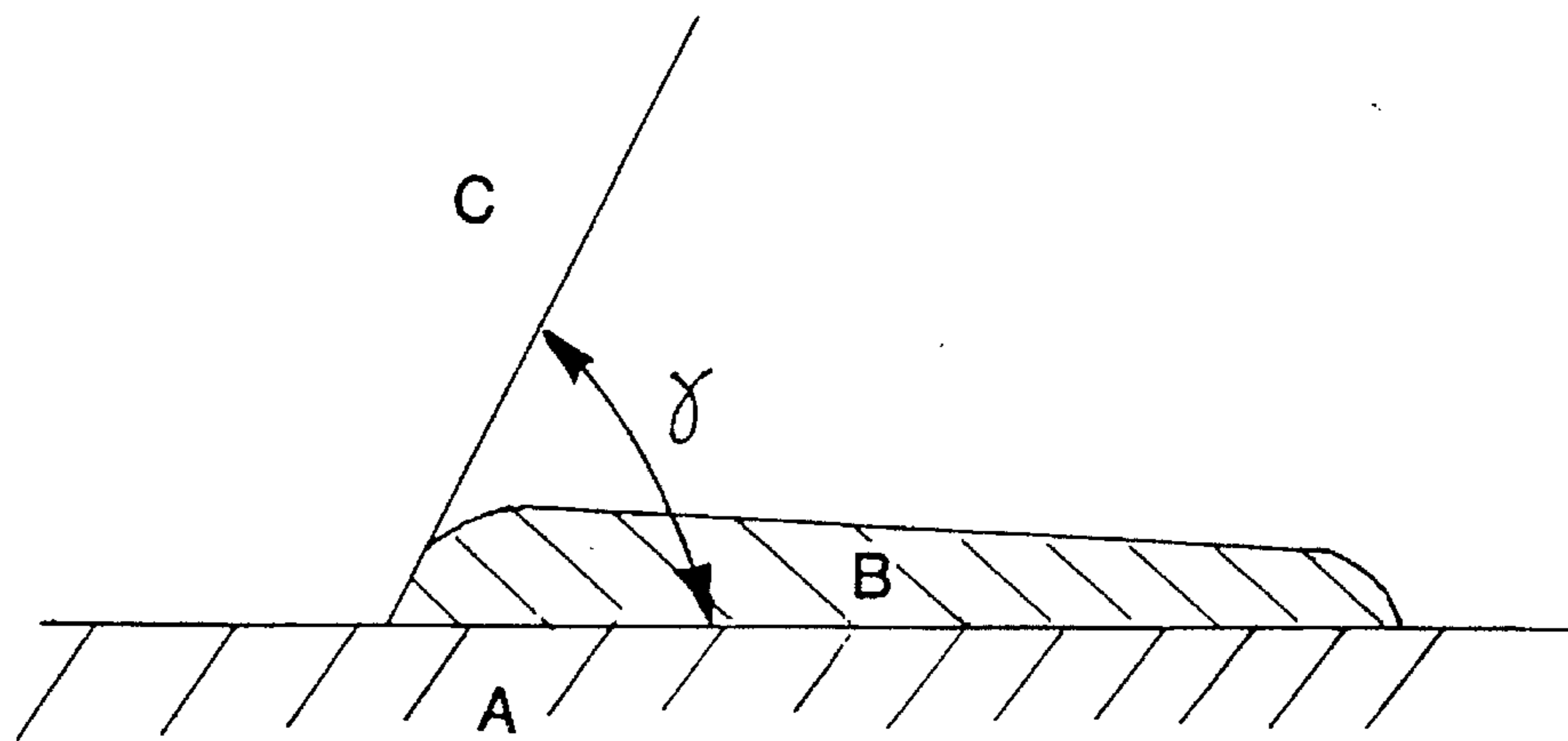
FIG. 1 SESSILE DROP
