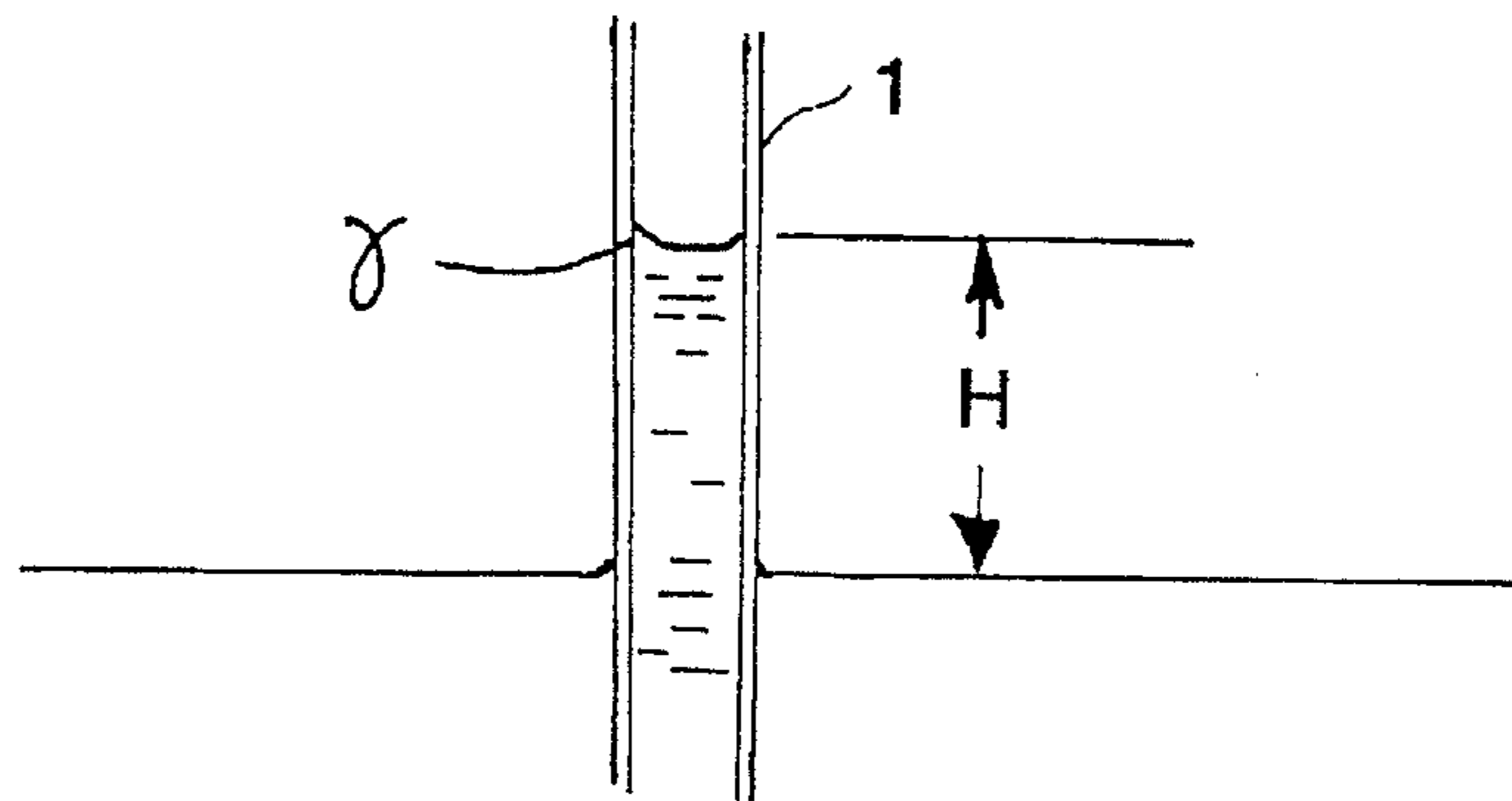
FIG. 2 CAPILLARY RISE
