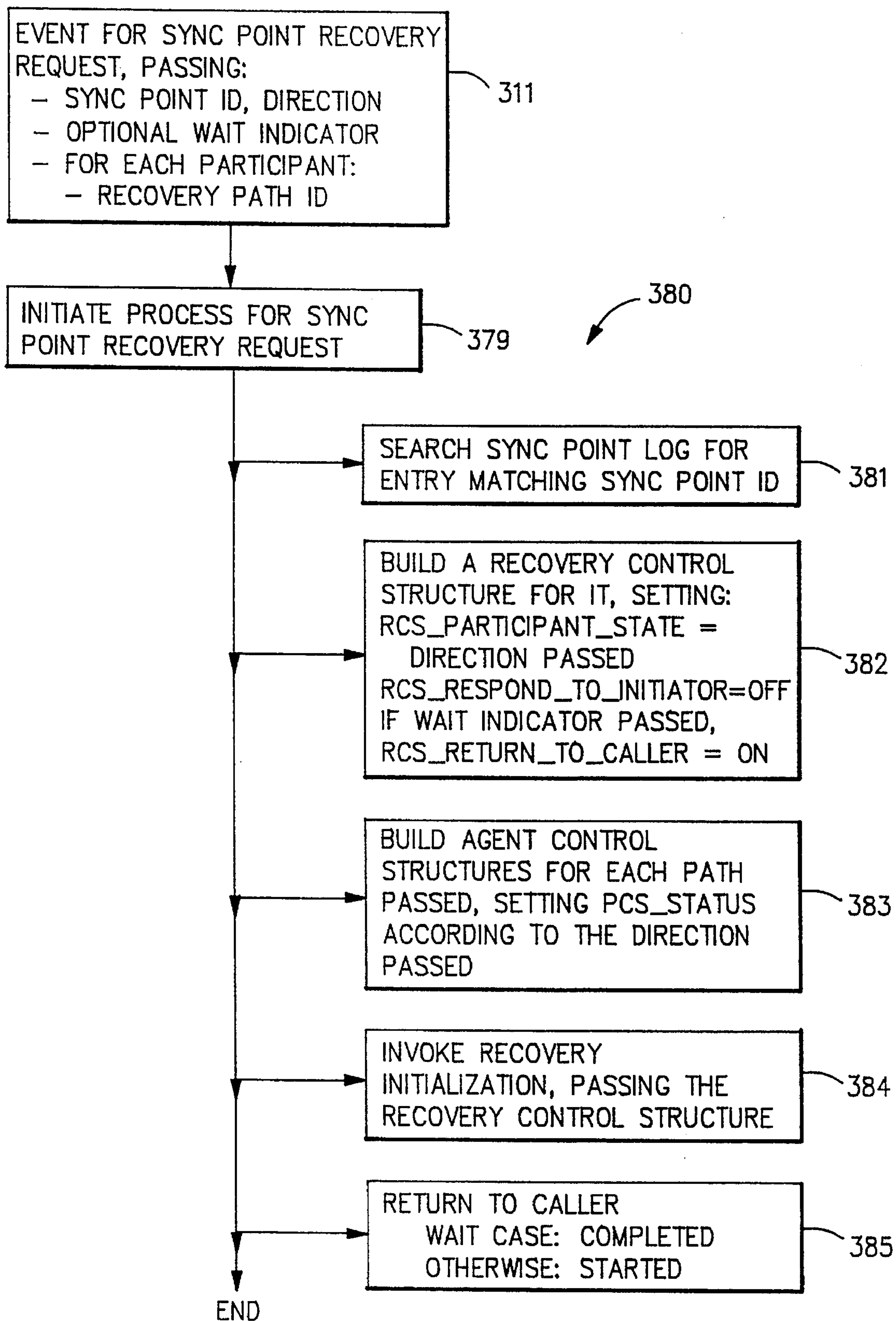
FIG. 40
