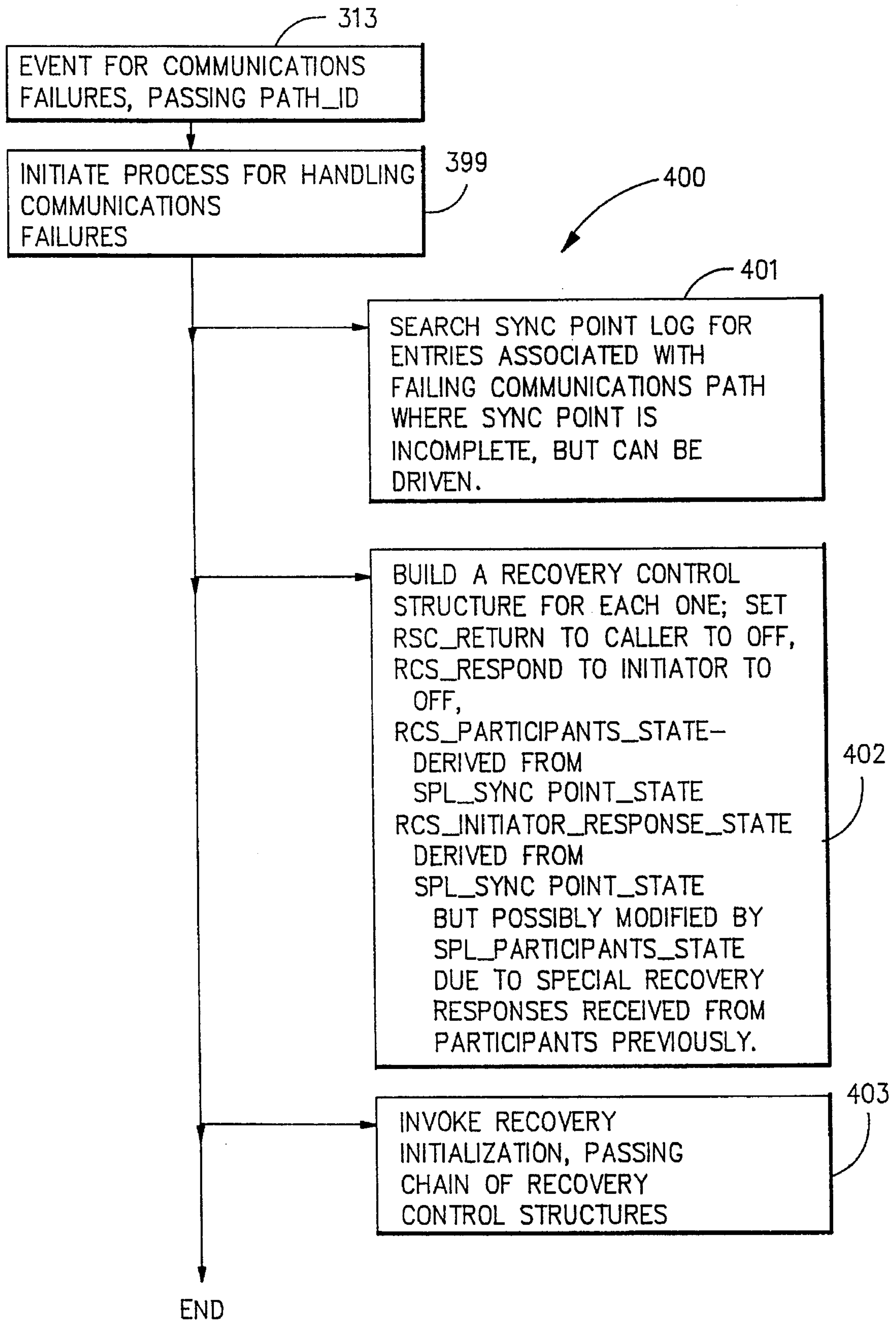
FIG.42
