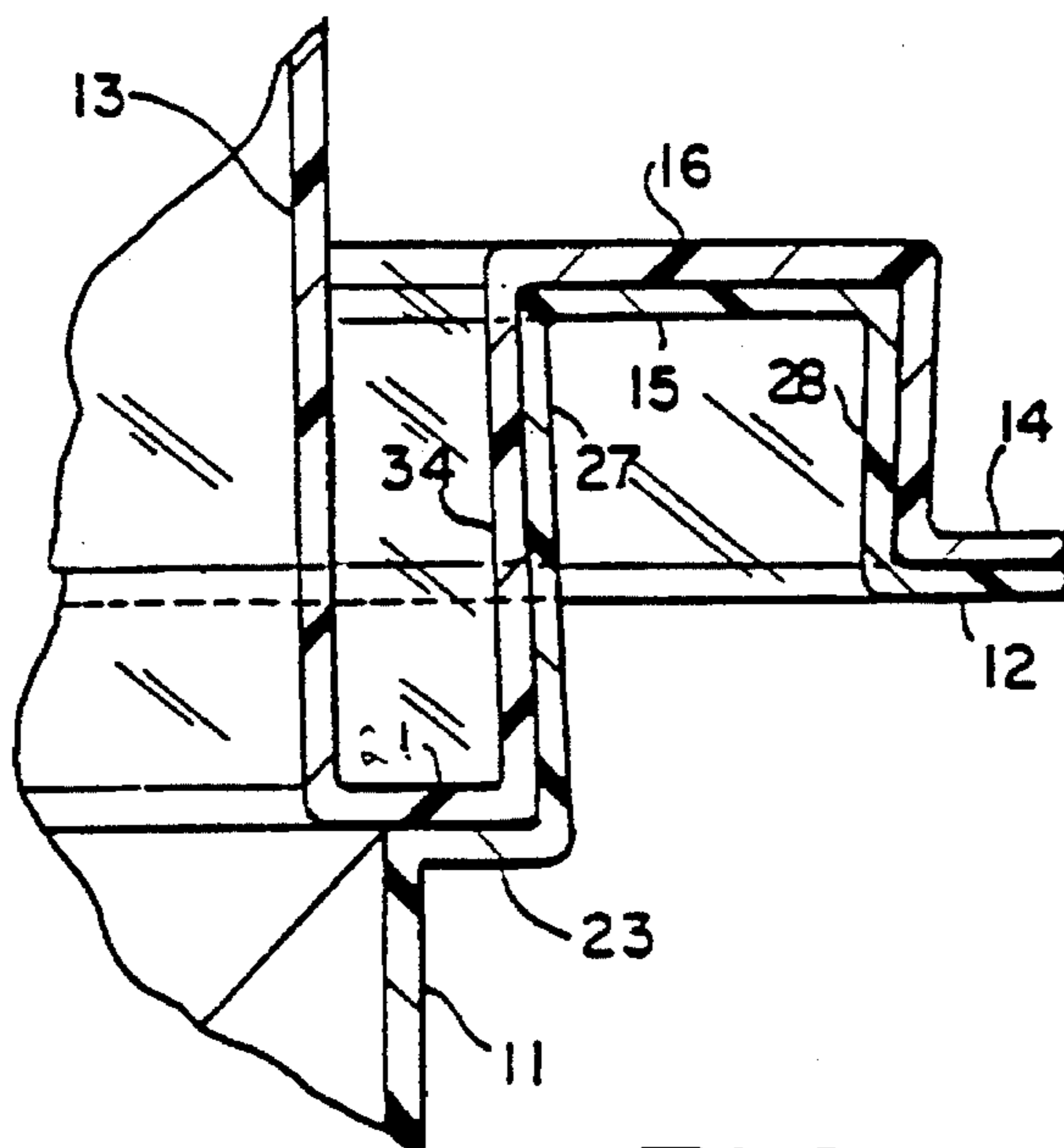
FIG. 8 (ENLARGED DETAIL)
