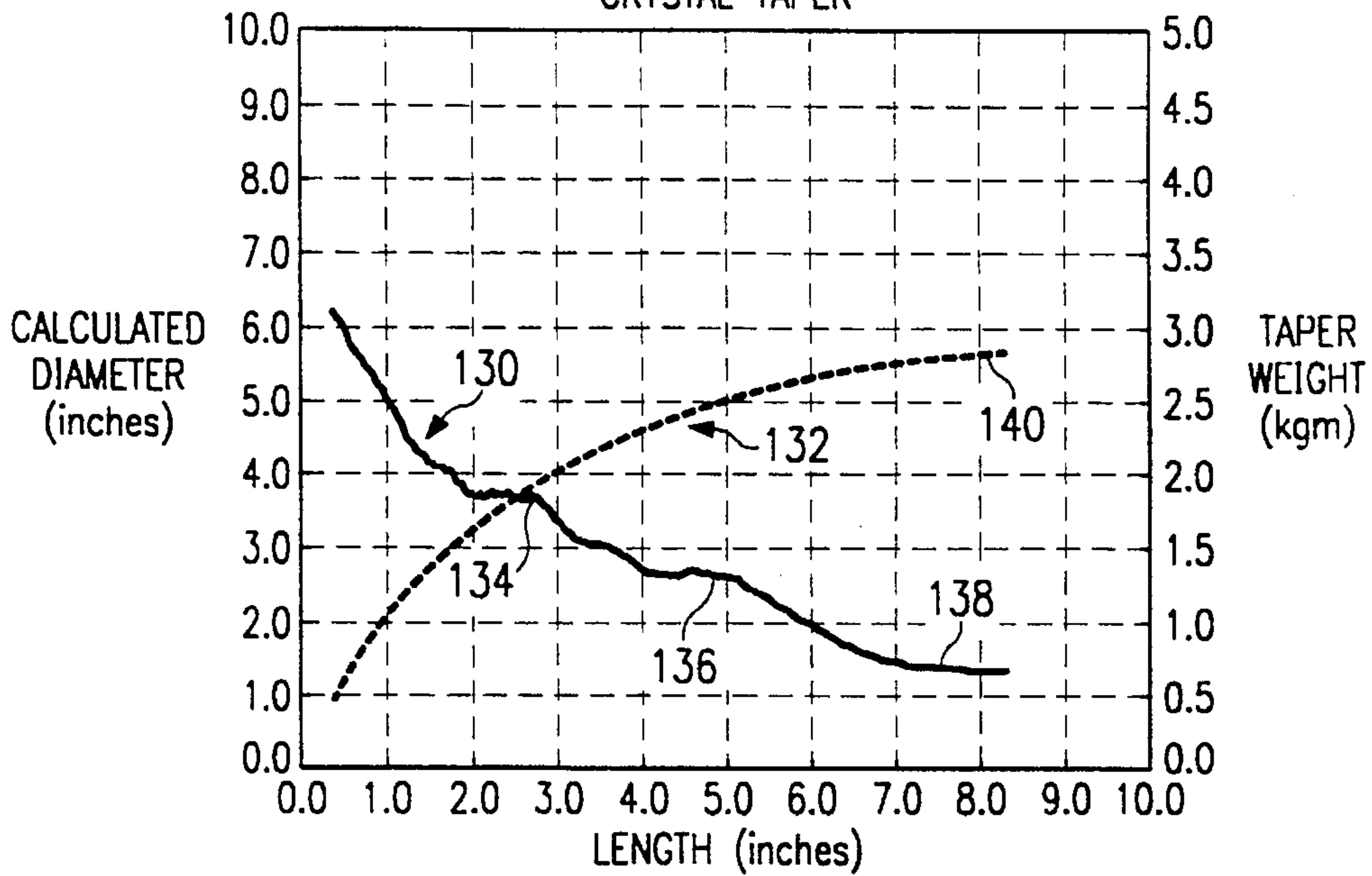
FIG. 5 CRYSTAL TAPER
