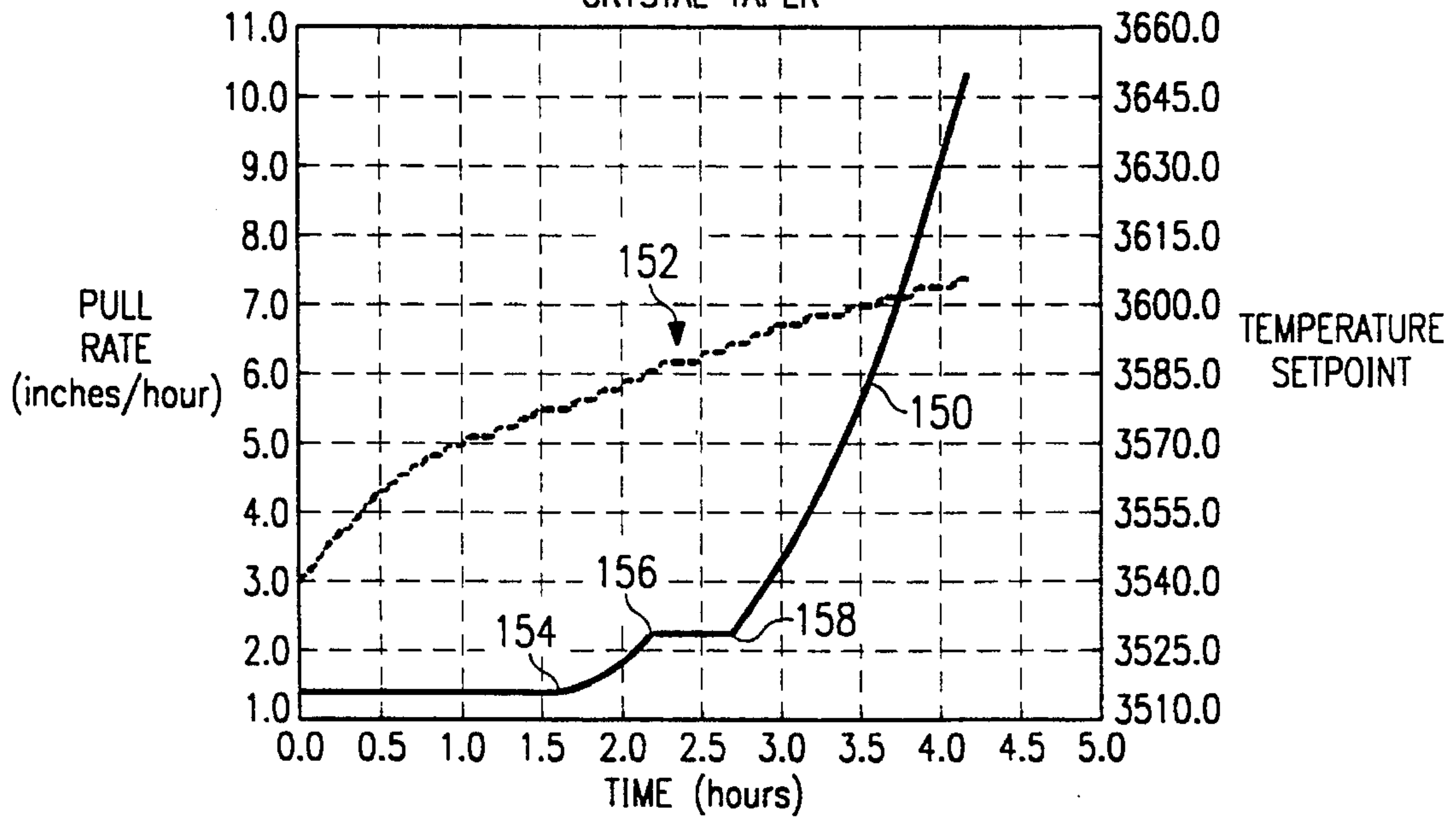
FIG. 6 CRYSTAL TAPER
