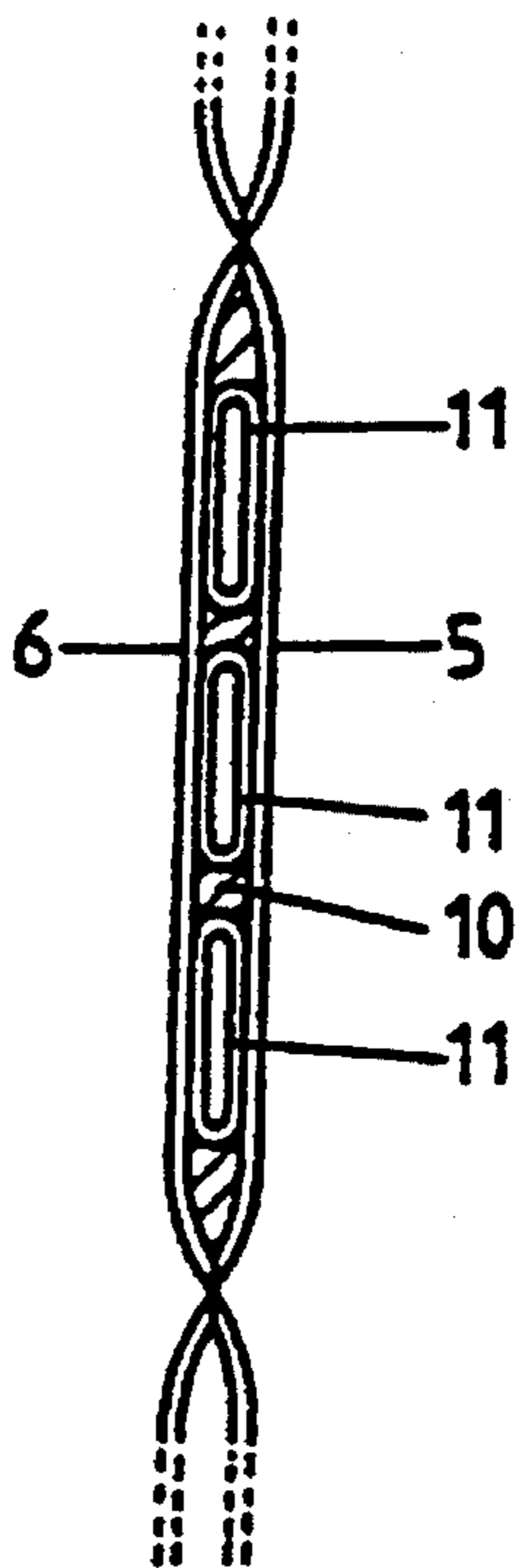
FIG 4 (VIEW A-A)
