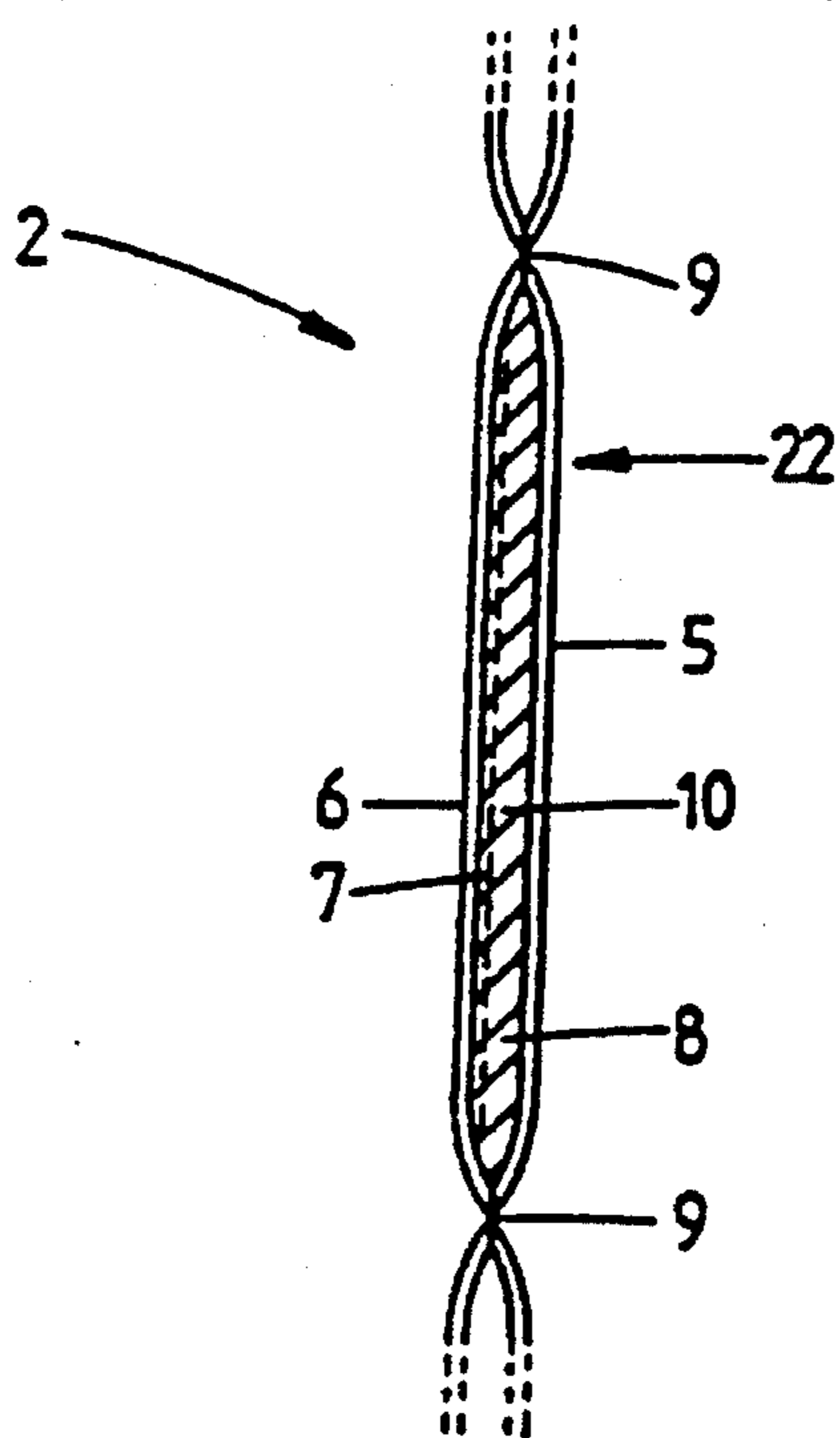
FIG 2 (VIEW A-A)
