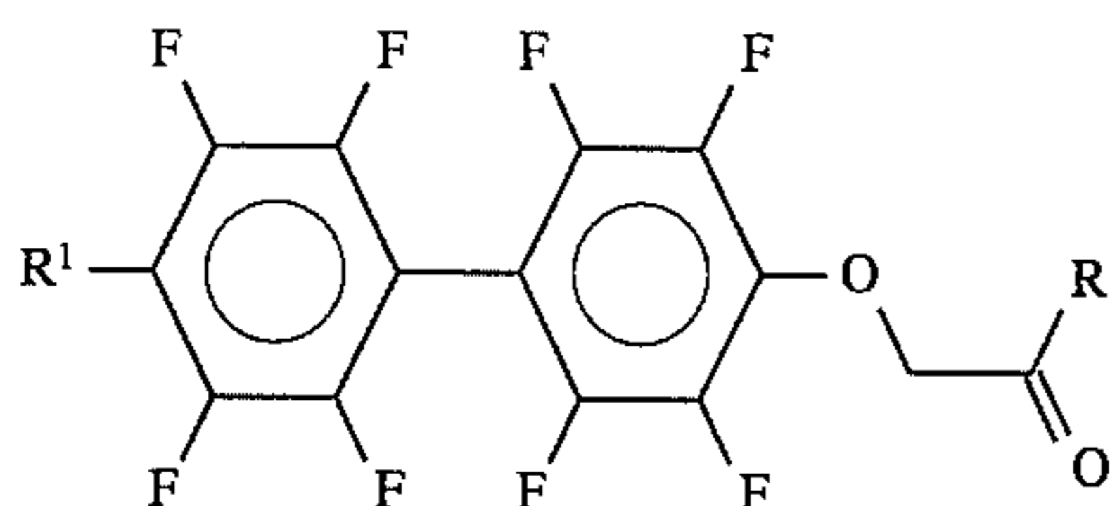
Ketones 73
