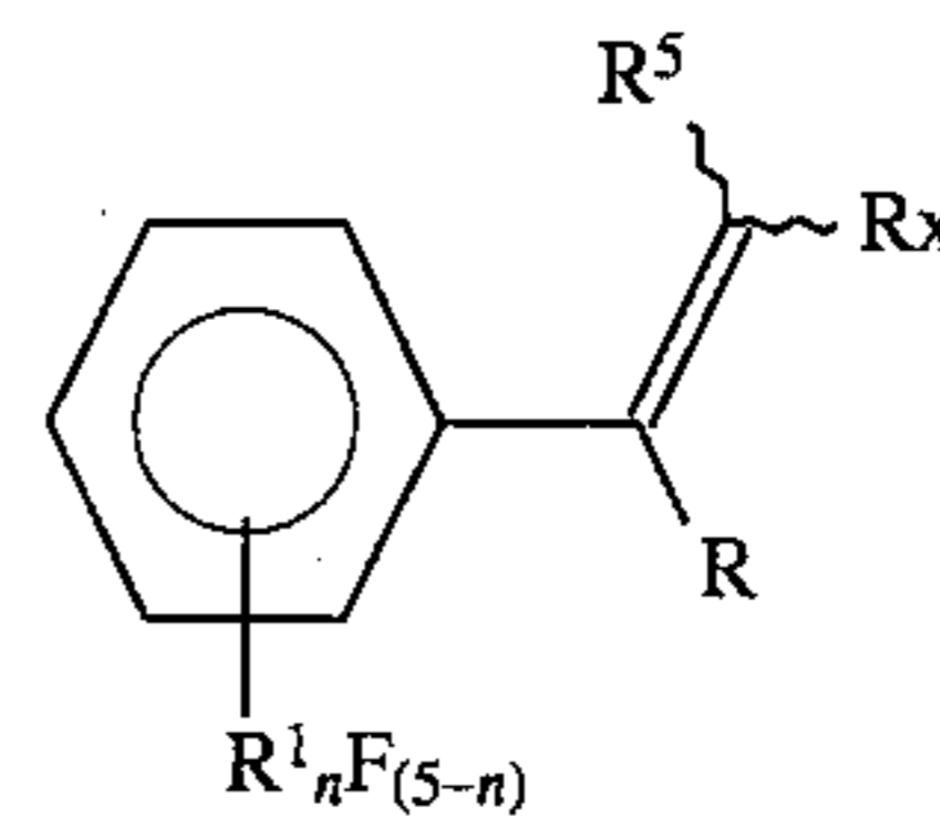
Olefins 70
