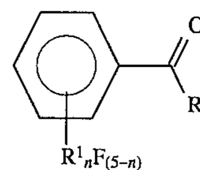
Ketones 69
