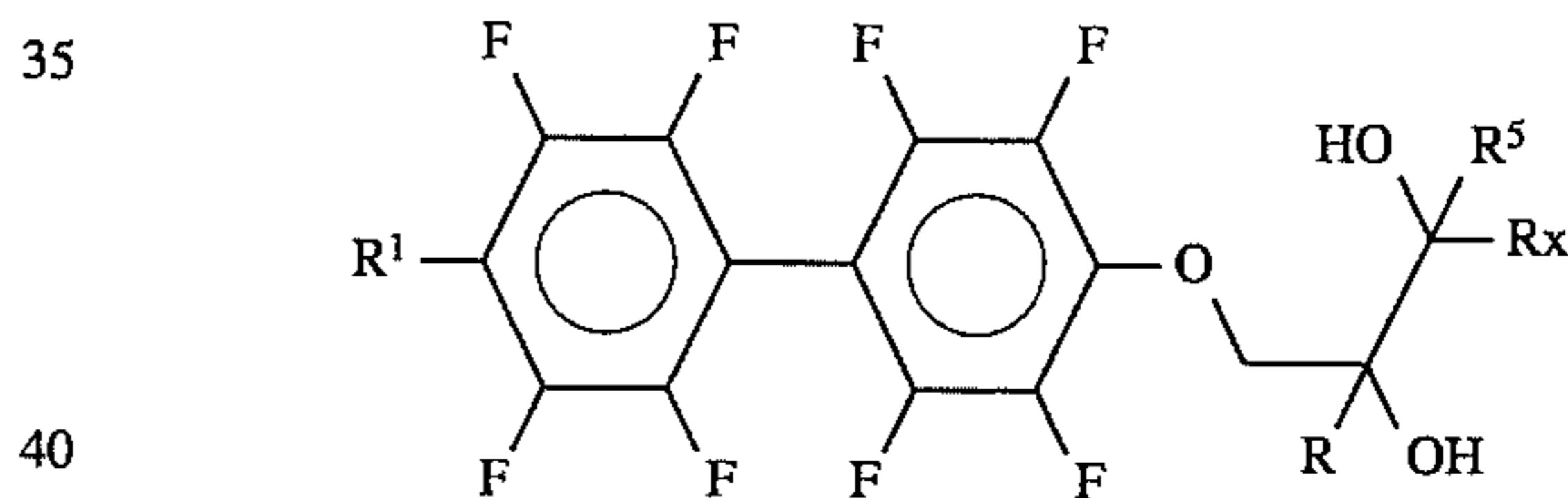
Glycols 75
