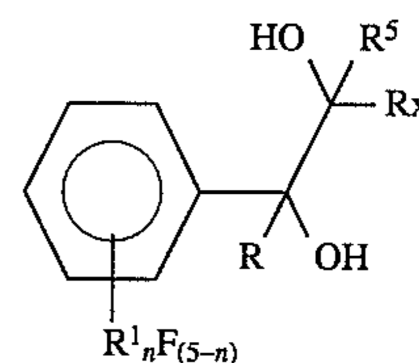
Glycols 71
