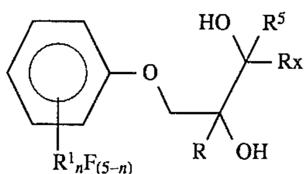
Glycols 67
