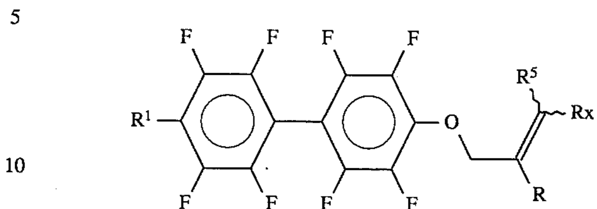
Olefins 74
