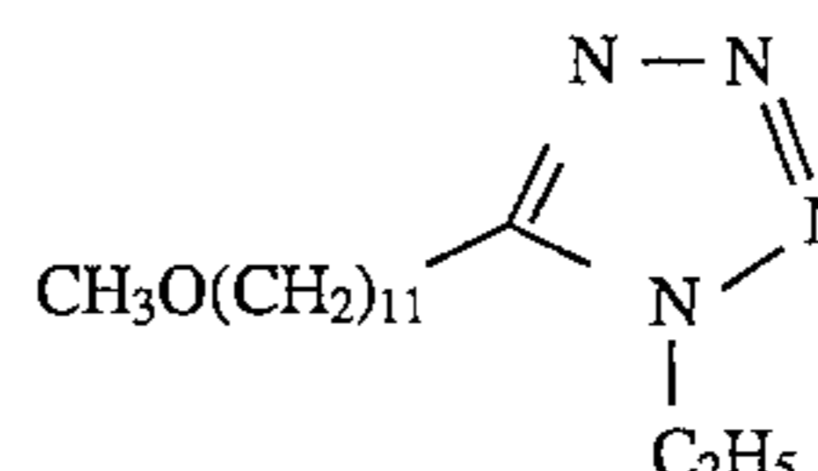
A. 1-Ethyl-5-(11-methoxyundecyl)-1H-tetrazole
