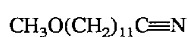
12-Methoxydodecanenitrile
