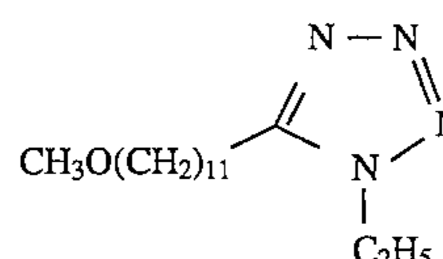
A. 1-Ethyl-5-(11-methoxyundecyl)-1H-tetrazole
