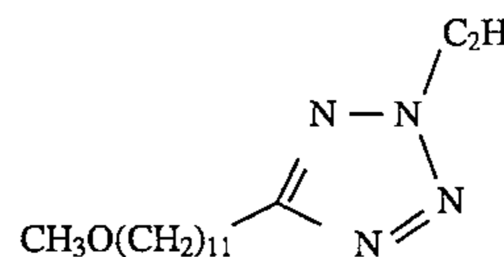
A. 1-Ethyl-5-(11-methoxyundecyl)-1H-tetrazole
