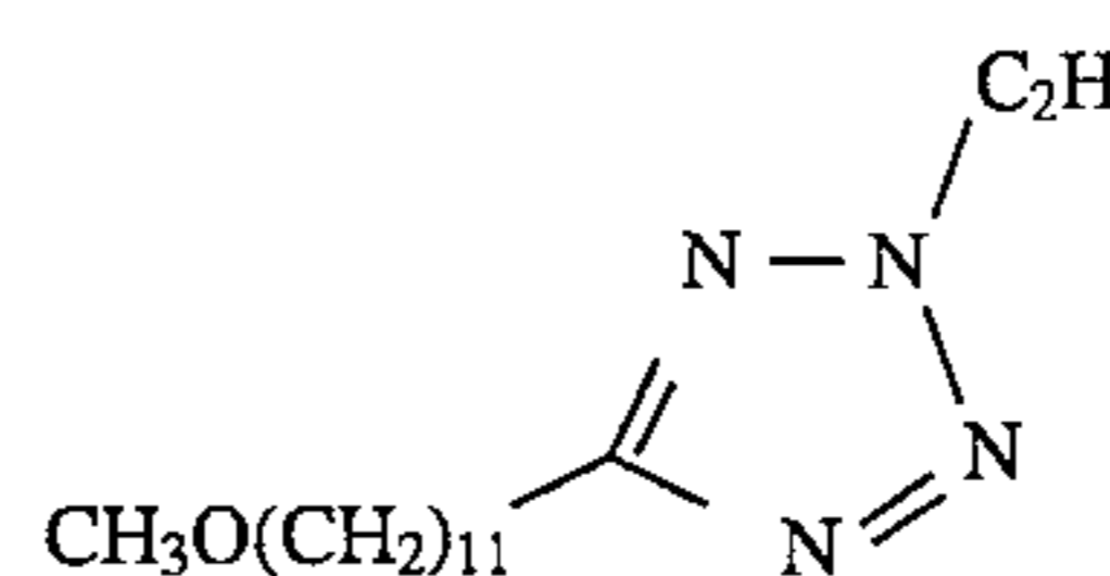
A. 1-Ethyl-5-(11-methoxyundecyl)-1H-tetrazole
