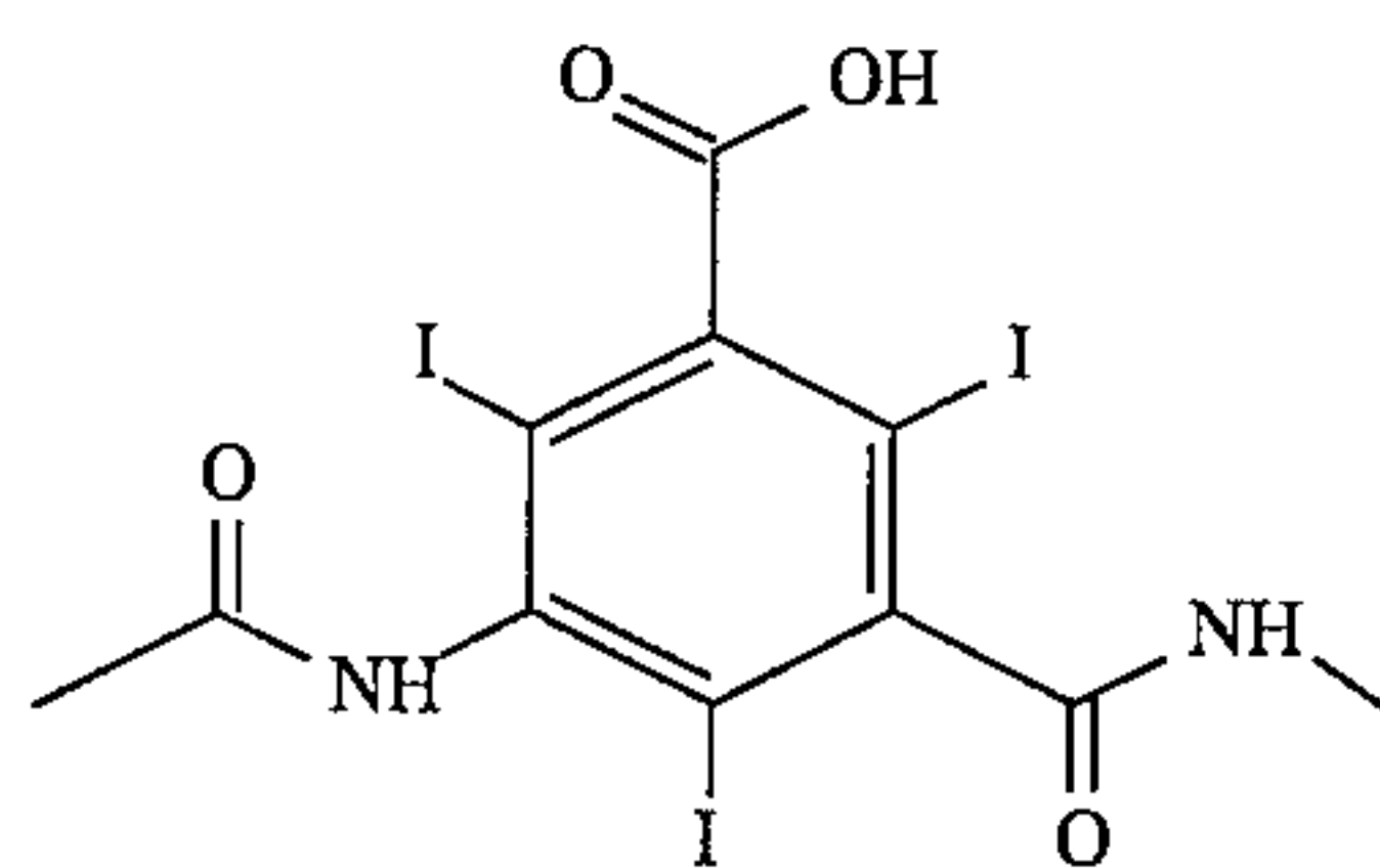
Meglumine Salt
