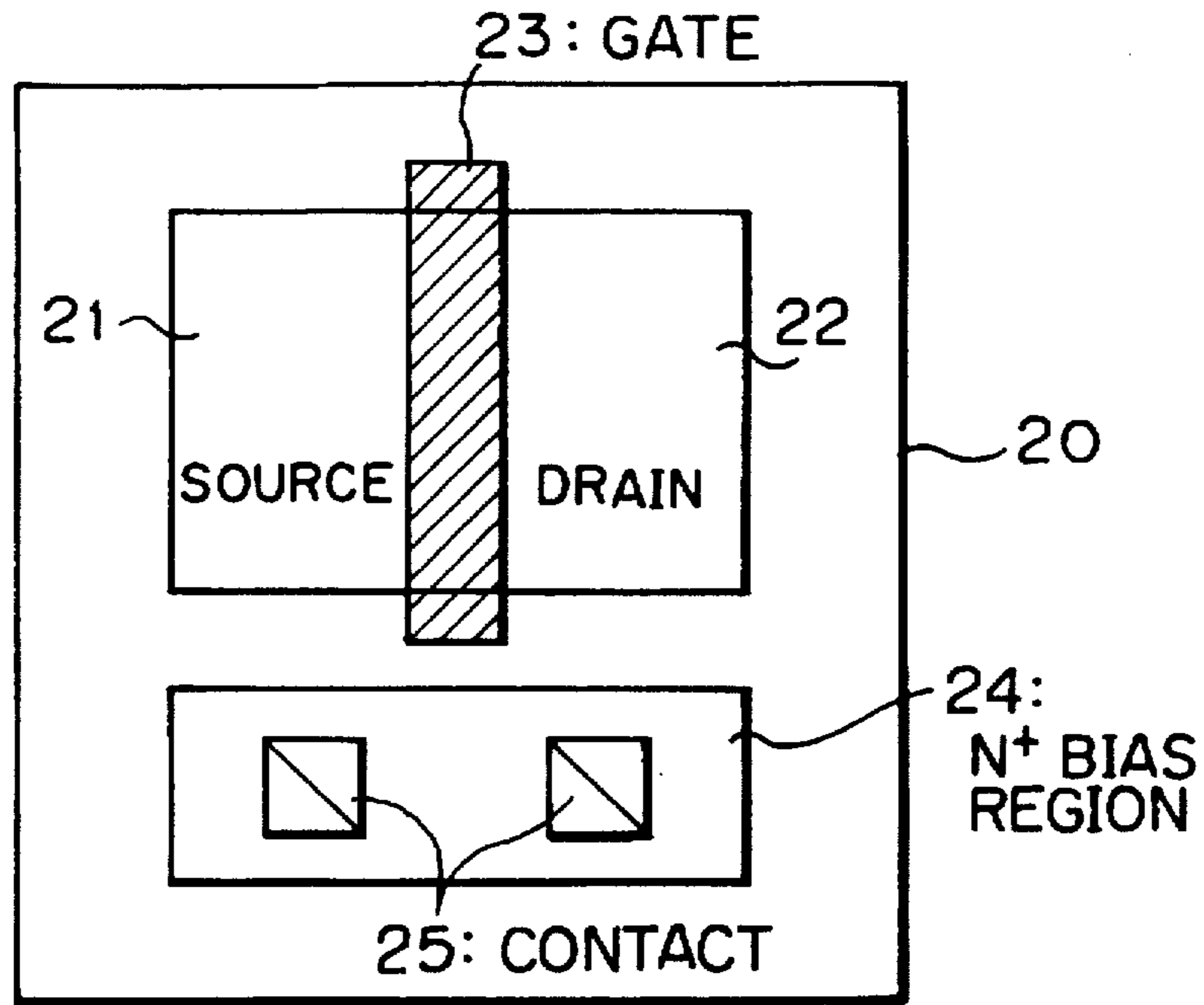
BULK MOSFET
