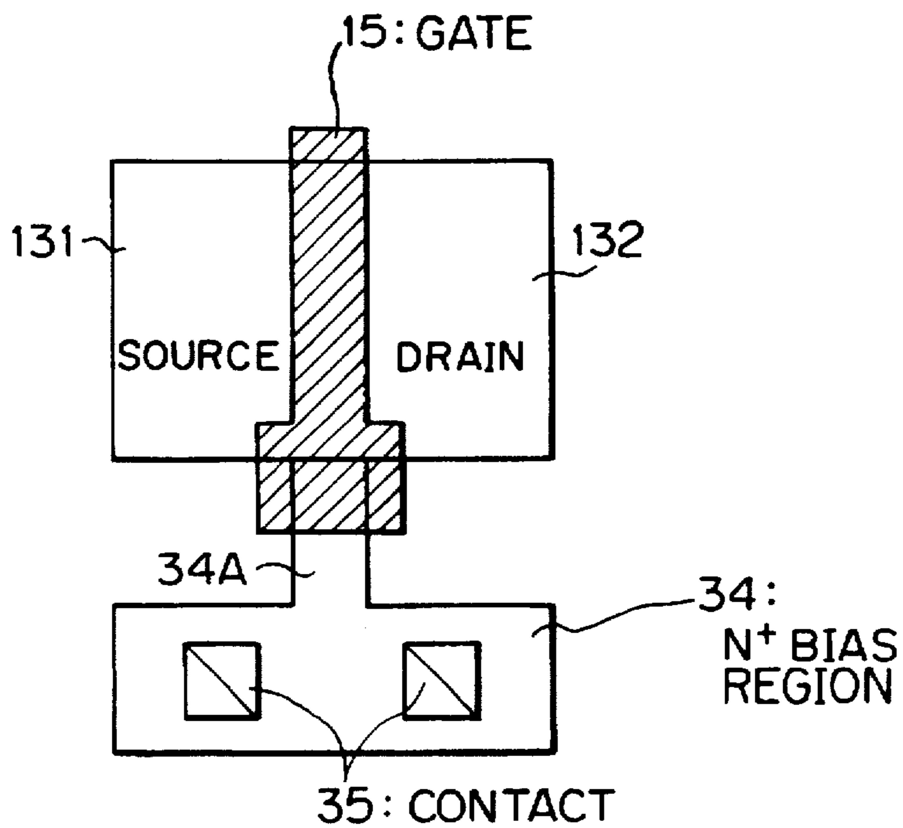
SOI MOSFET
