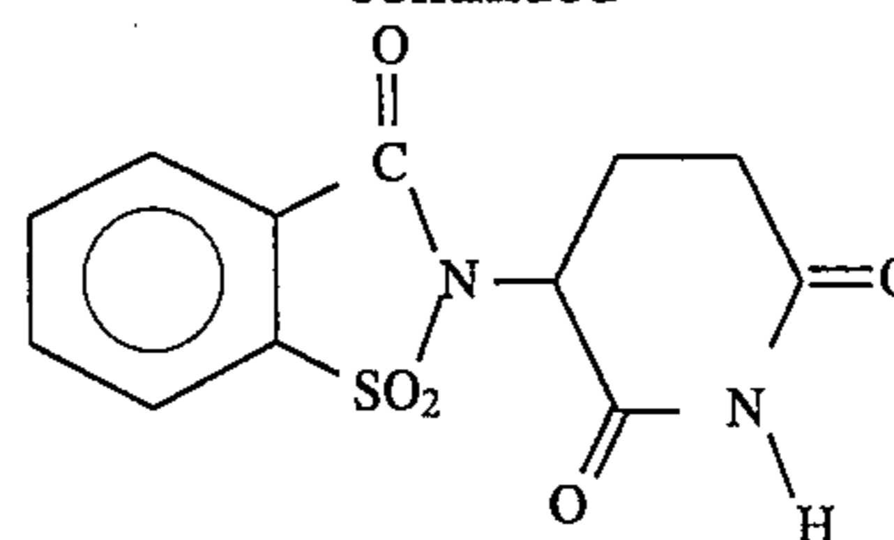
supidimide.
