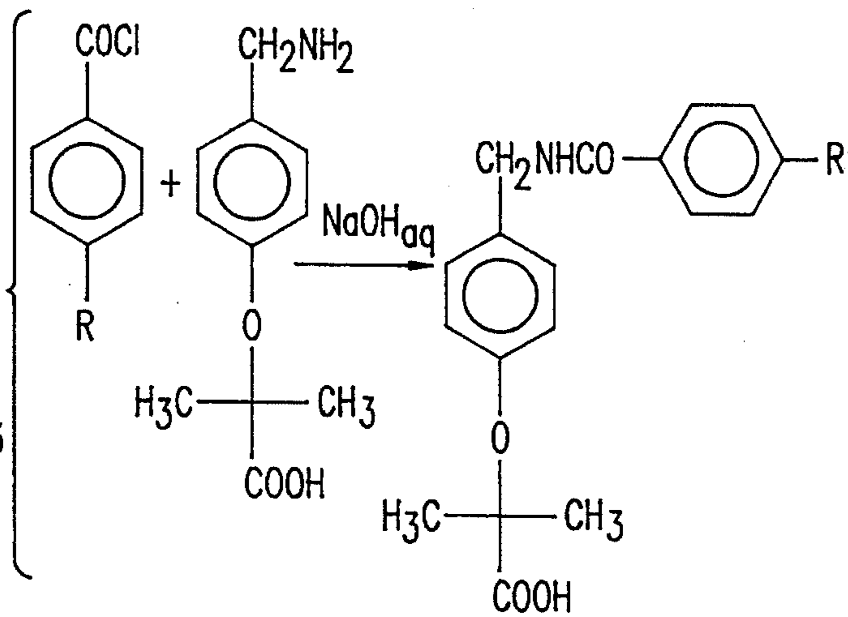
FIG. 7B
