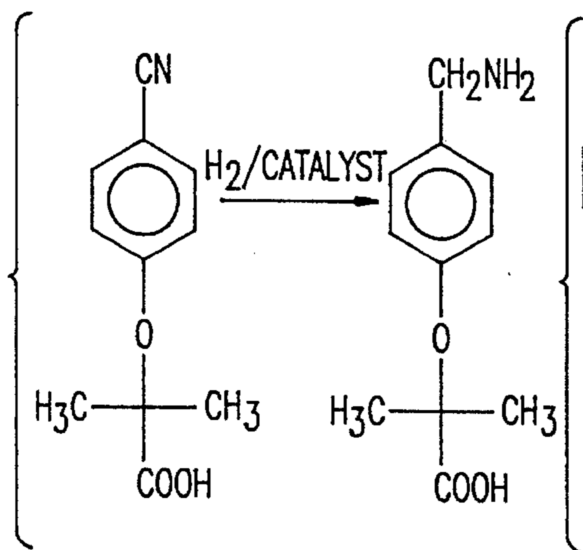
FIG. 7A
