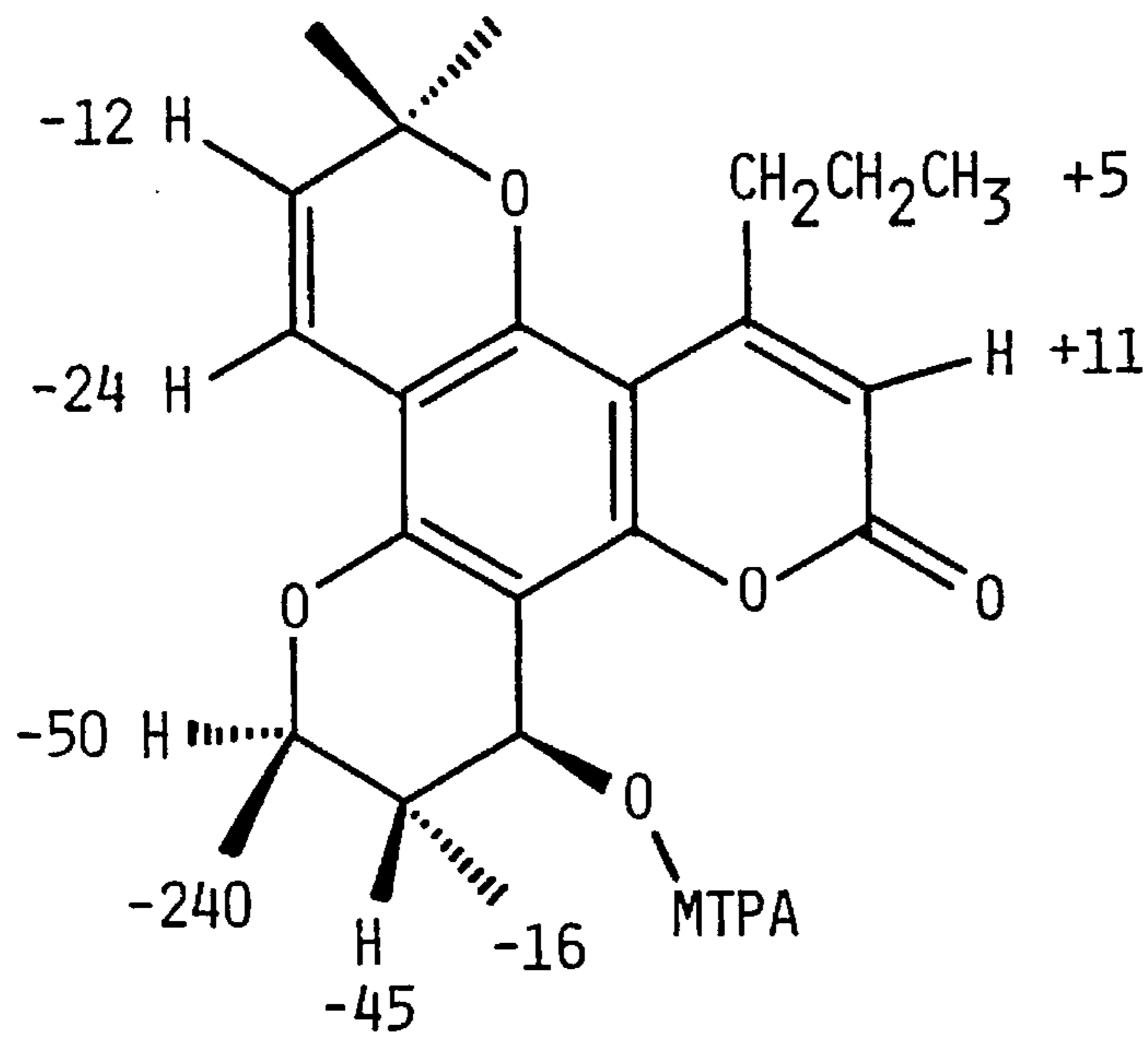
Calanolide A- MTPA ester
