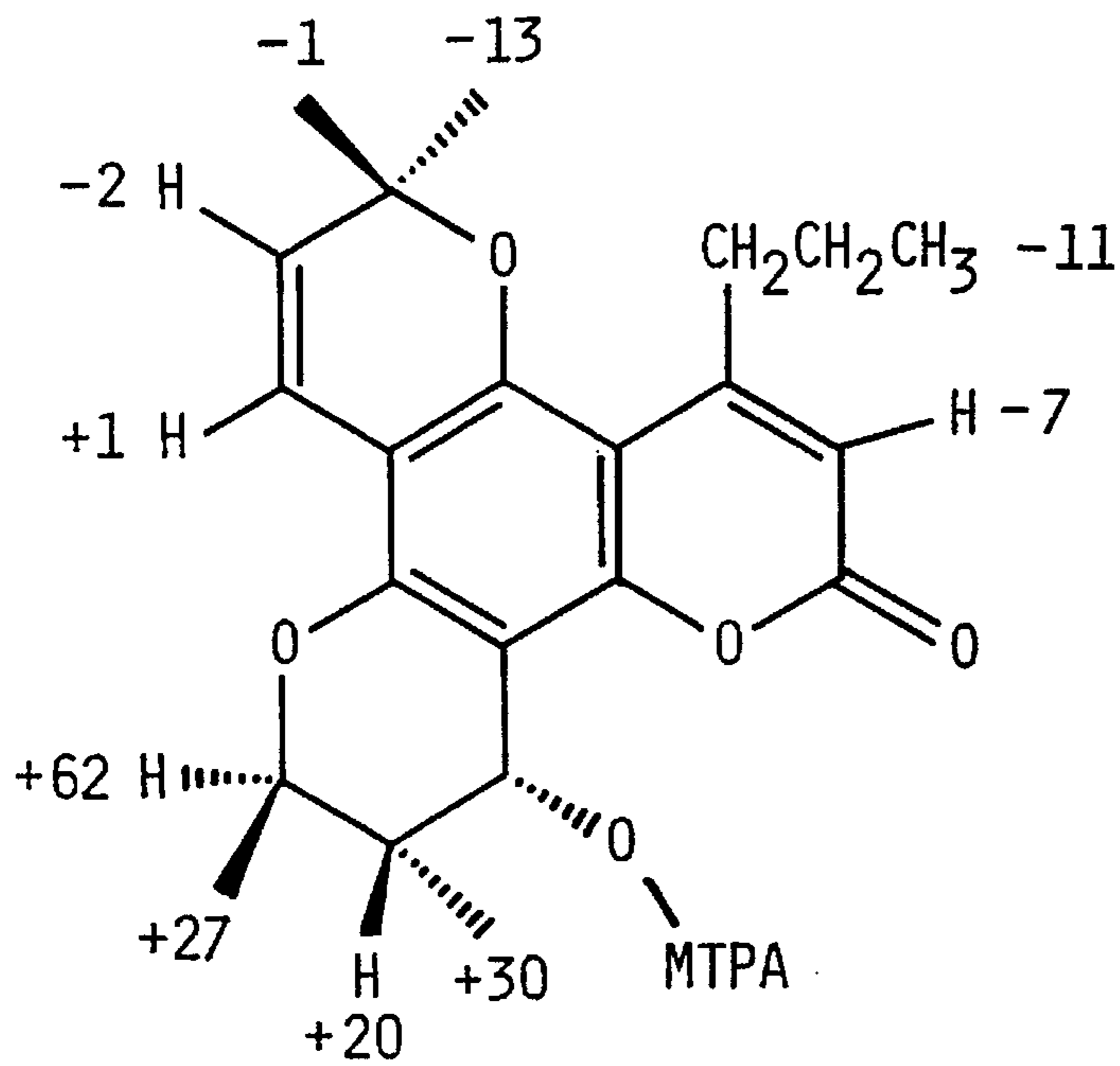
Calanolide B - MTPA ester
