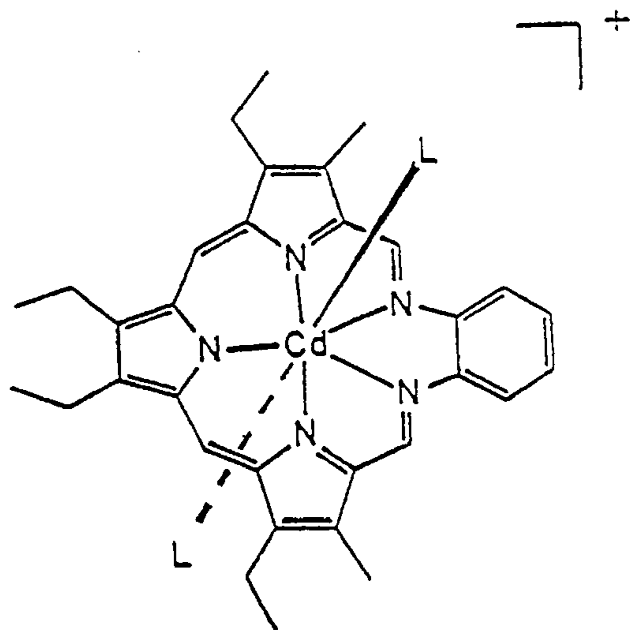
5aA. L = pyr 5bA. L = BzIm
