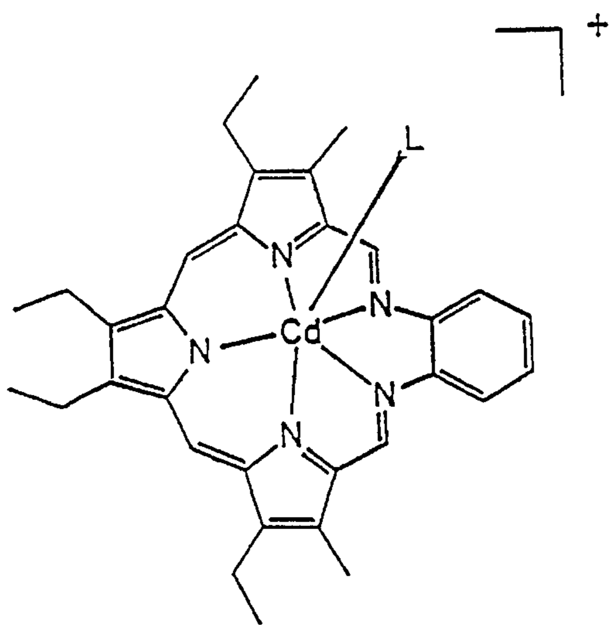
4aA. L = pyr 4bA. L = BzIm
