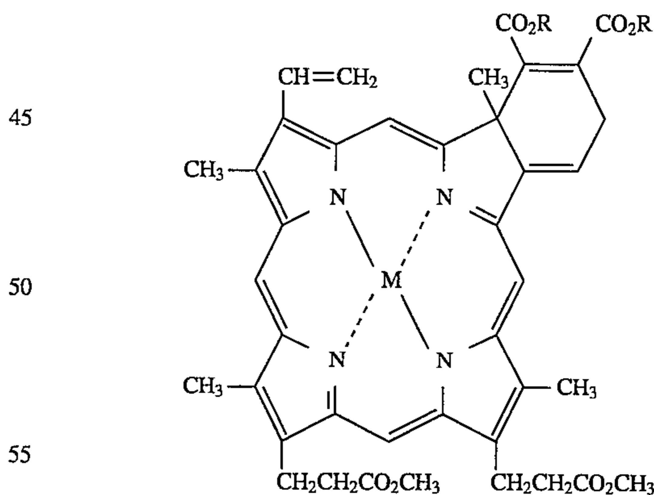
Complex VI
