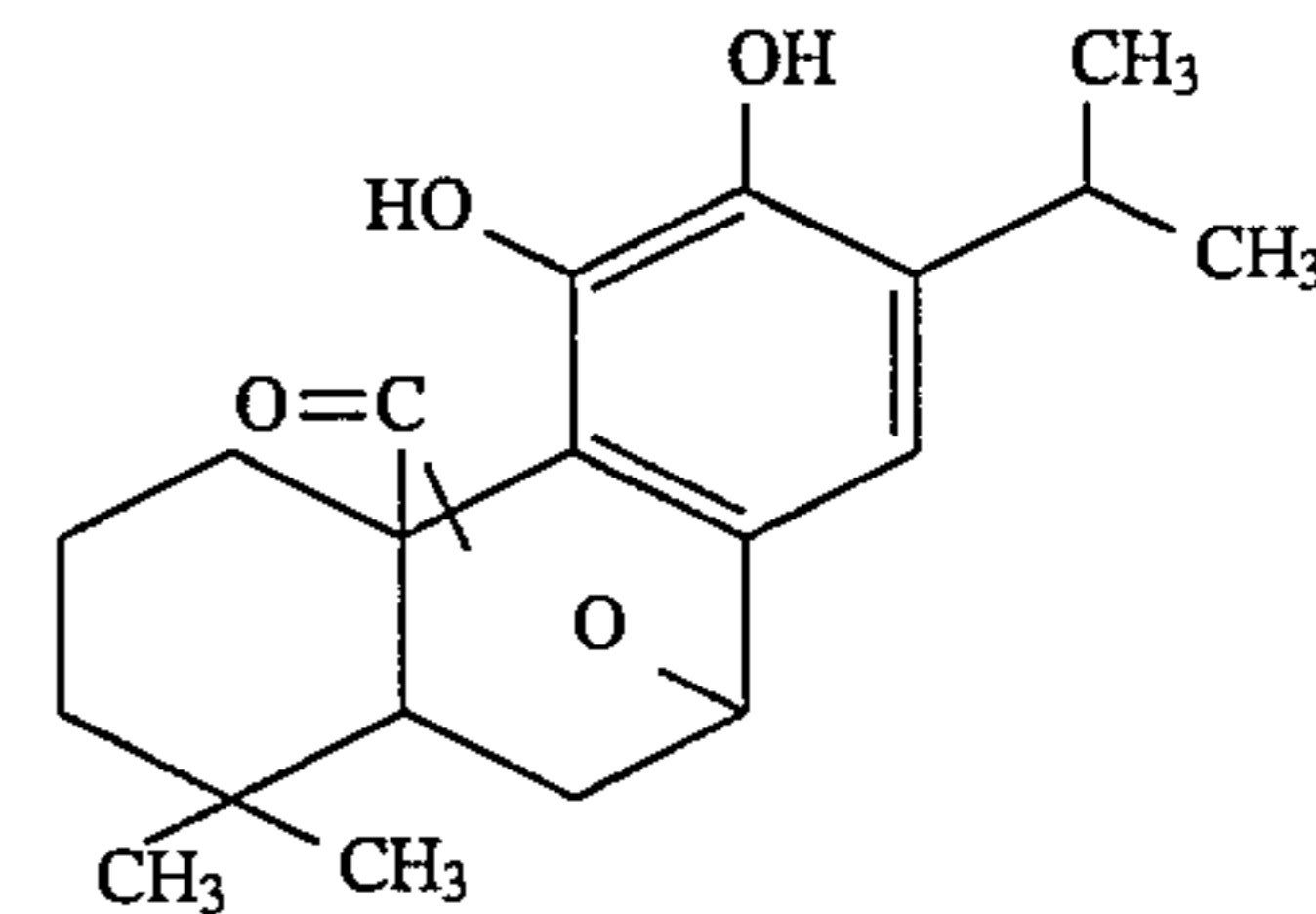
Carnosol
