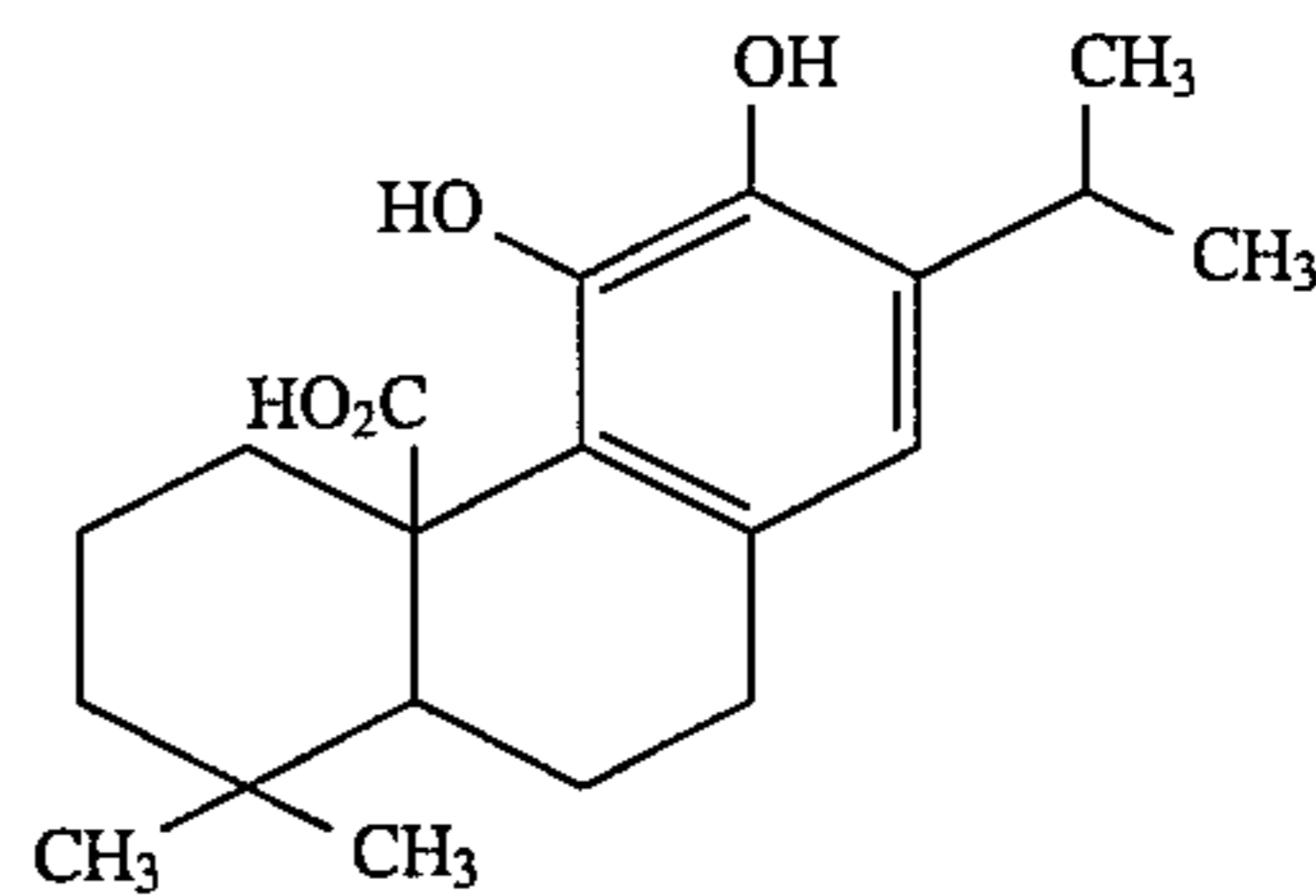
Carnosic acid
