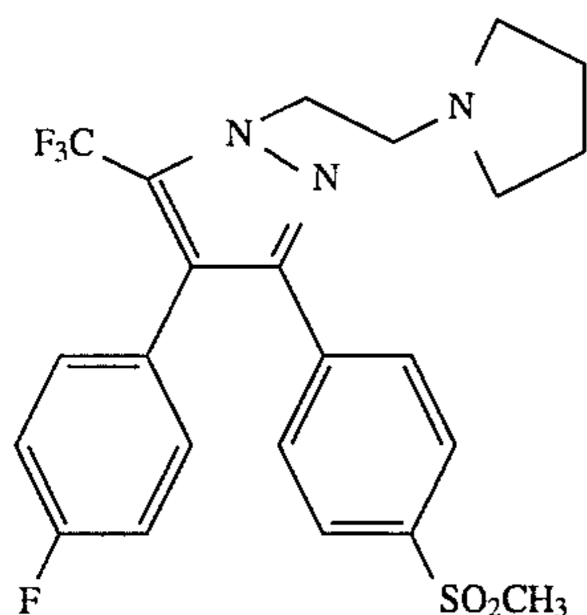
4-(4-Fluorophenyl)-3-[4-(methylsulfonyl)phenyl]-1-[2-(1H-pyrrolidin-1-yl)ethyl]-5-(trifluoromethyl)-1H-pyrazole
