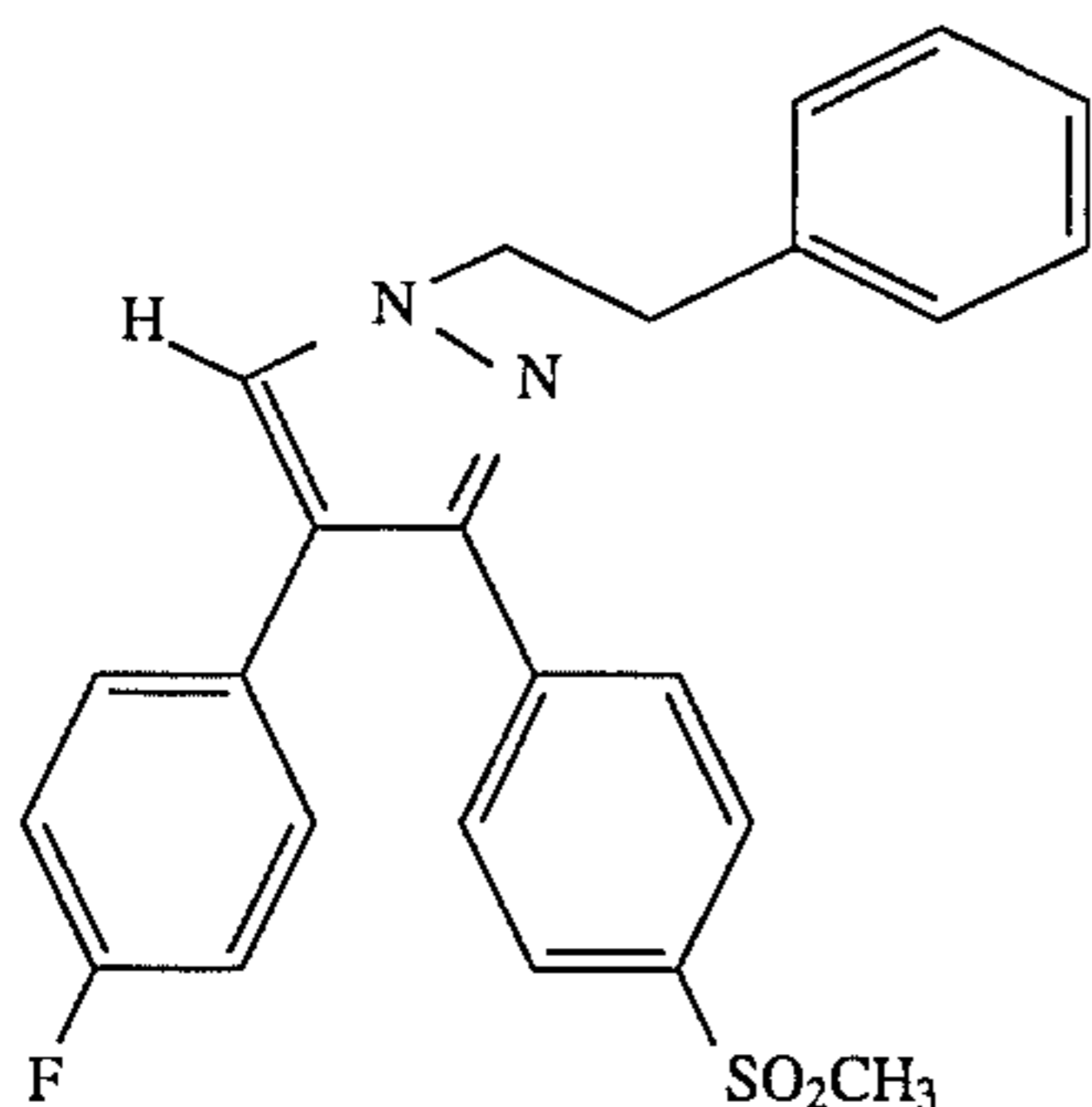
4-(4-Fluorophenyl)-3-[4-(methylsulfonyl)phenyl]-1-(2-phenylethyl)-1H-pyrazole
