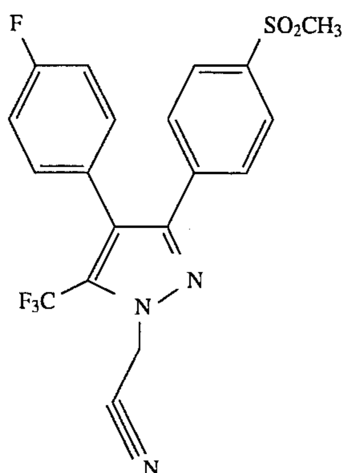
1-Cyanomethyl-4-(4-fluorophenyl)-3-[4-(methylsulfonyl)phenyl]-5-(trifluoromethyl)-1H-pyrazole
