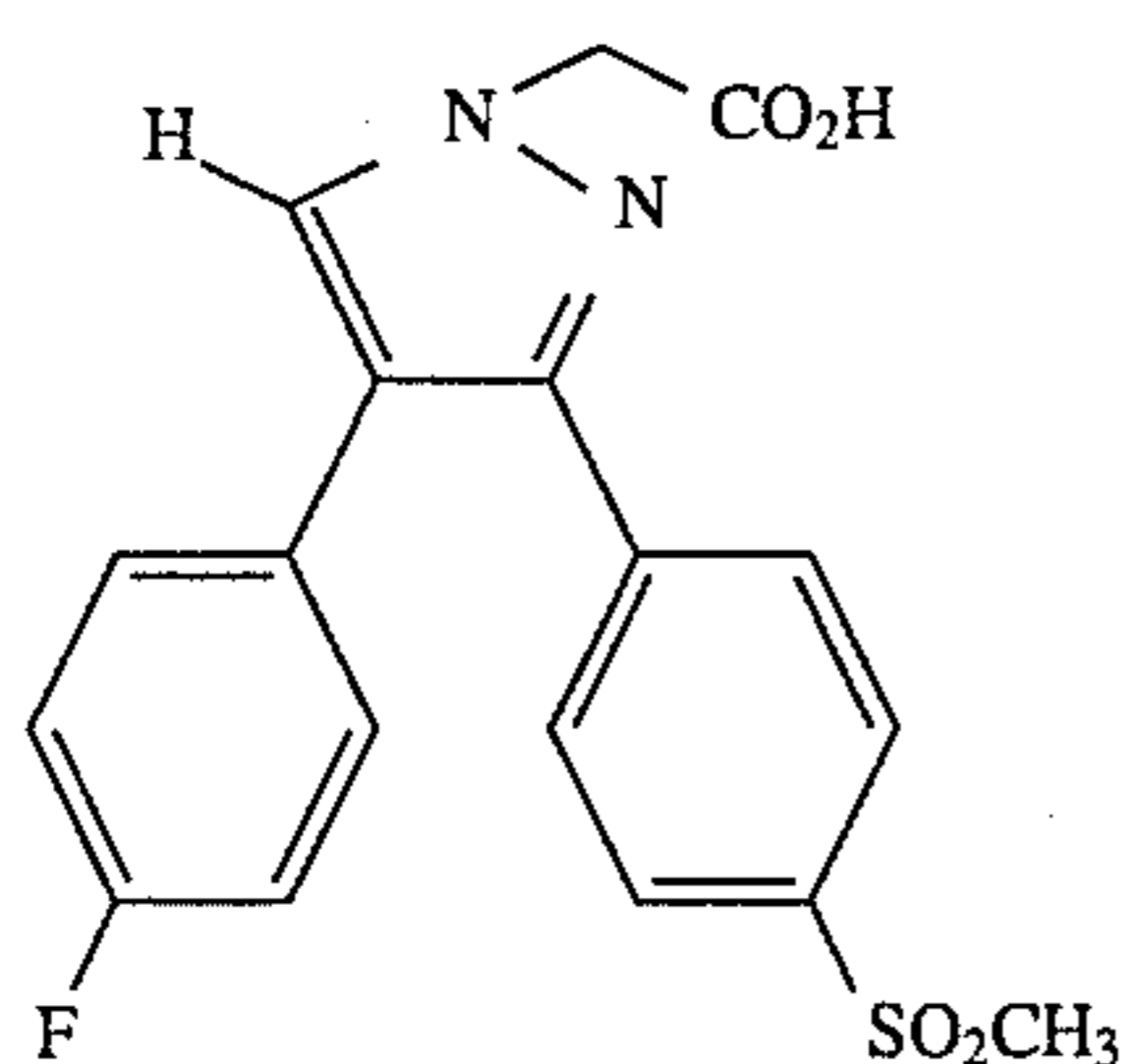
4-(4-Fluorophenyl)-3-[4-(methylsulfonyl)phenyl]-1H-pyrazol-1-yl]acetic acid
