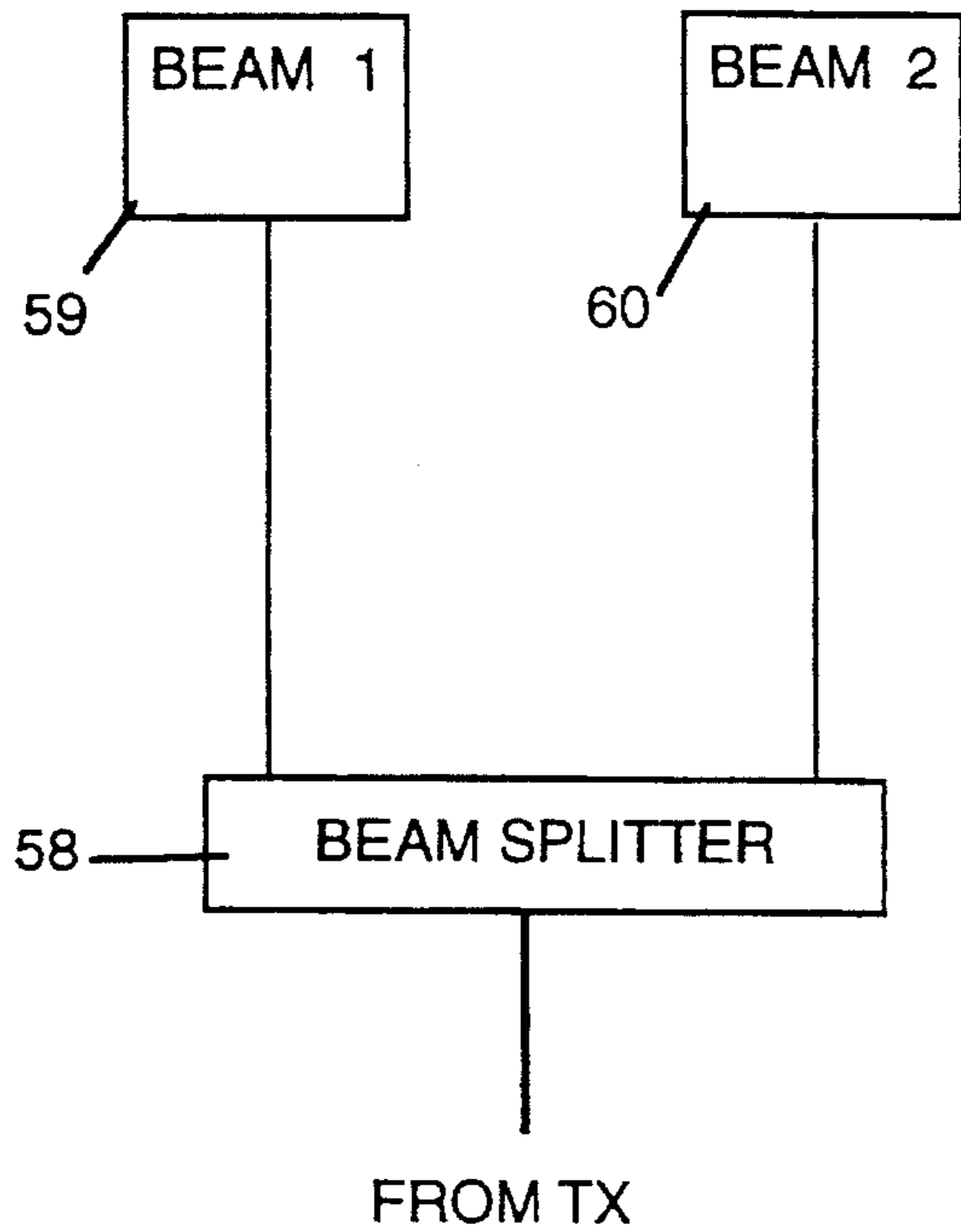
Fig. 14 (a) INPHASE
