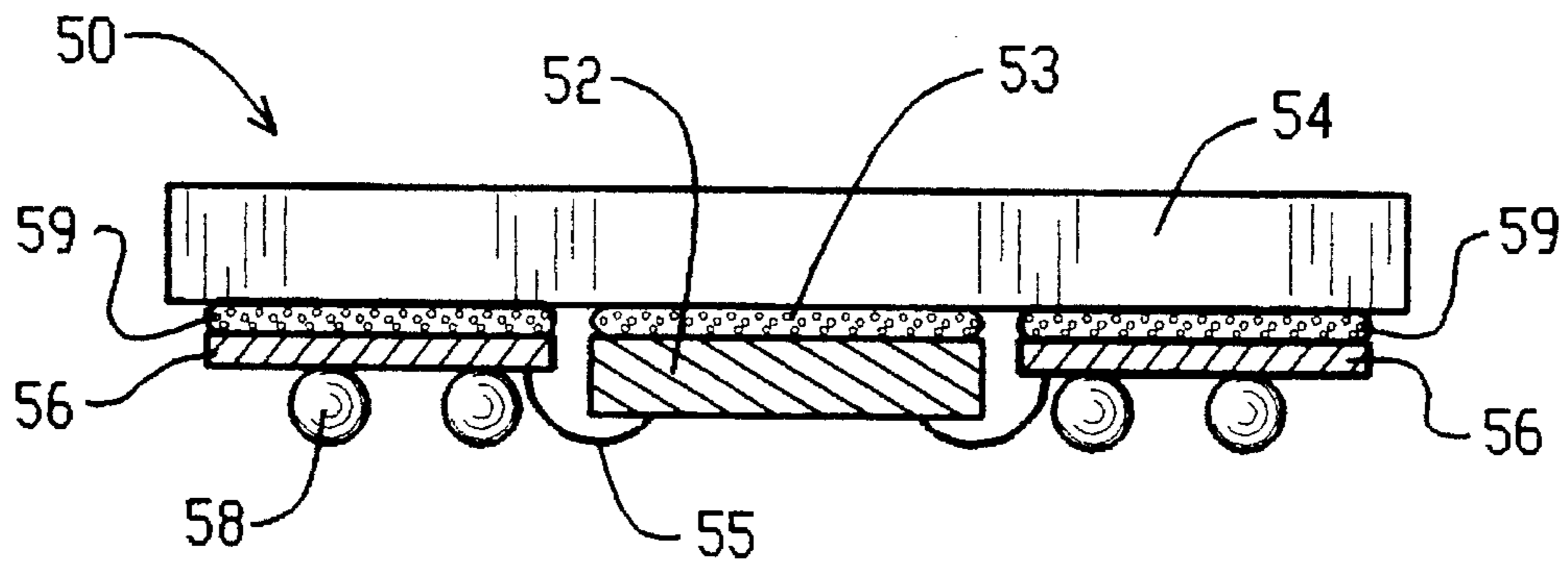
FIG. 7
