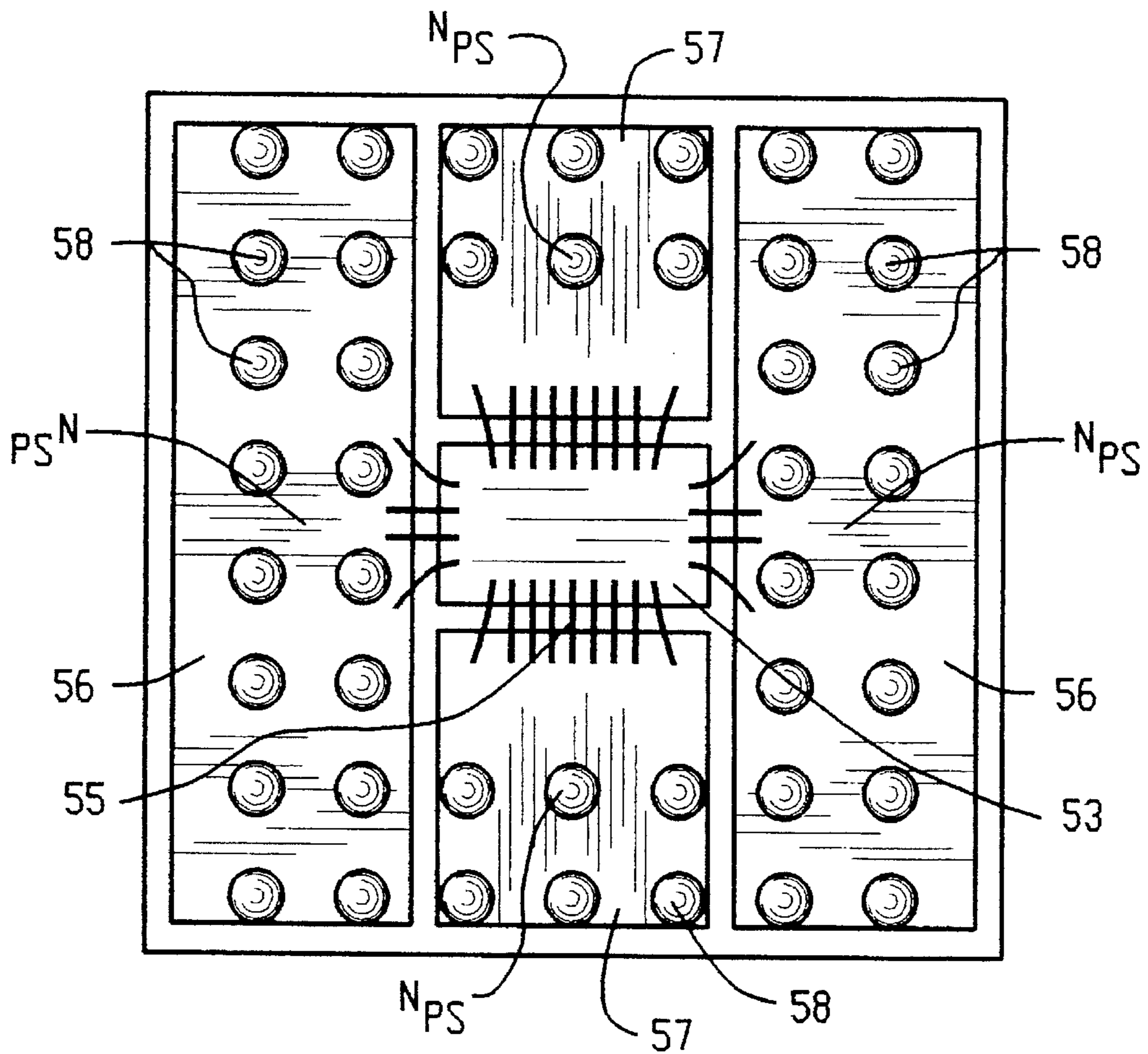
FIG. 8
